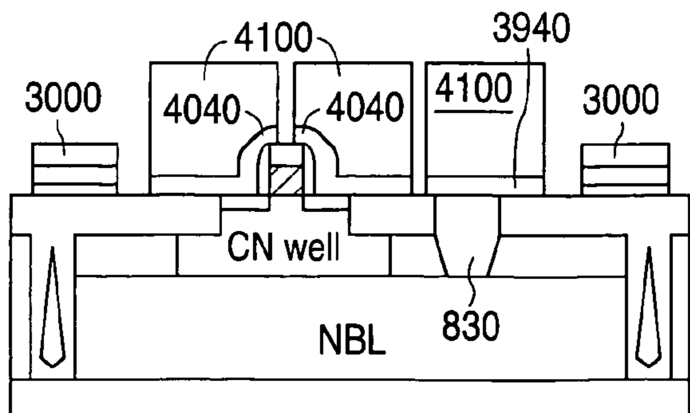
PMOS FIG. 41D
