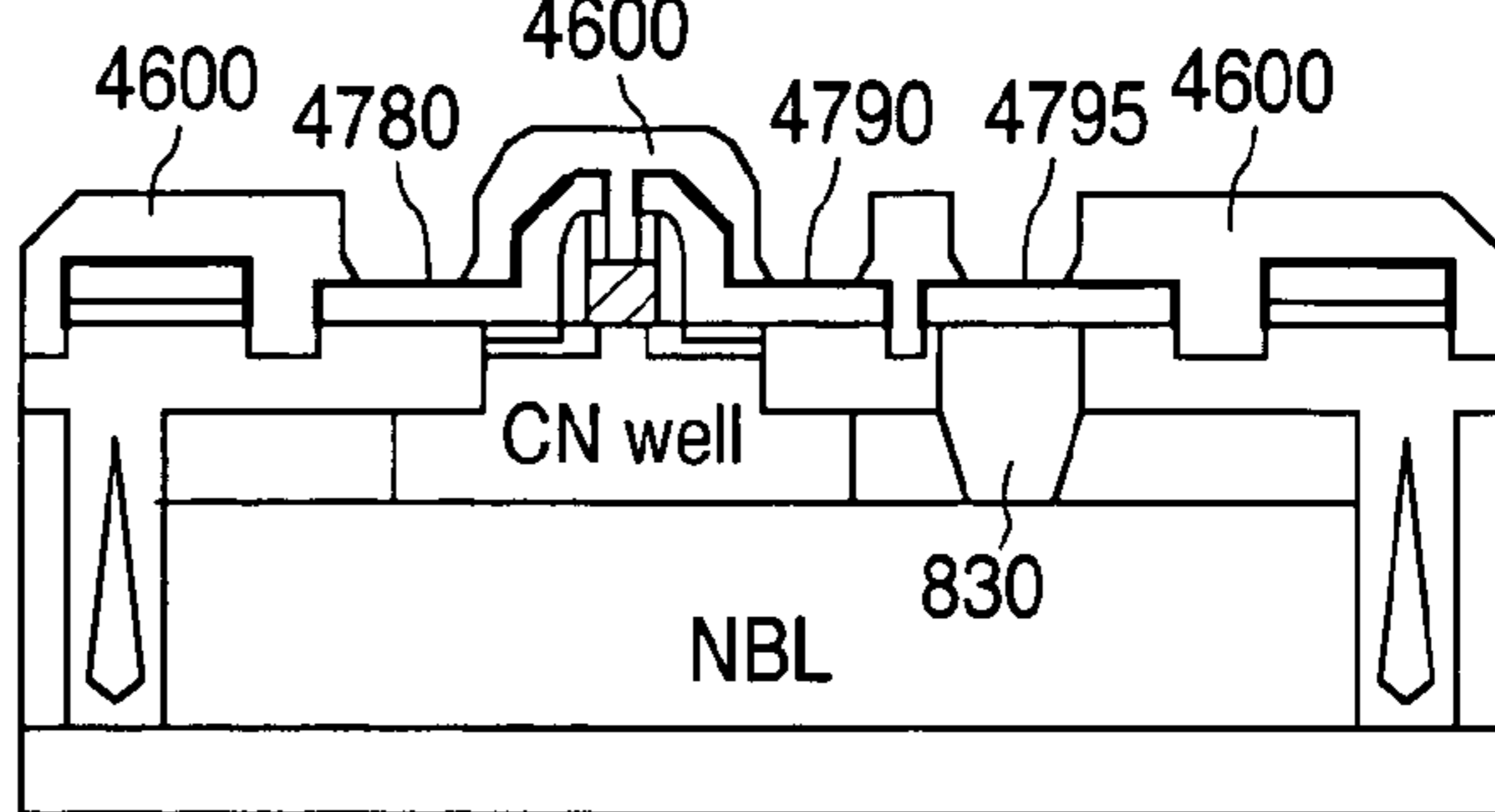
PMOS
