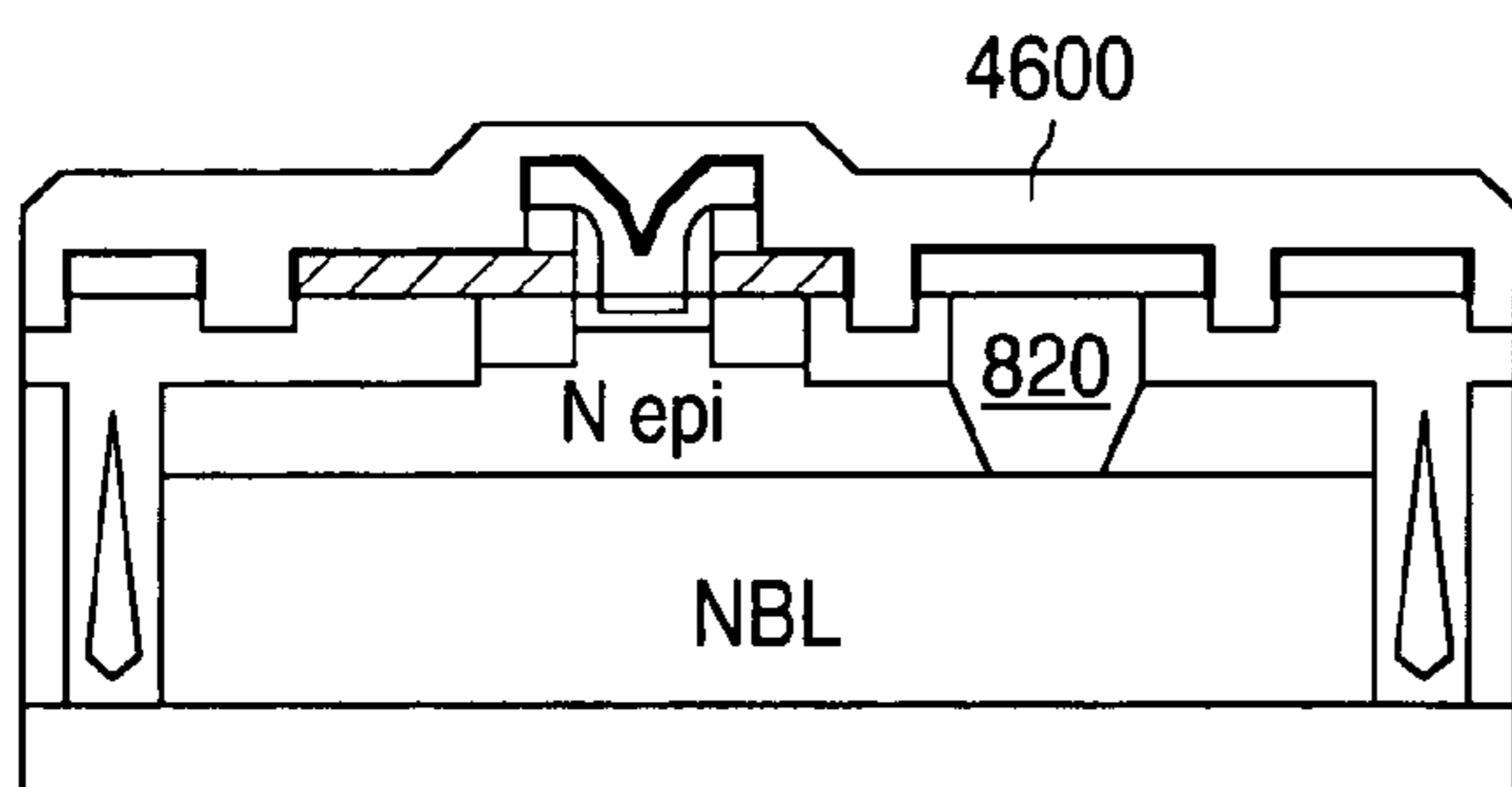
NPN FIG. 46A
