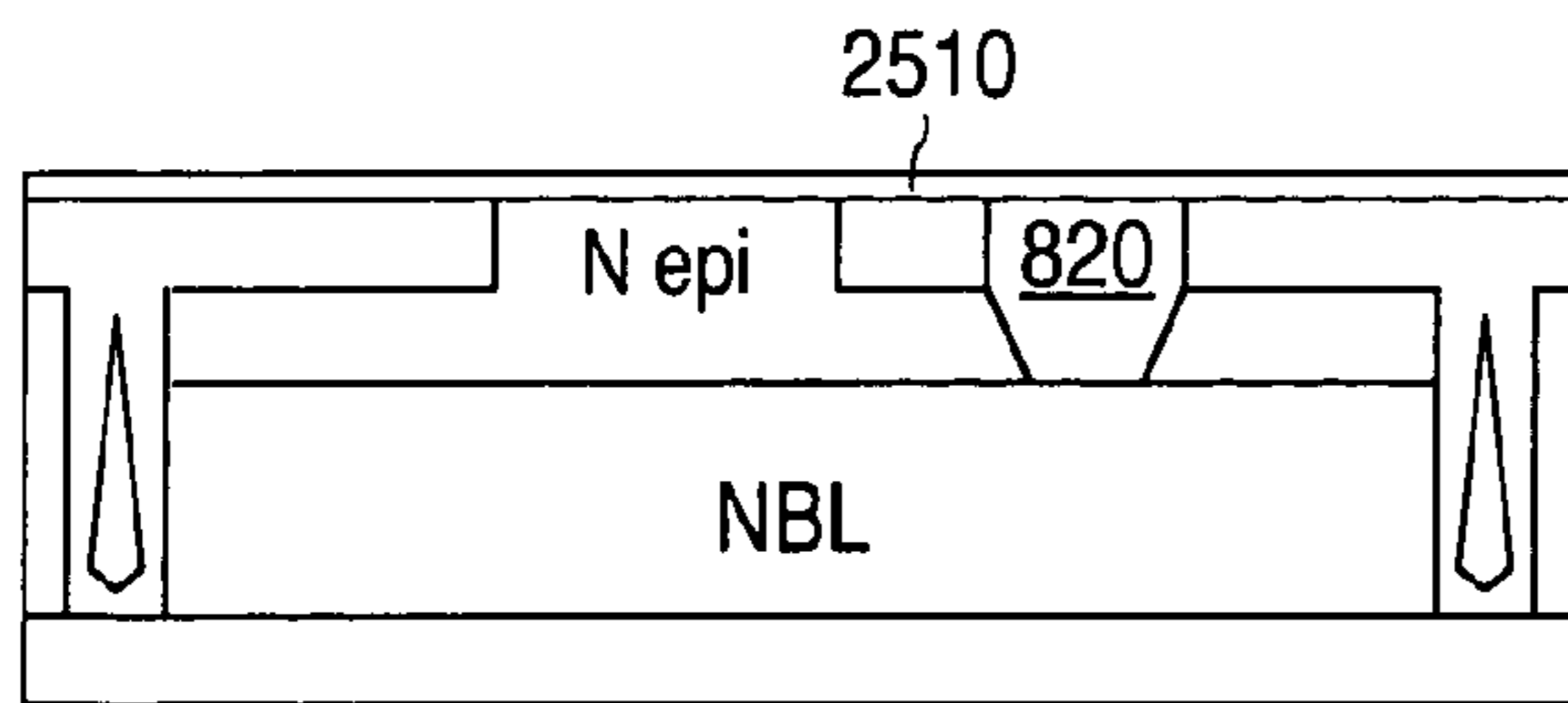
NPN FIG. 25A
