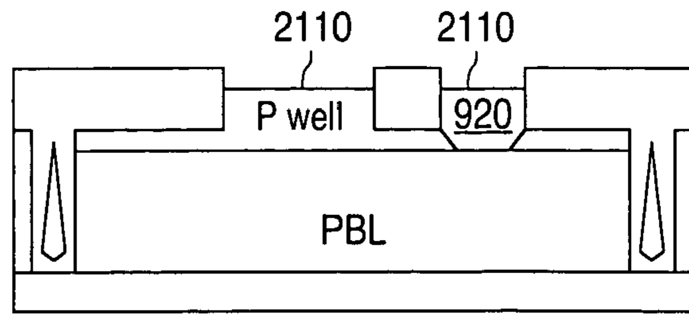
PNP FIG. 21B
