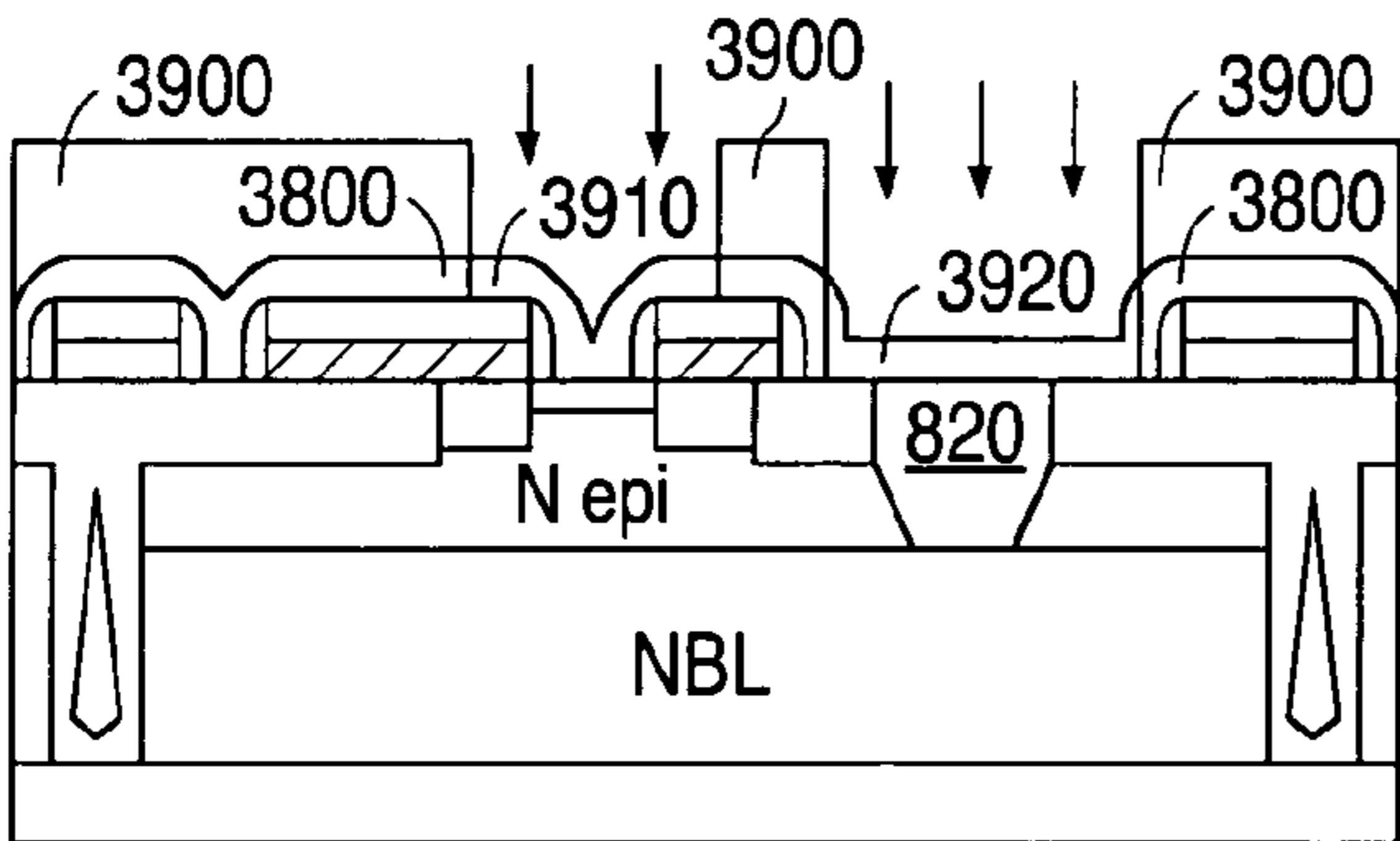
NPN FIG. 39A
