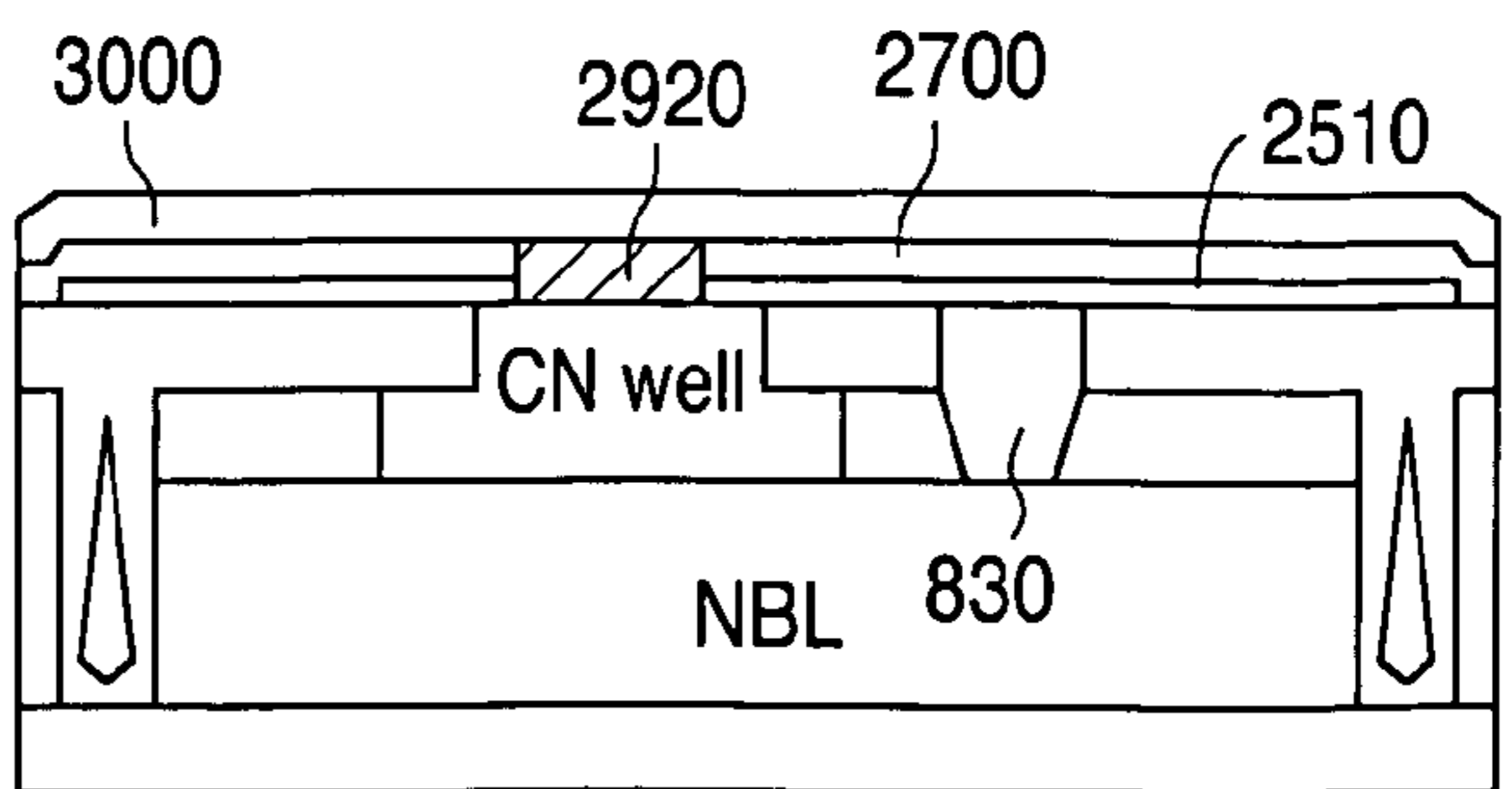
PMOS FIG. 30D
