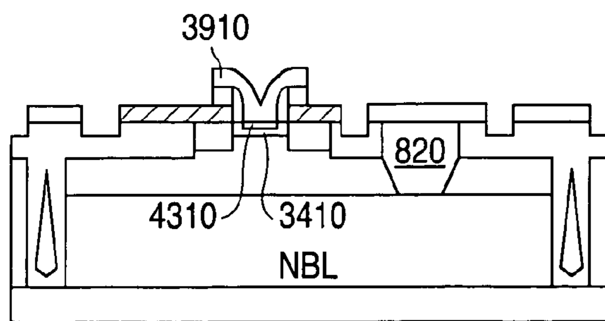
NPN
