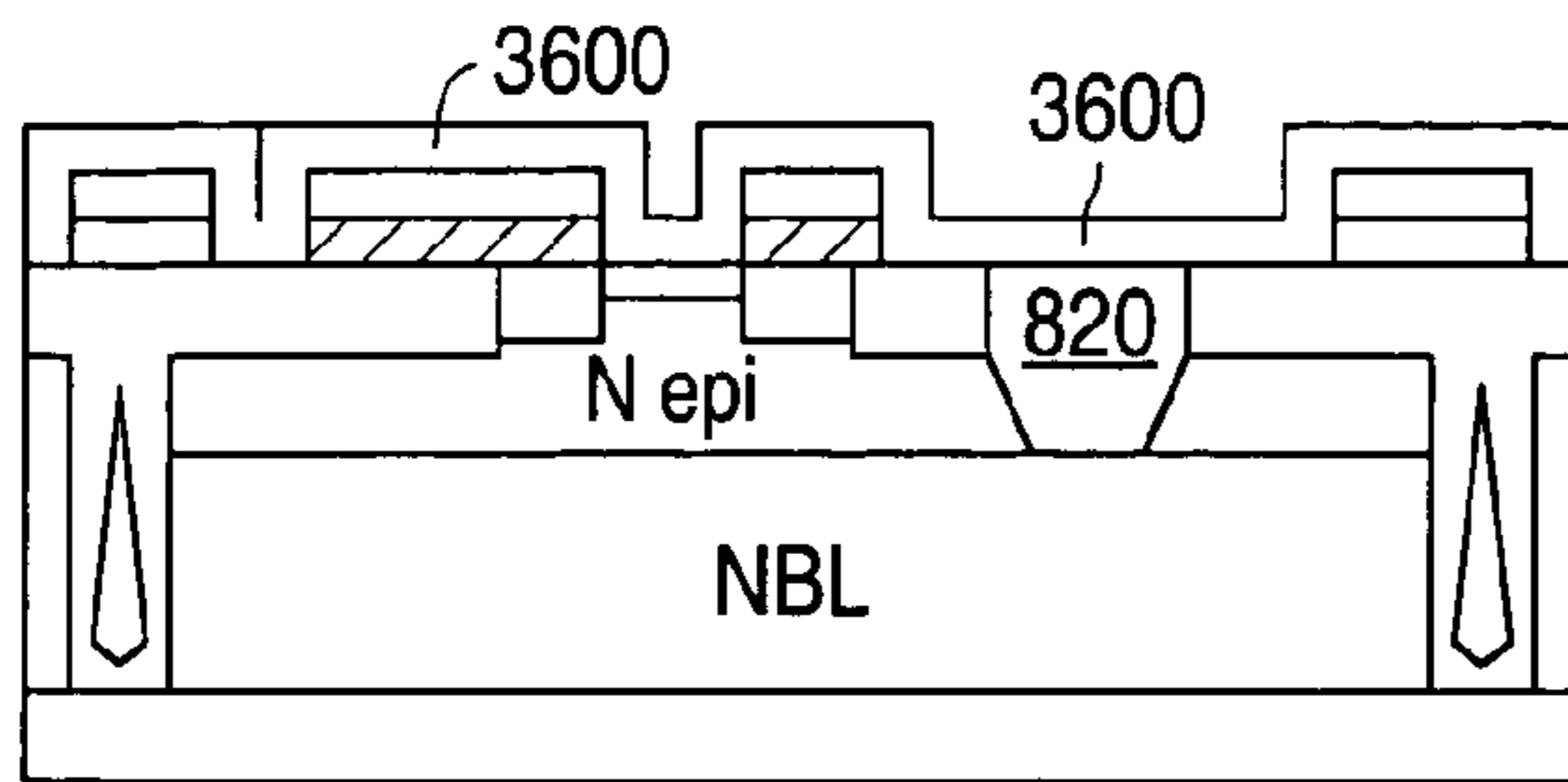
NPN FIG. 36A
