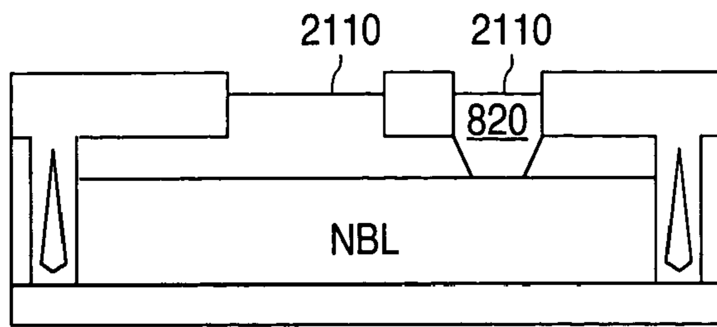
NPN FIG. 21A
