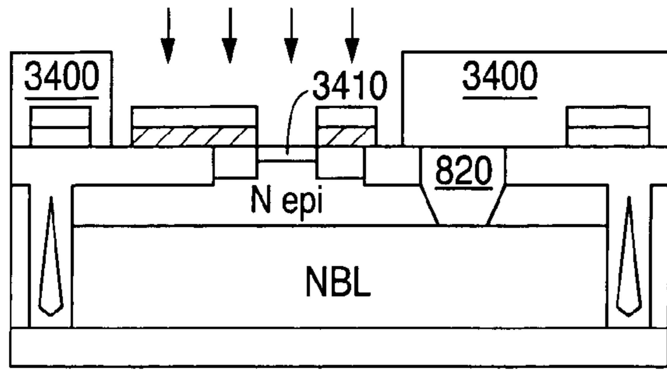
NPN FIG. 34A
