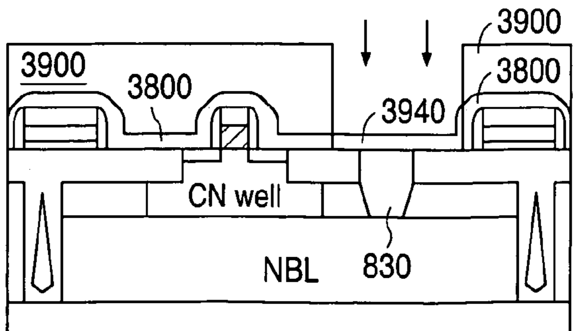
PMOS FIG. 39D
