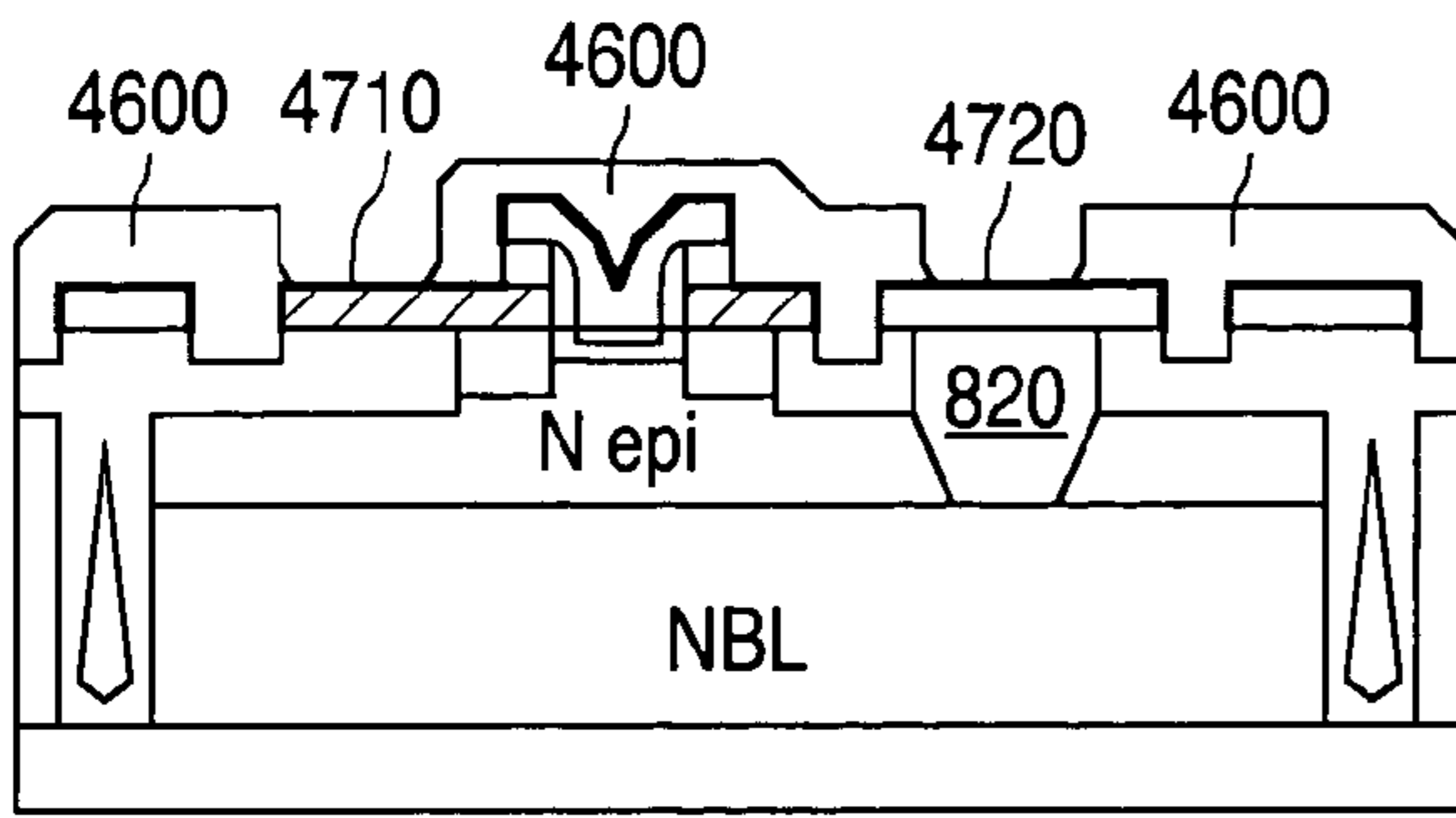
NPN
