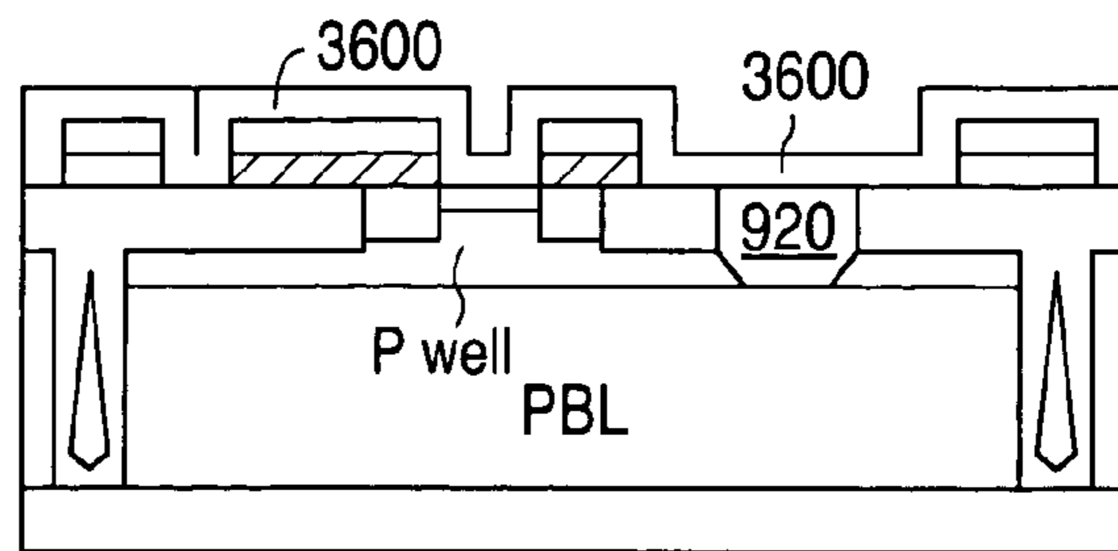
PNP FIG. 36B
