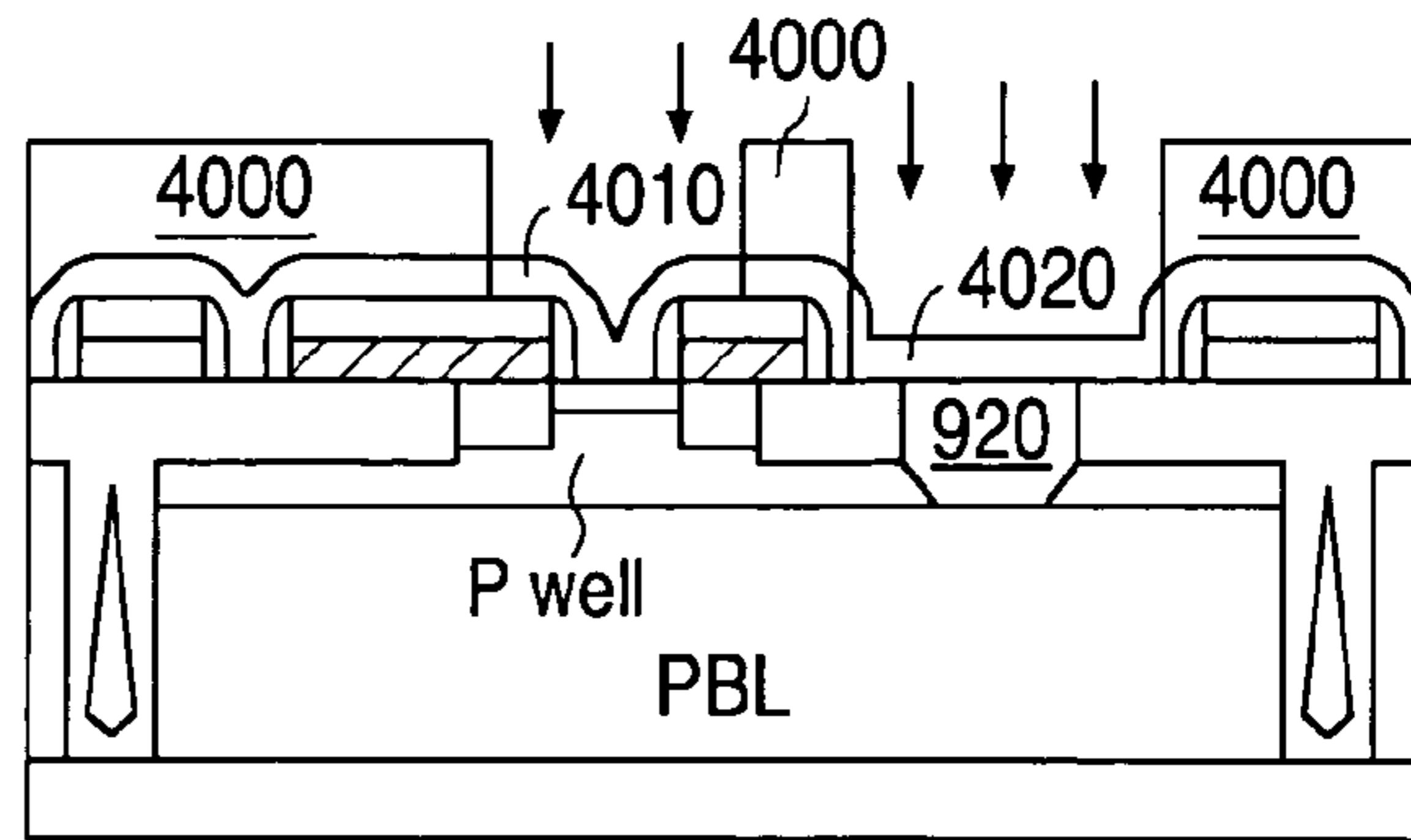
PNP FIG. 40B
