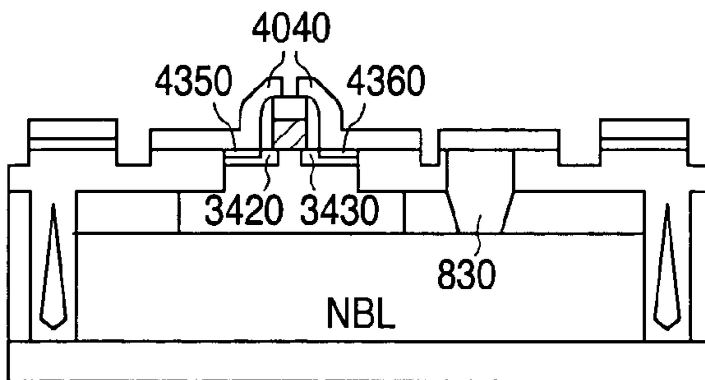
PMOS
