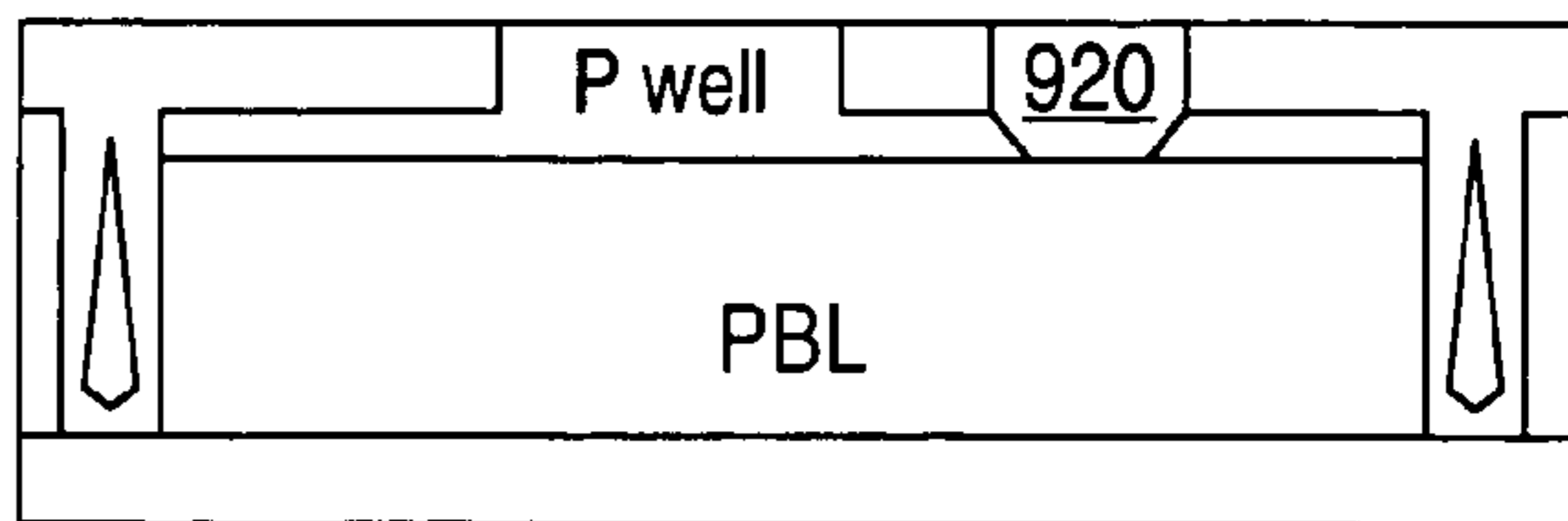
PNP FIG. 26B
