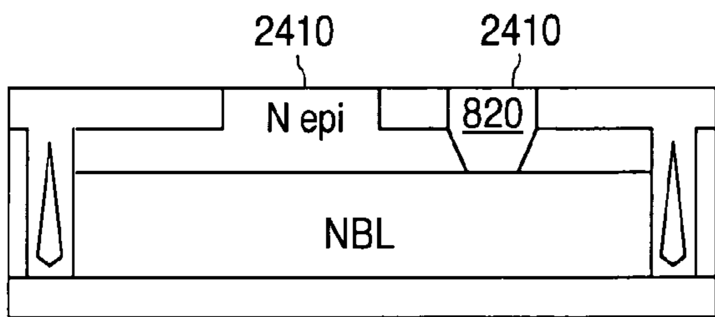
NPN
