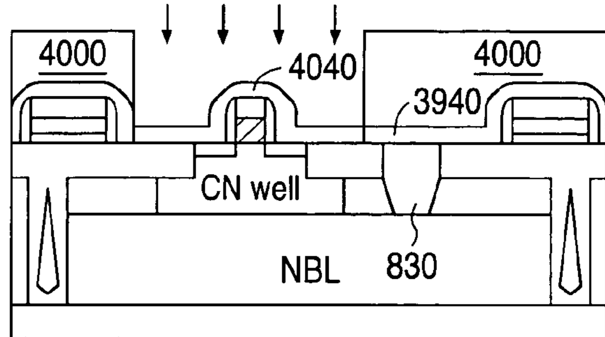
PMOS FIG. 40D
