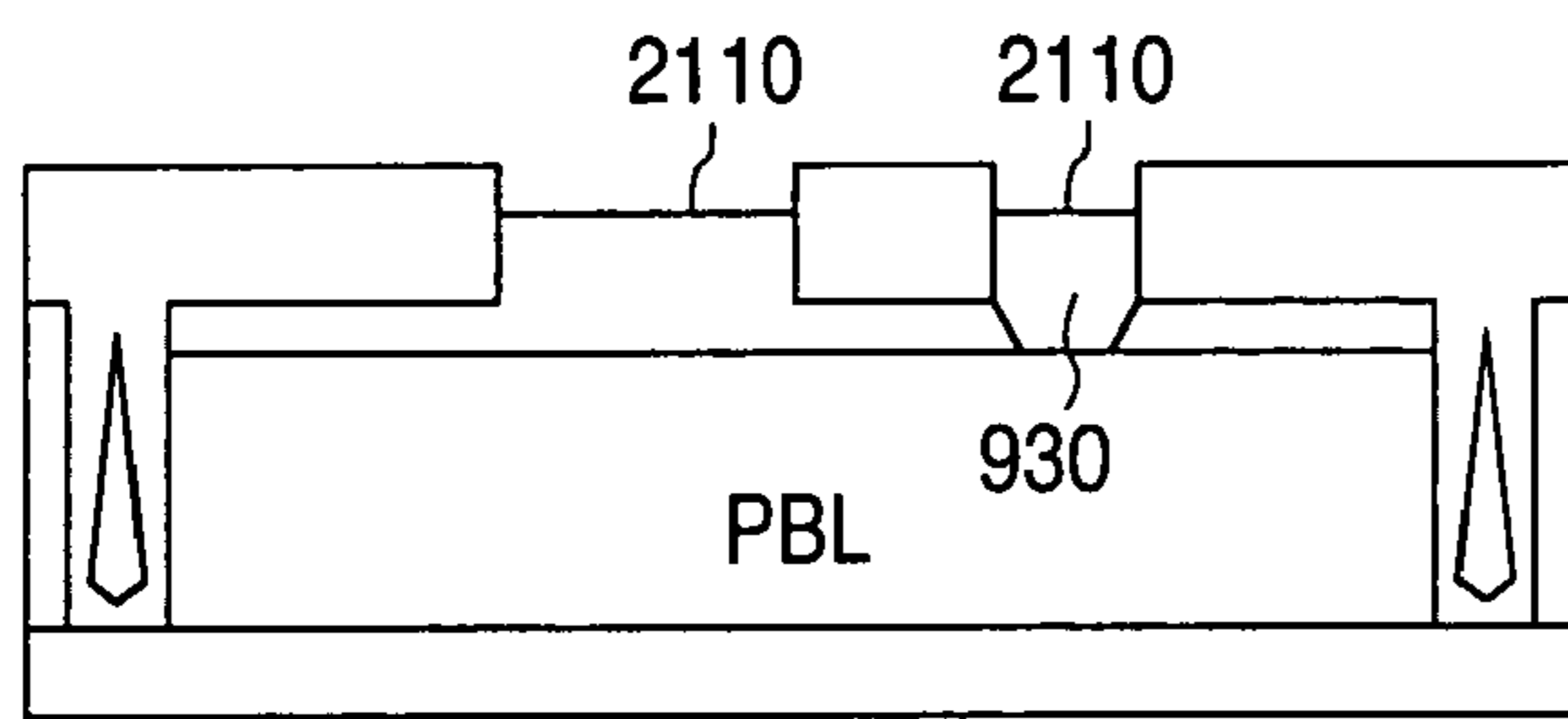
NMOS FIG. 21C
