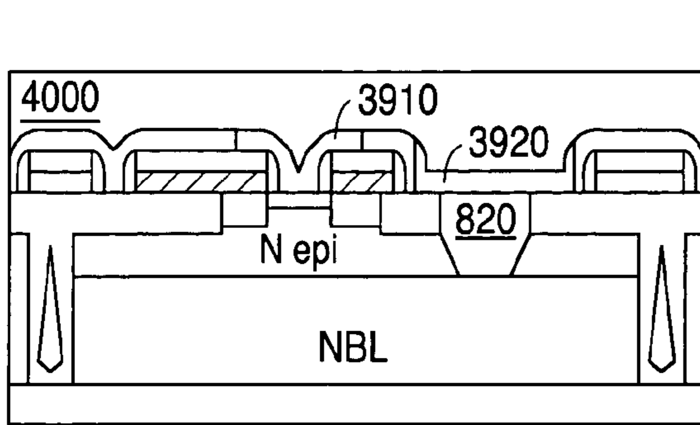
NPN FIG. 40A
