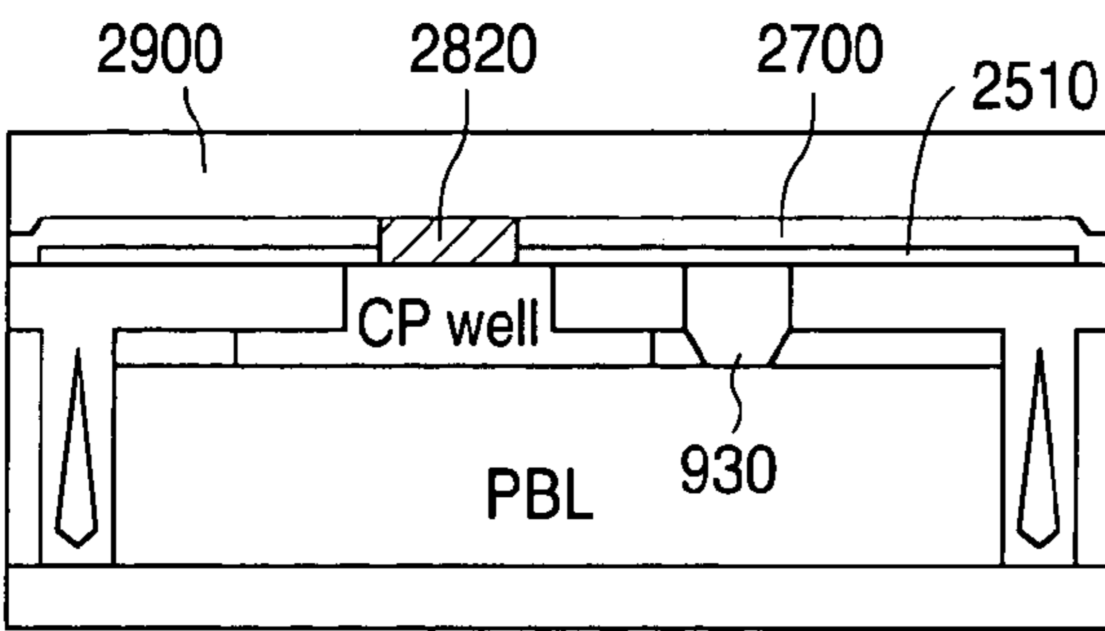
NMOS FIG. 29C
