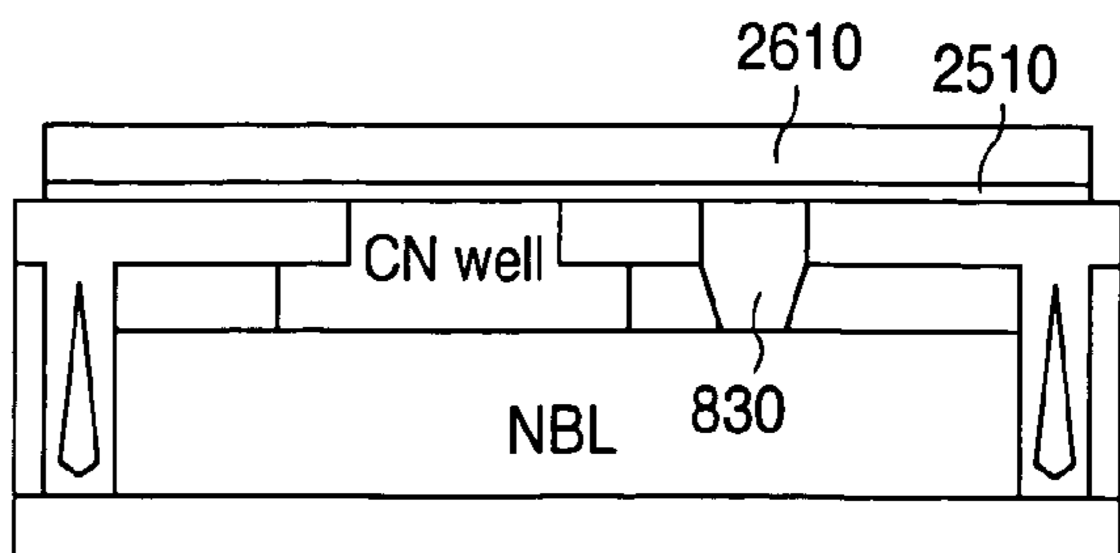
PMOS FIG. 26D
