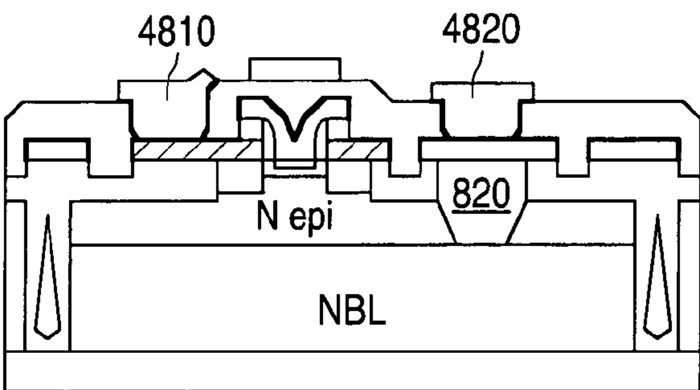
NPN
