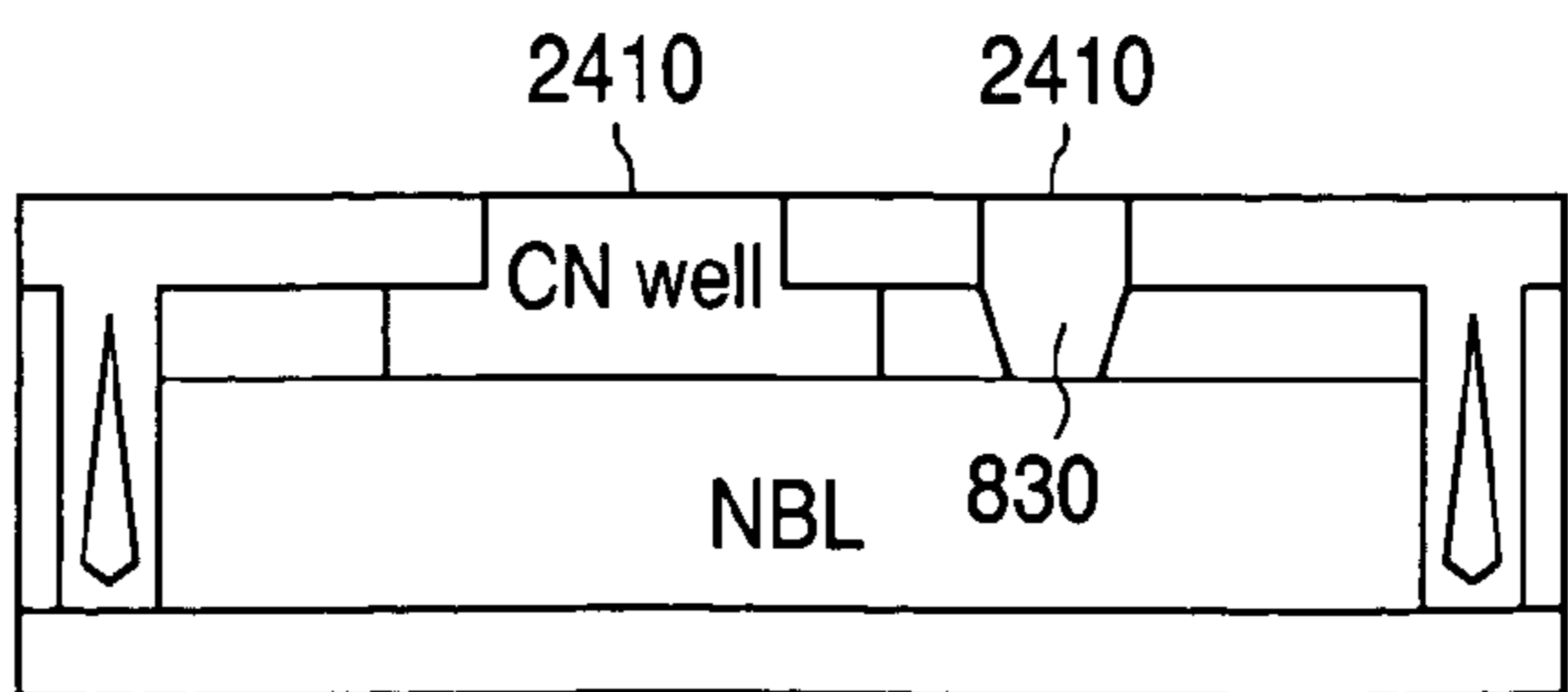
PMOS
