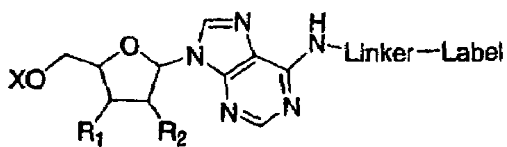
Adenosine N6-linker
