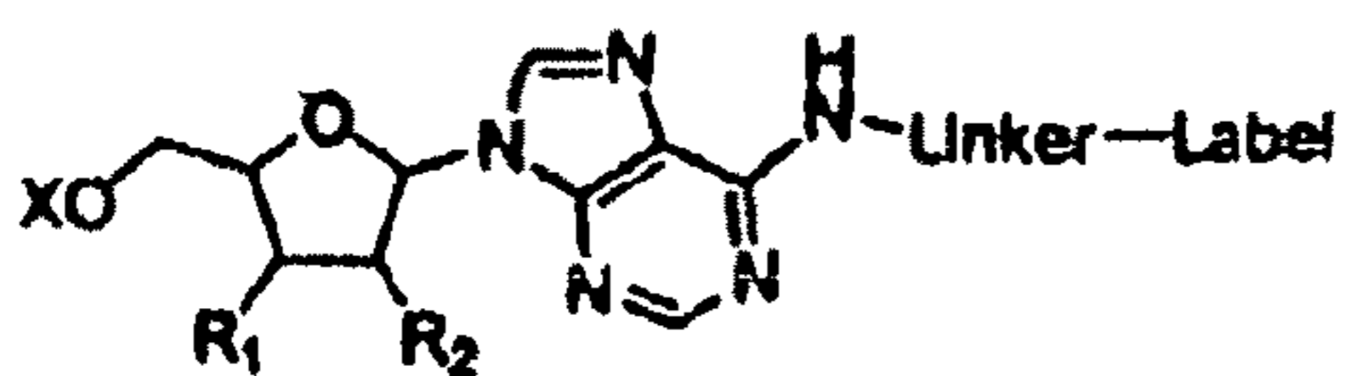
Adenosine N6-linker
