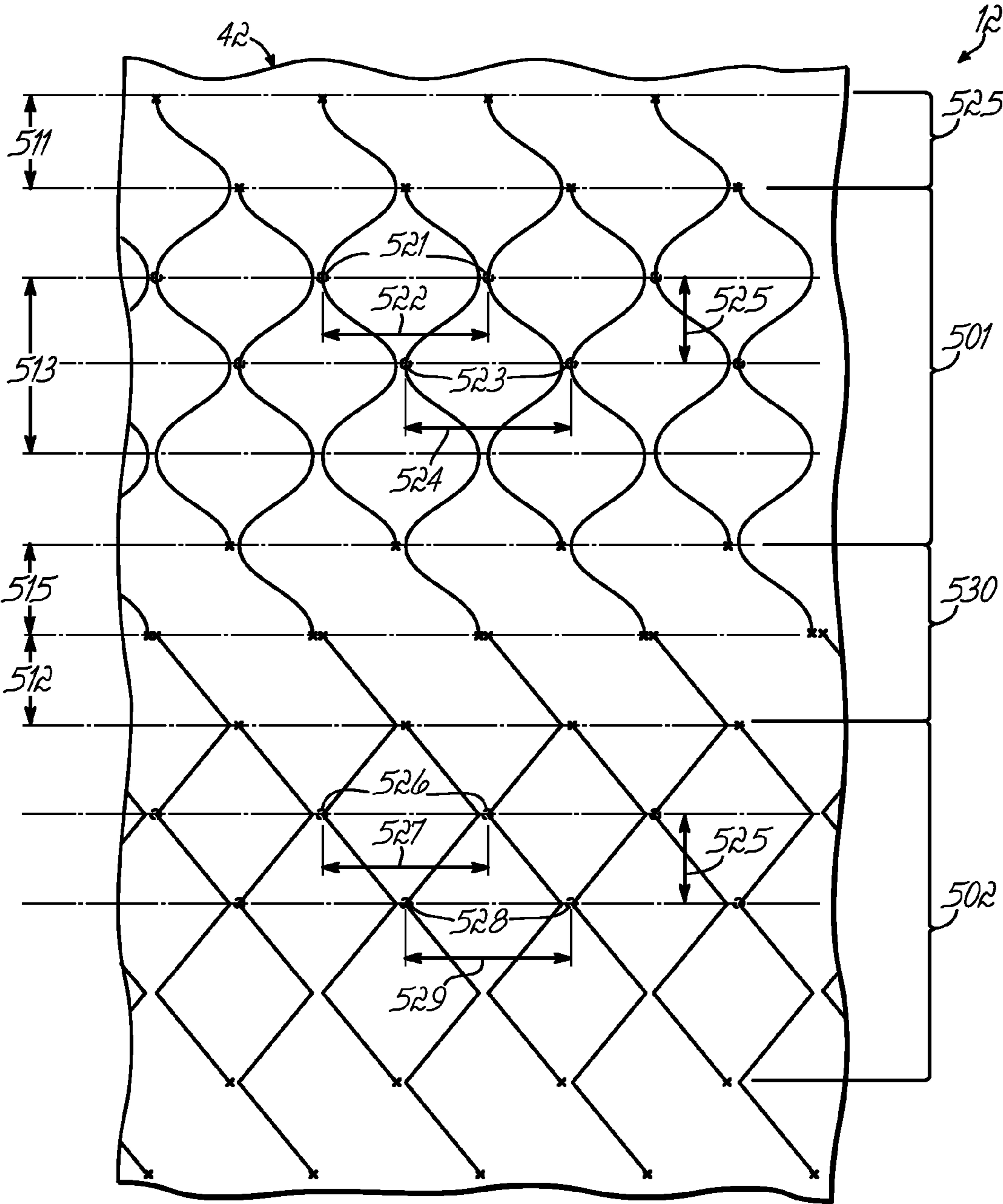
PRIOR ART FIG. 9A
