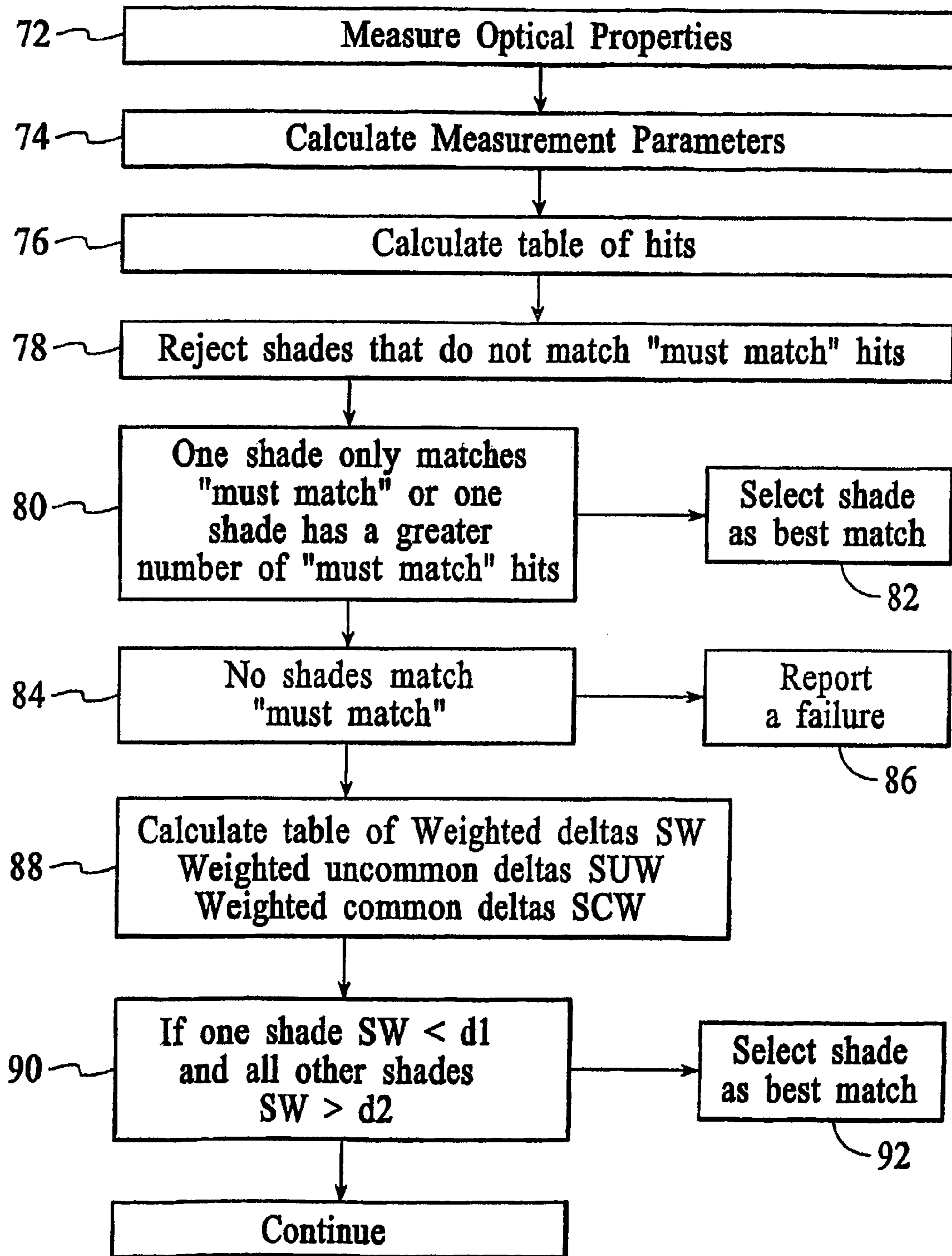
FIG. 11/1
