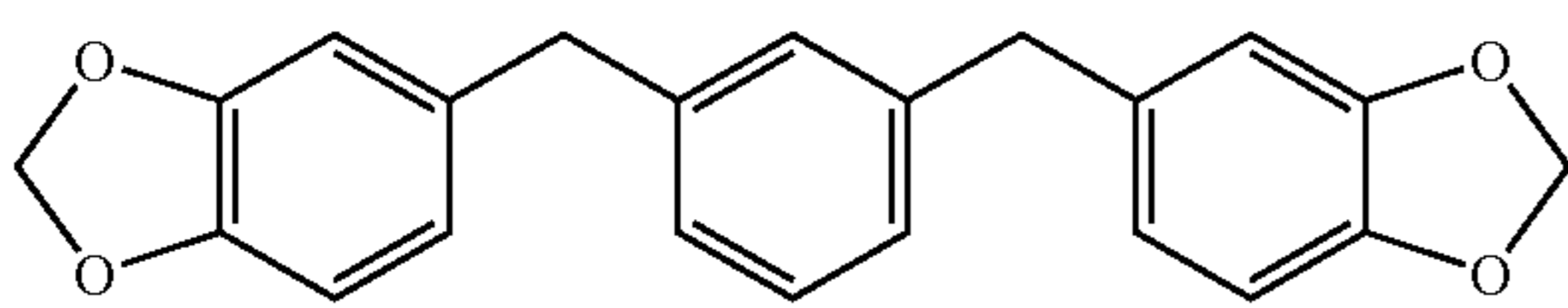
1,3-bis(3,4-methylenedioxybenzyl)benzene
