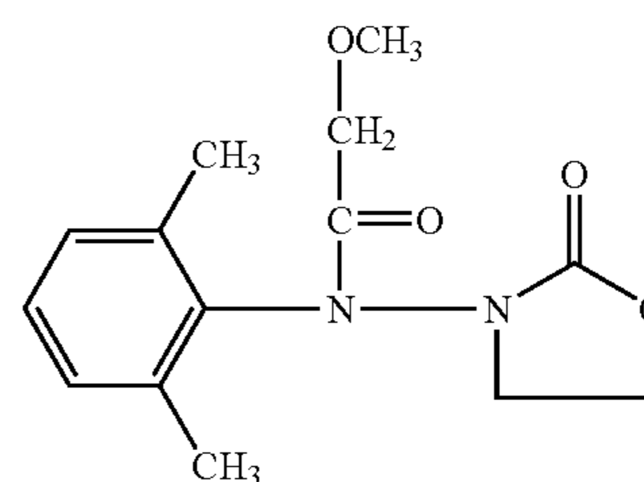
(OXADIXYL)
