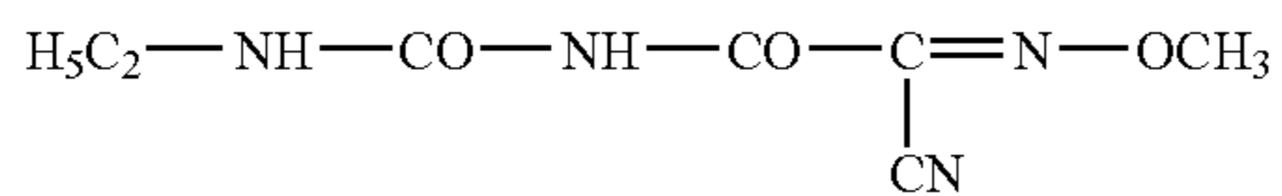
(CYMOXANIL)
