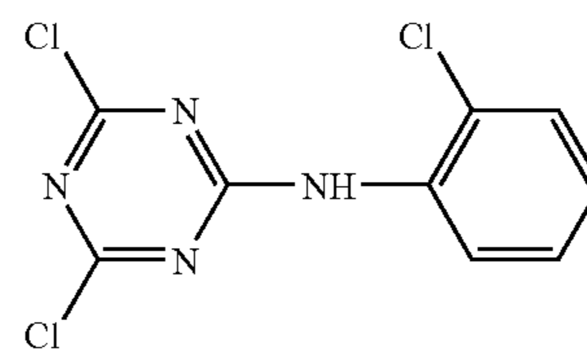
(ANILAZIN)
