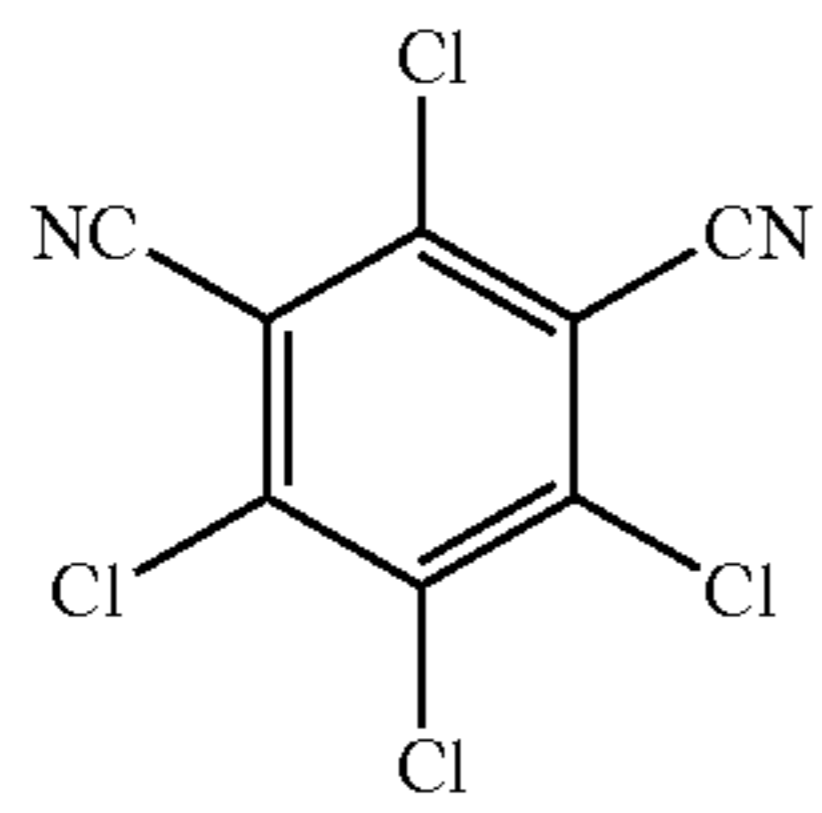
(CHLOROTHALONIL)
