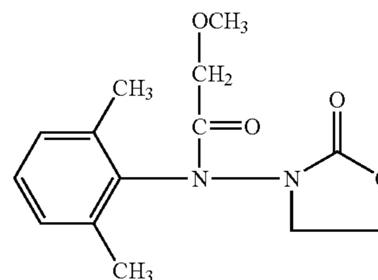
(OXADIXYL)
