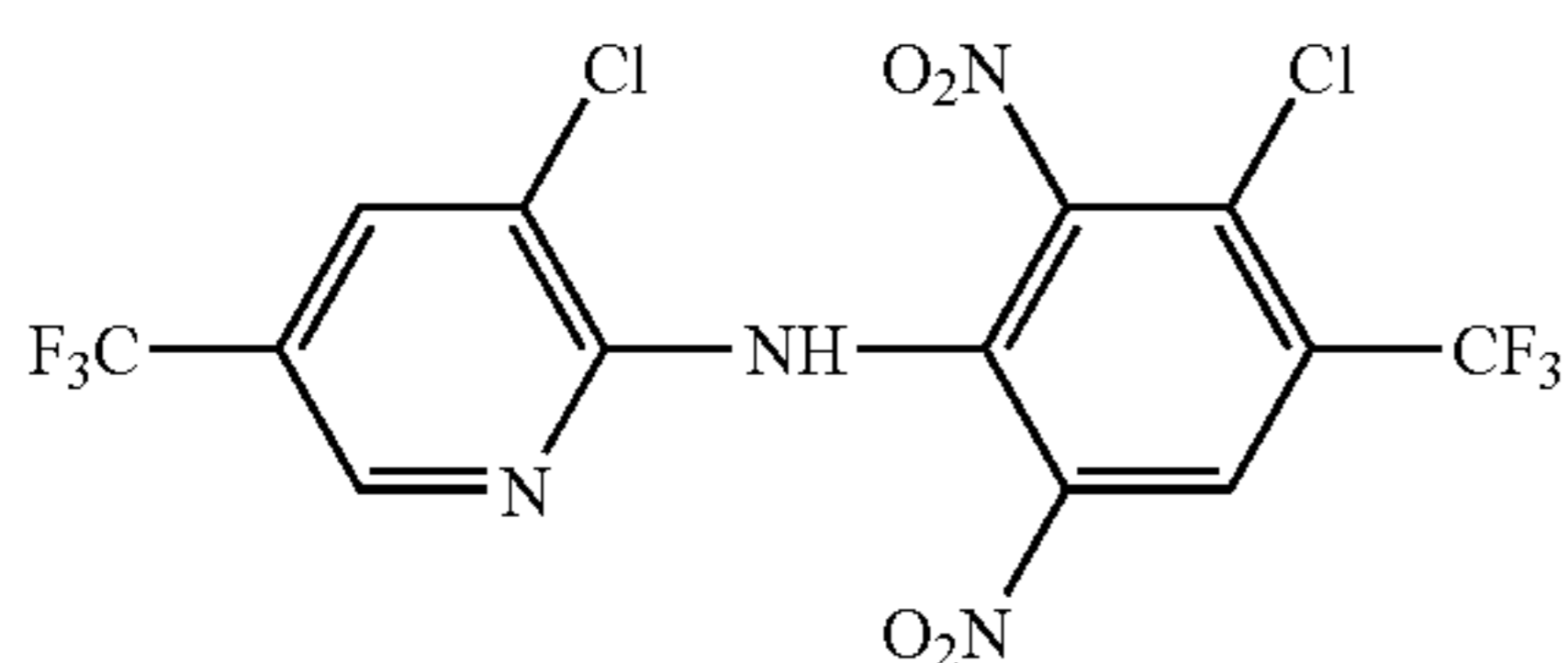
(FLUAZINAM)
