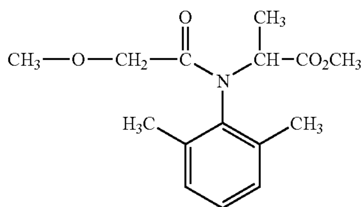
(METALAXYL)
