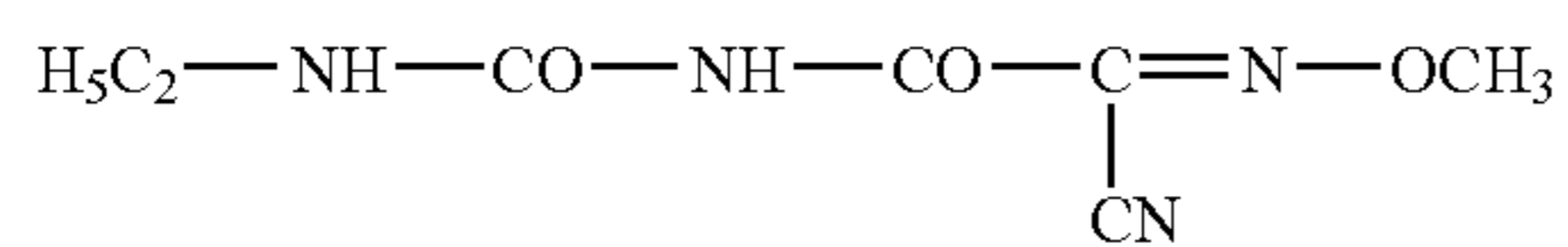
(CYMOXANIL)
