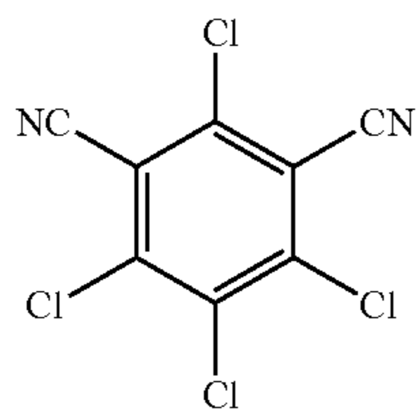
(CHLOROTHALONIL)
