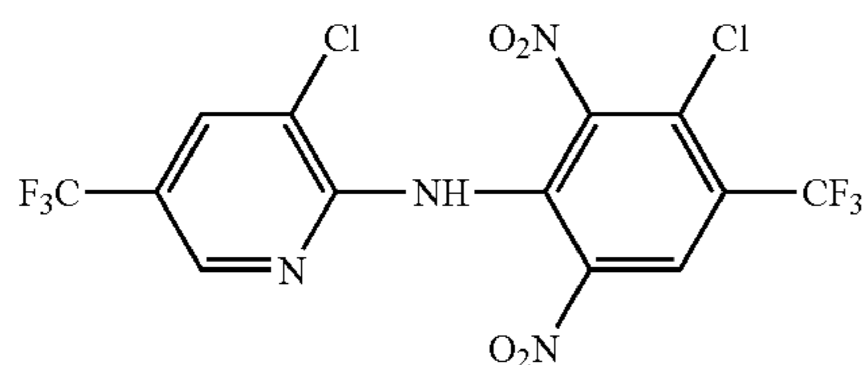
(FLUAZINAM)
