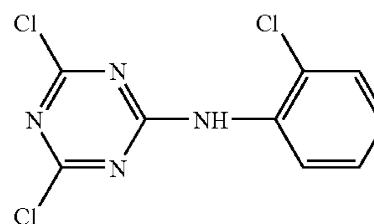
(ANILAZIN)
