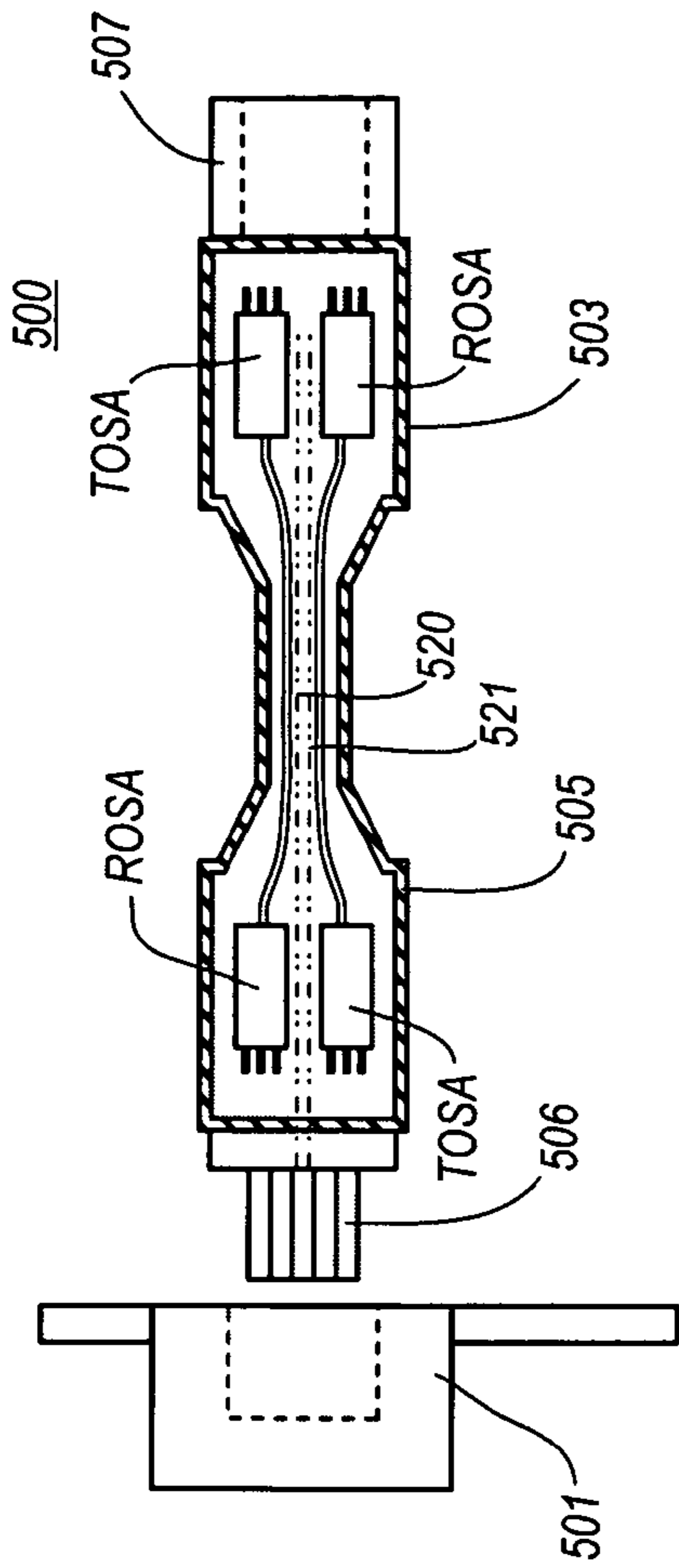
FIG. 5A
