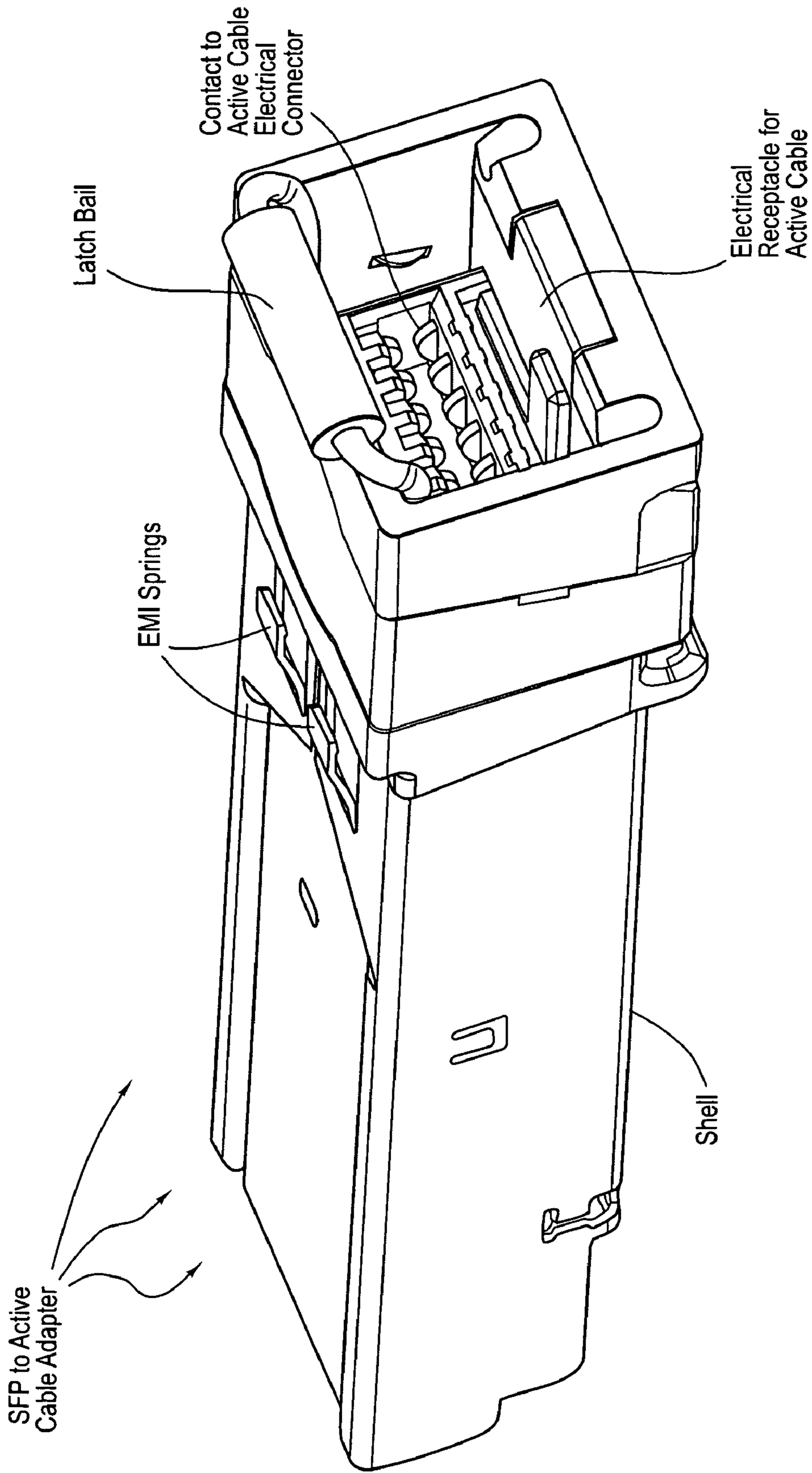
FIG. 20A
