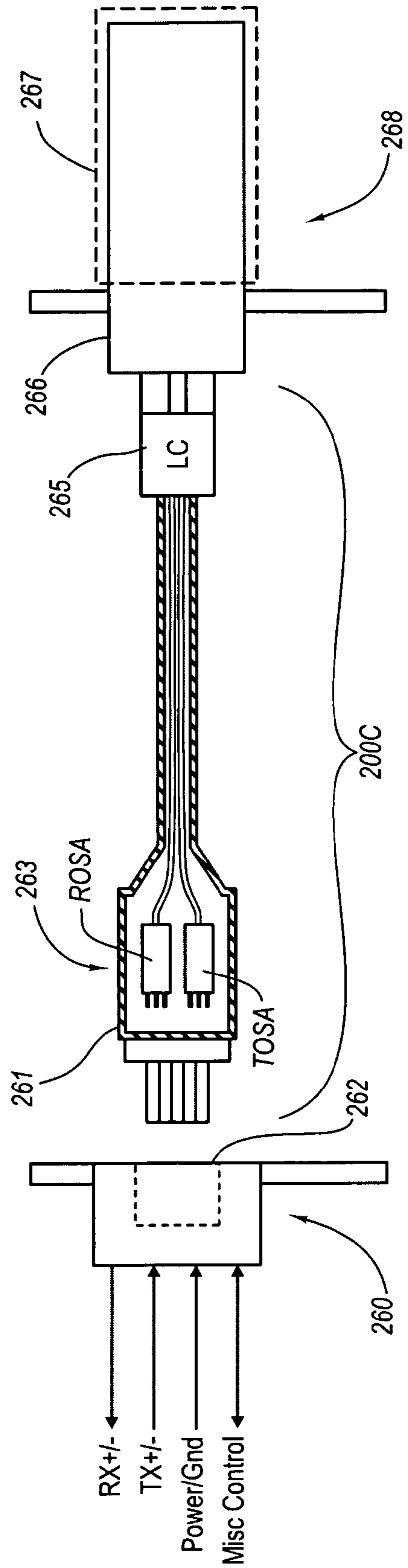
FIG. 2C
