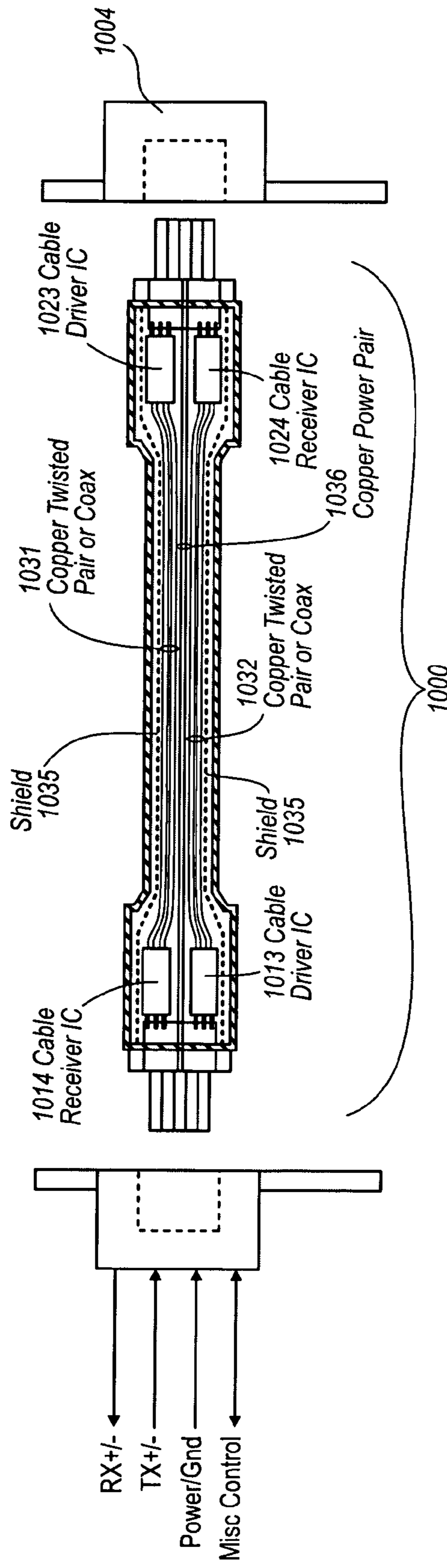
FIG. 10
