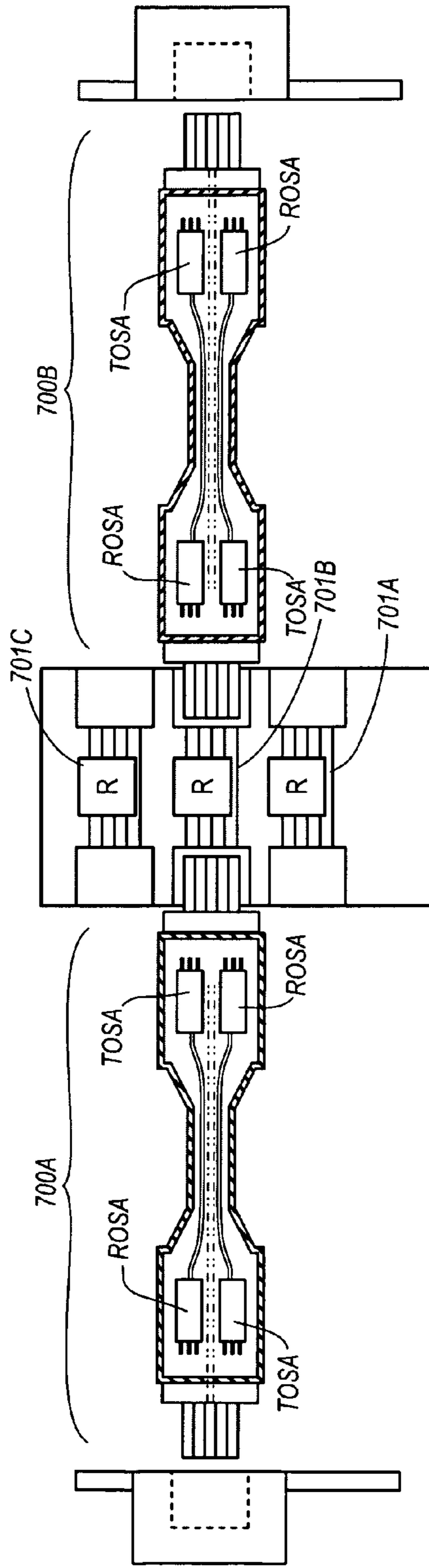
FIG. 6A
