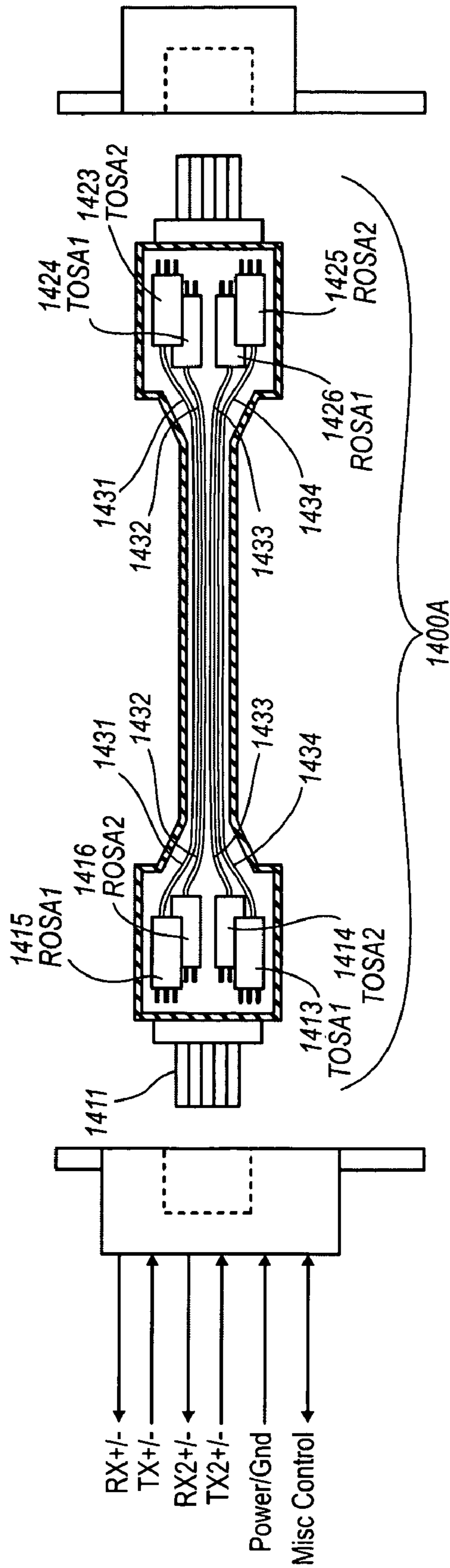
FIG. 14A
