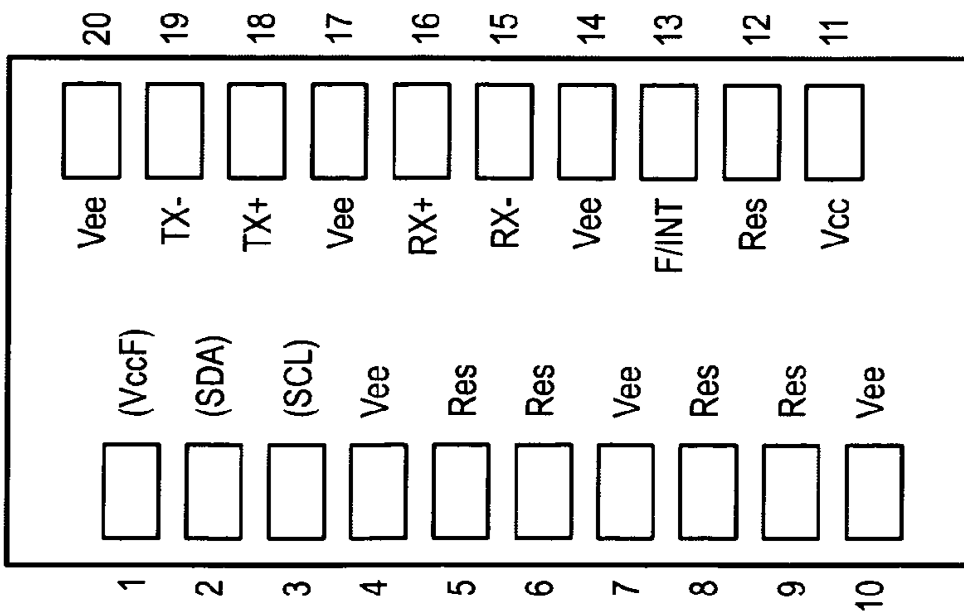
FIG. 15C
