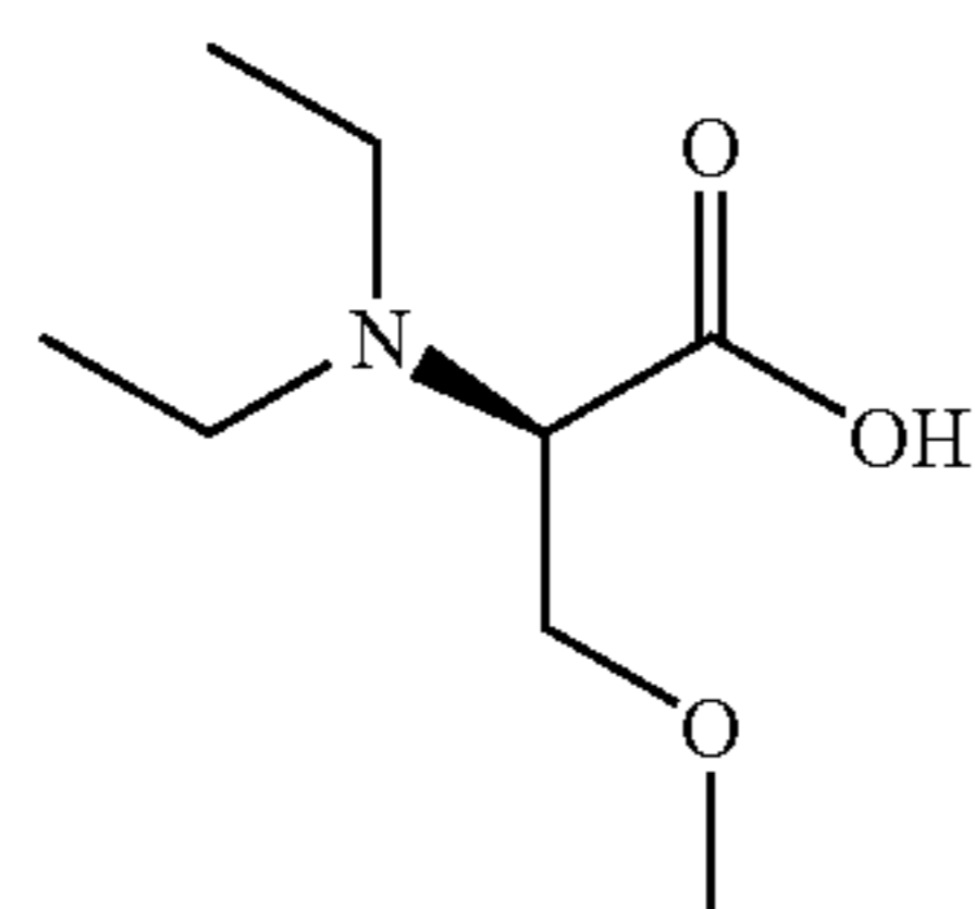
Cap-75, Step a
