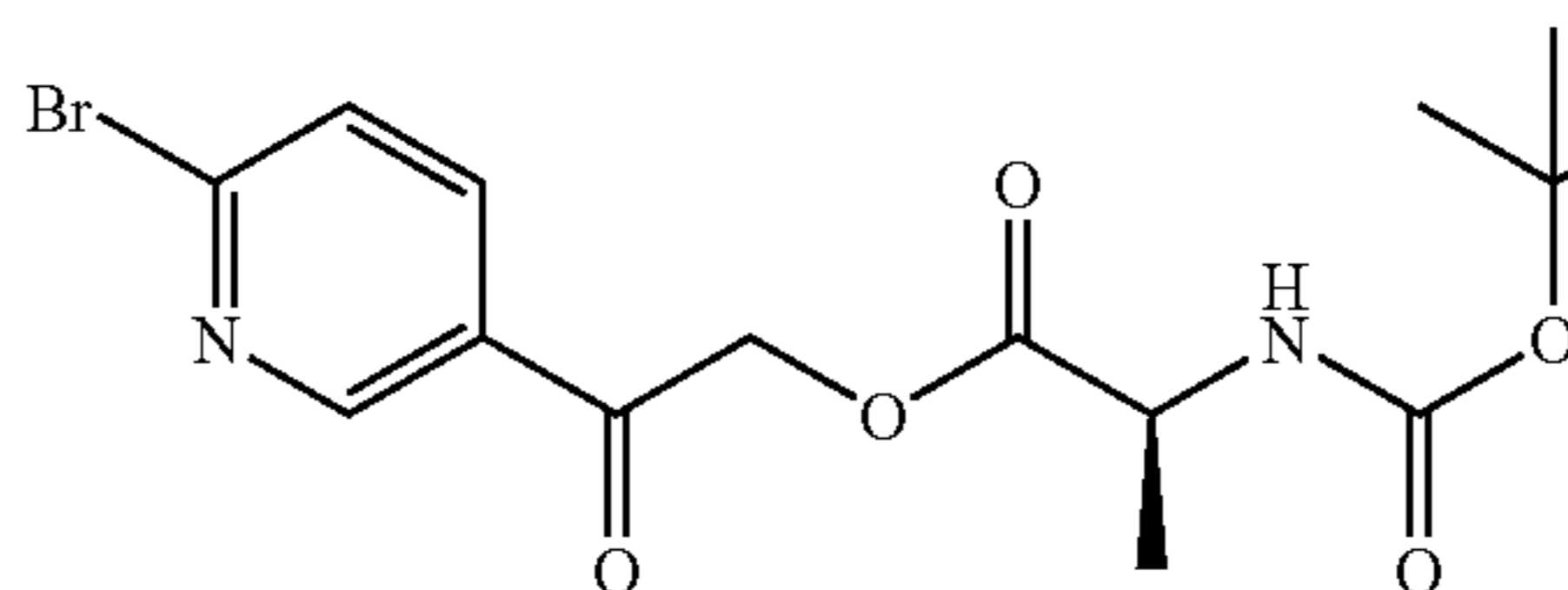
Example 152c-3
