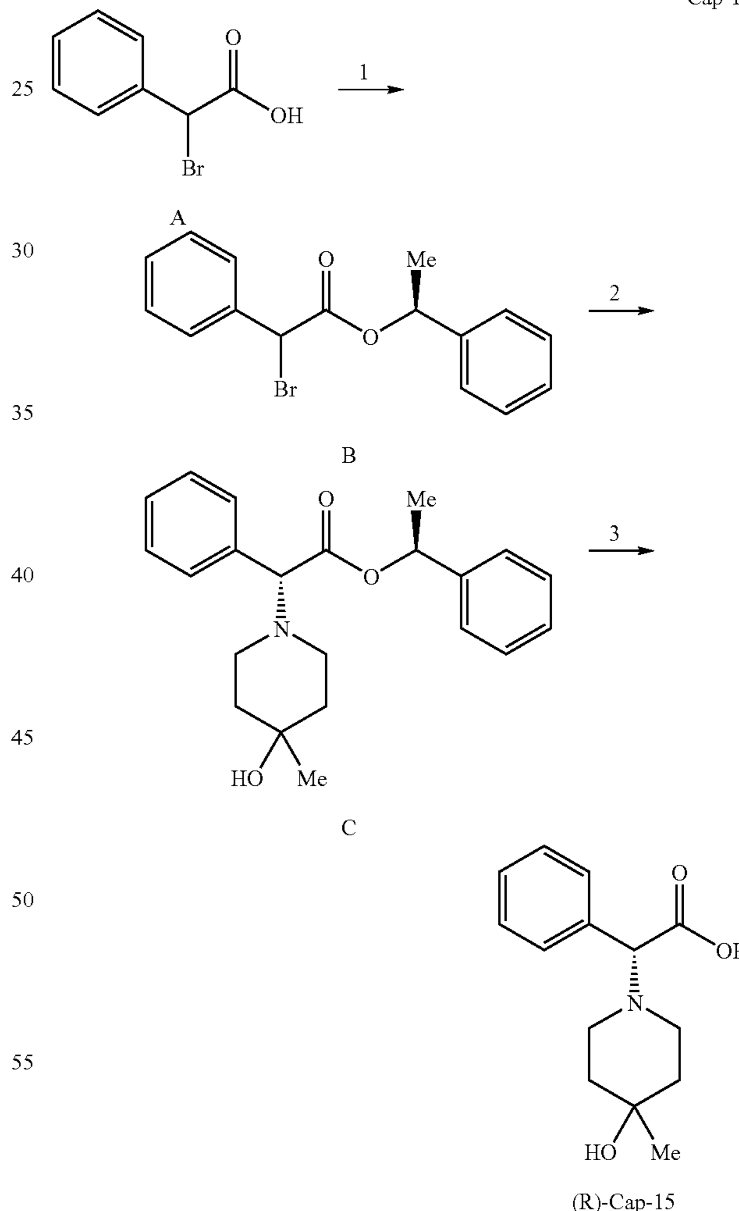
Cap-15
