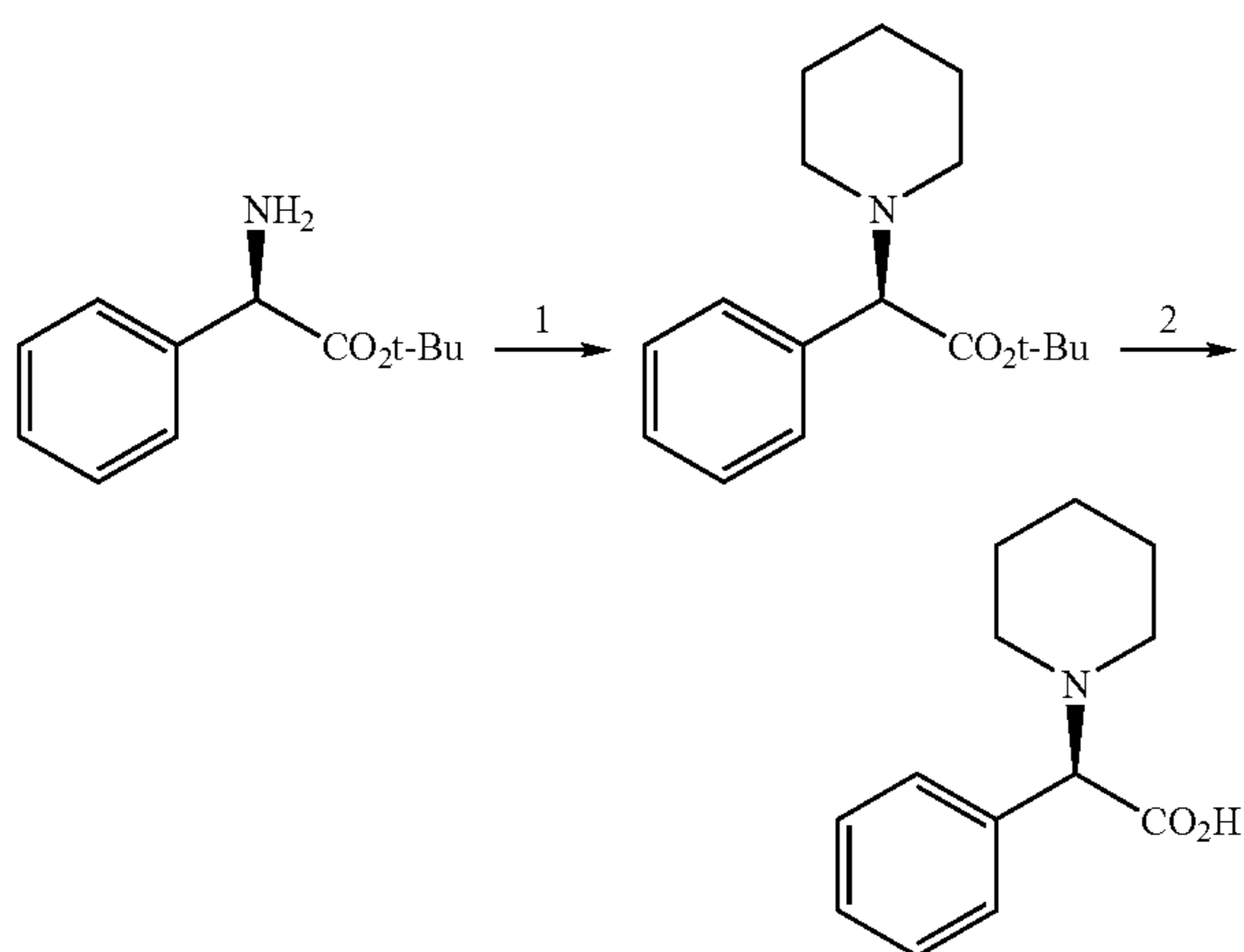
Cap-14
