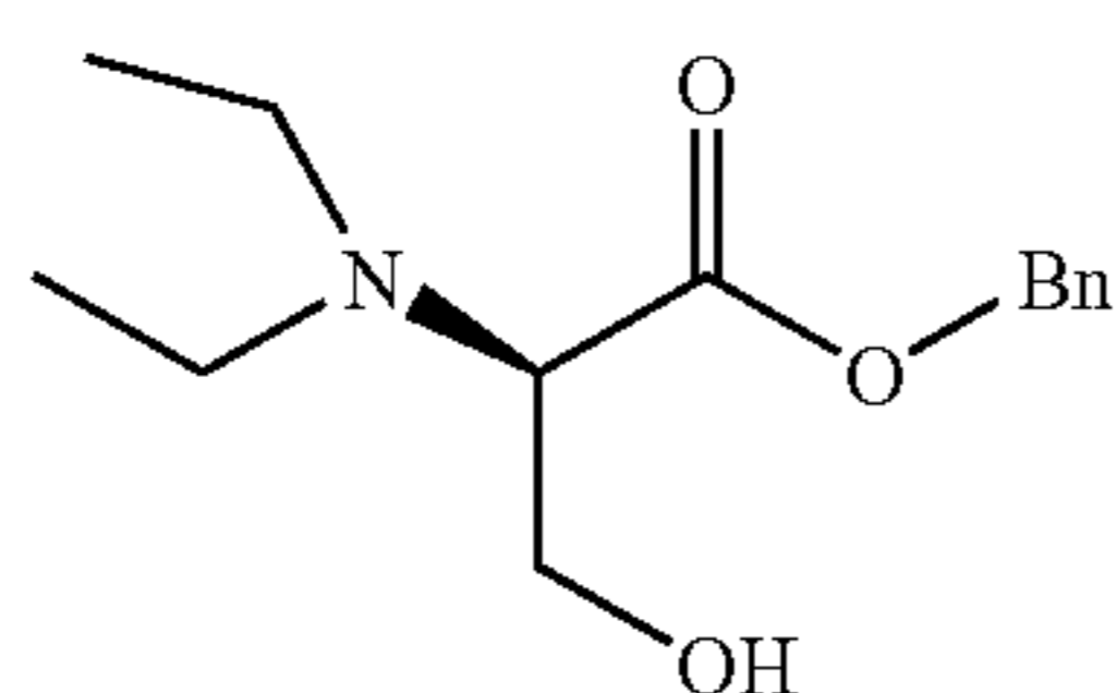
Cap-75, Step a
