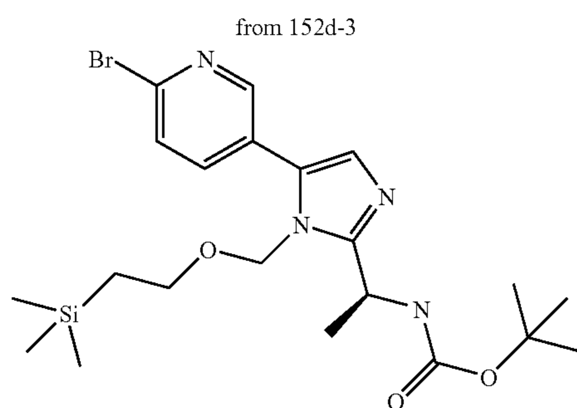
Example 152e-4
