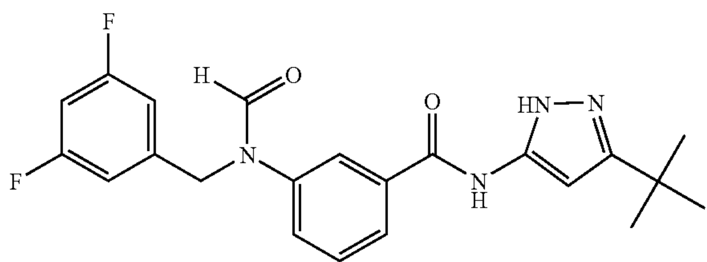
N-(5-tert-Butyl-2H-pyrazol-3-yl)-3-[(3,5-difluorophenyl)-formyl-amino]-benzamide
