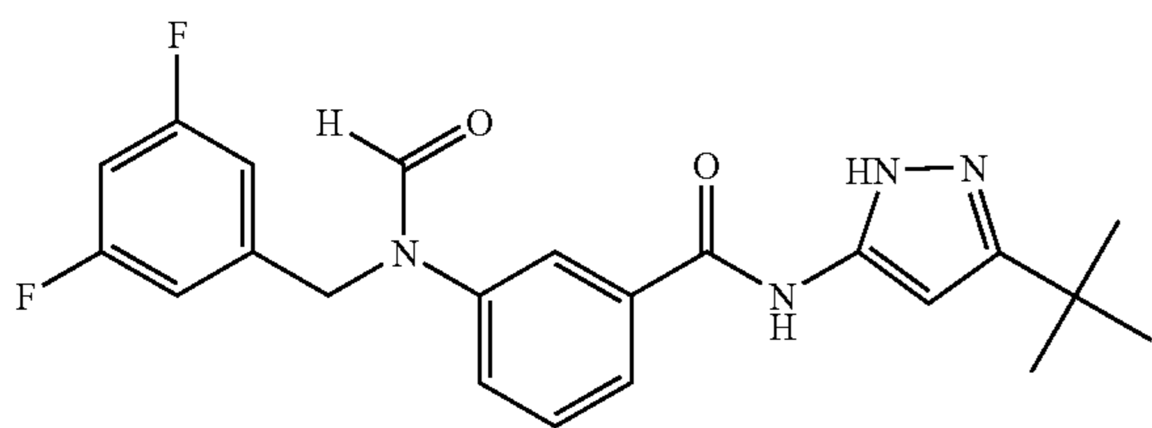
N-(5-tert-Butyl-2H-pyrazol-3-yl)-3-[(3,5-difluorophenyl)-formyl-amino]-benzamide
