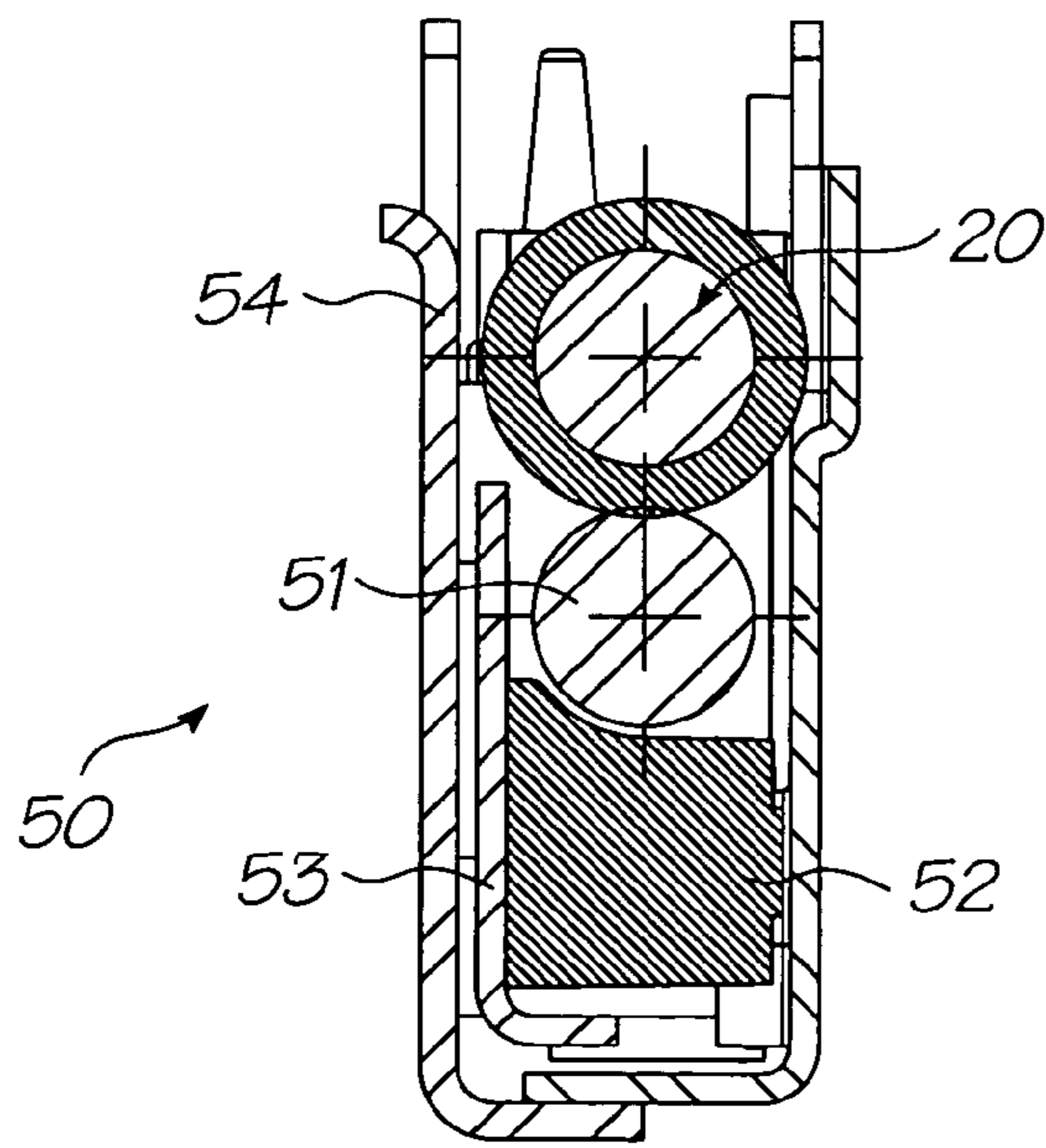
Section A-A
