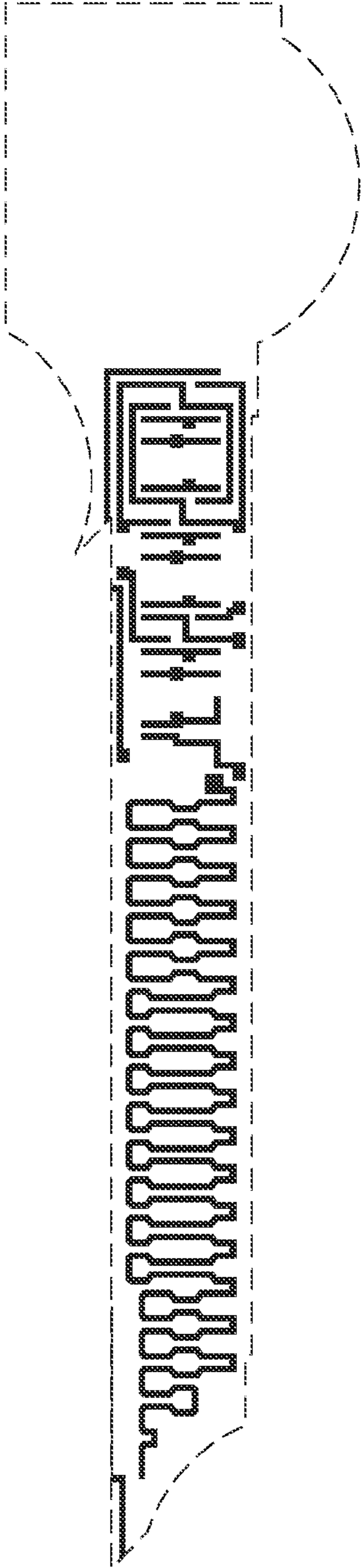
Poly mask
