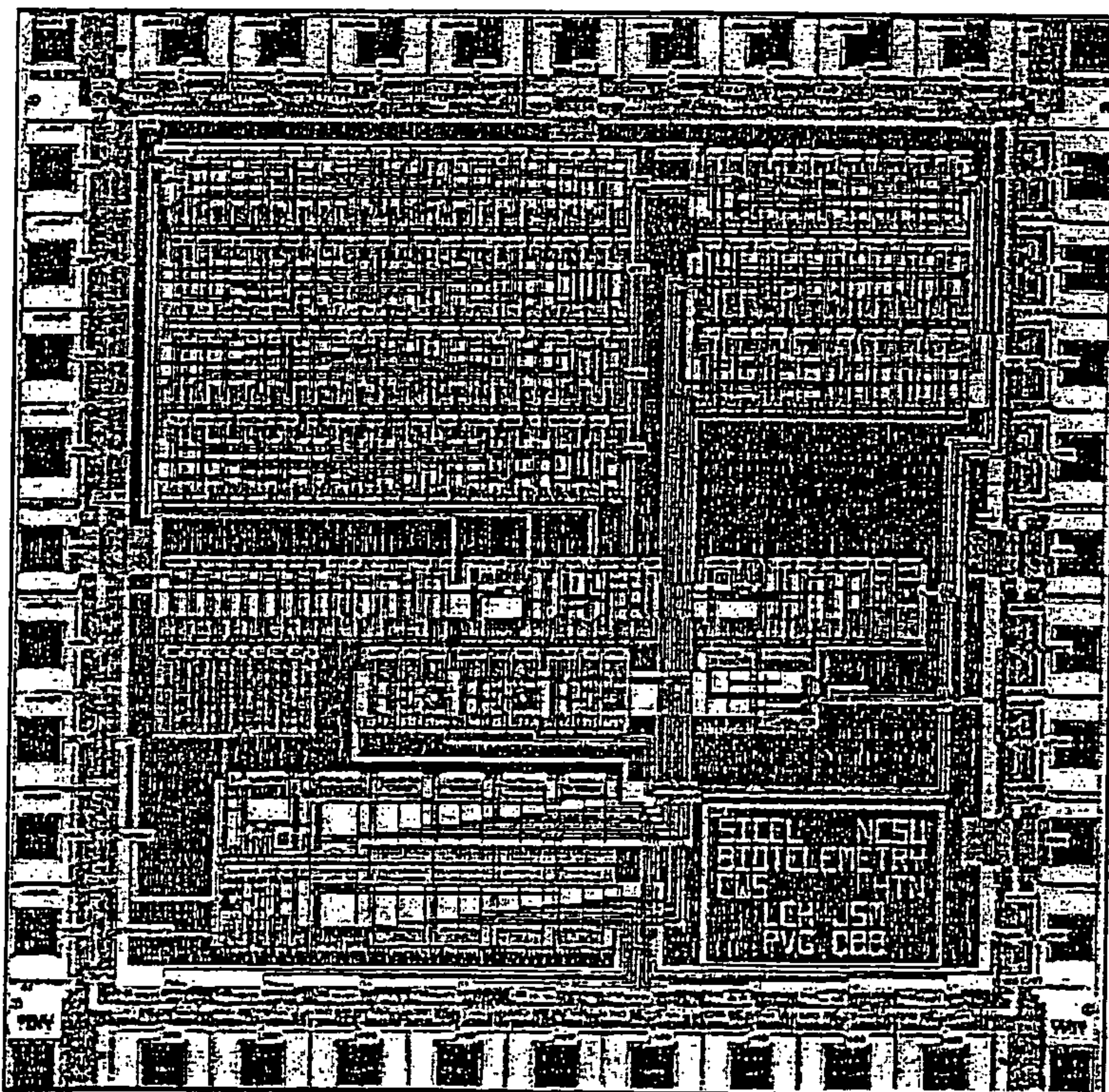
IC LAYOUT
