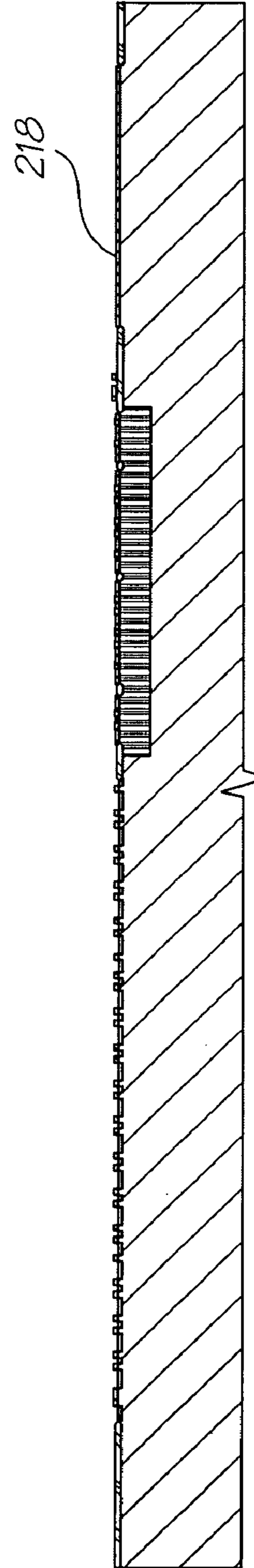
p+ implant
