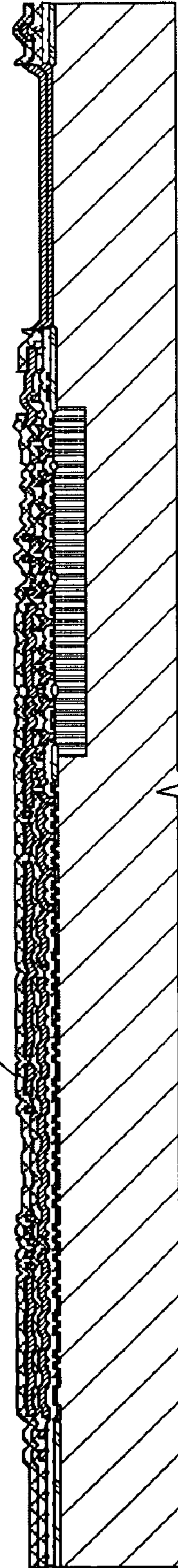
Deposit ILD 3, etch vias
