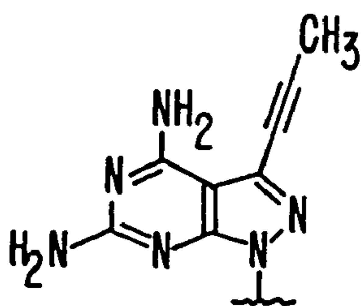
(NH 2 ) 2 PPPA
