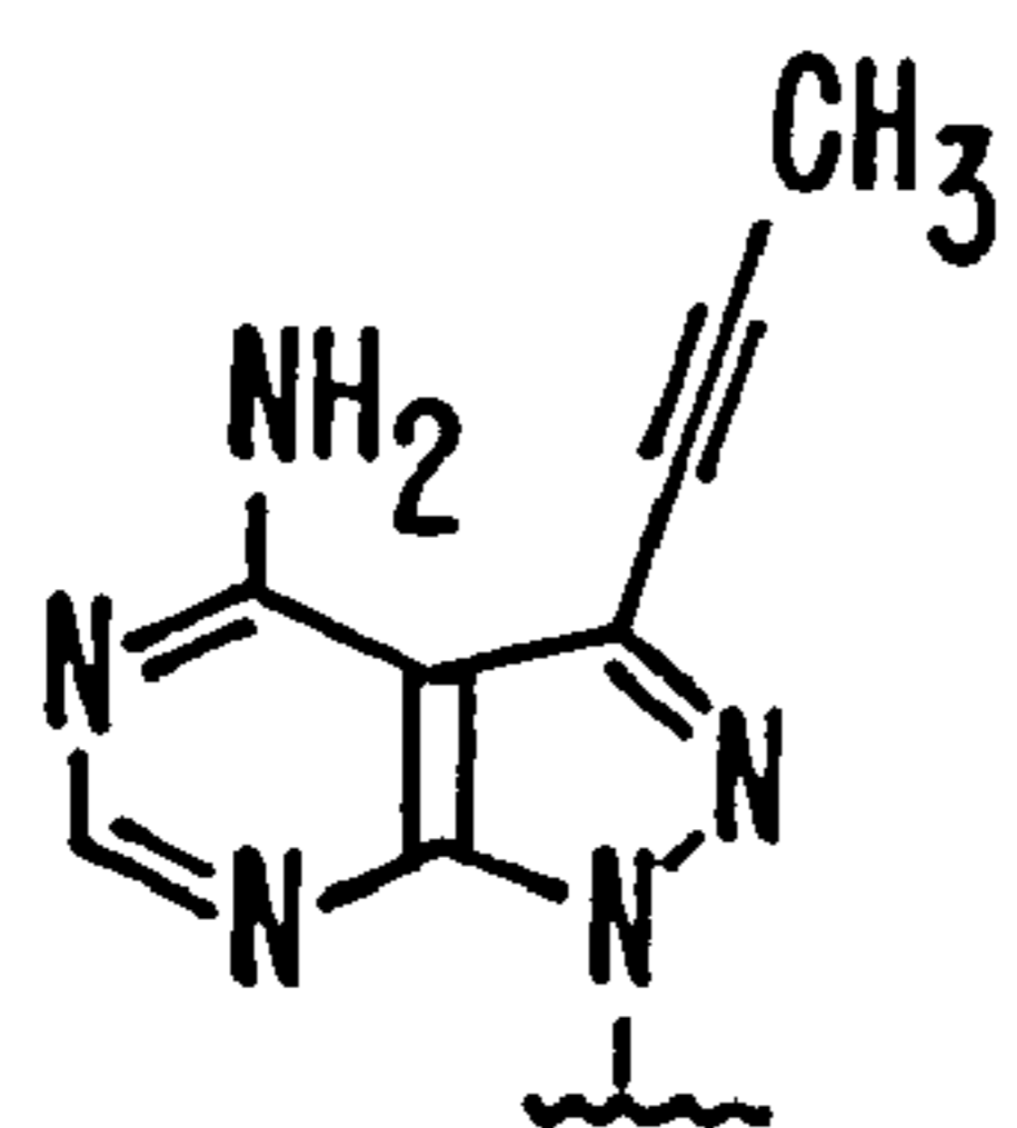
PPPA
