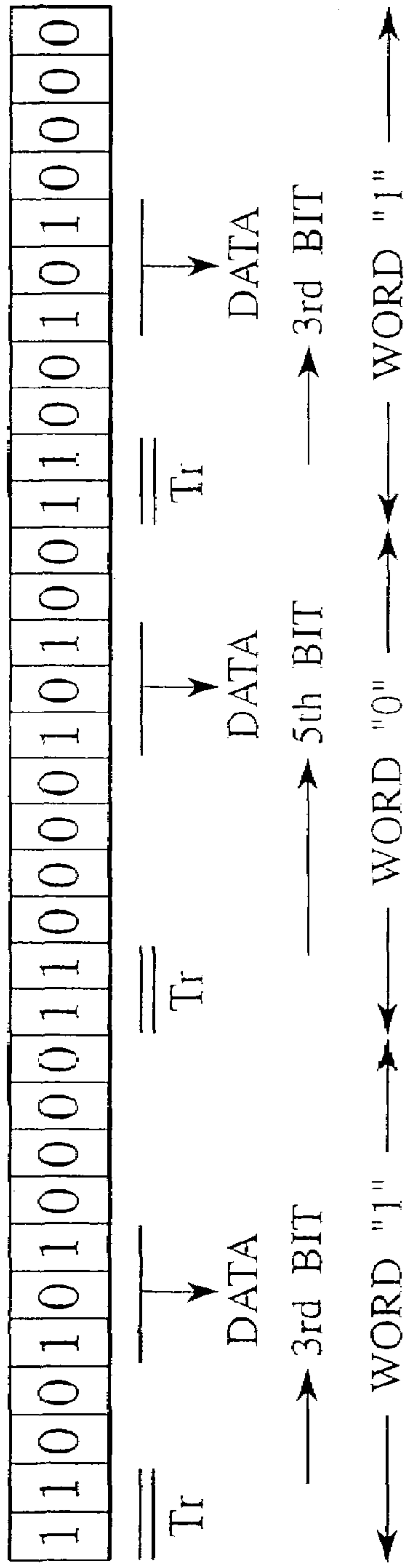
FIG.19
