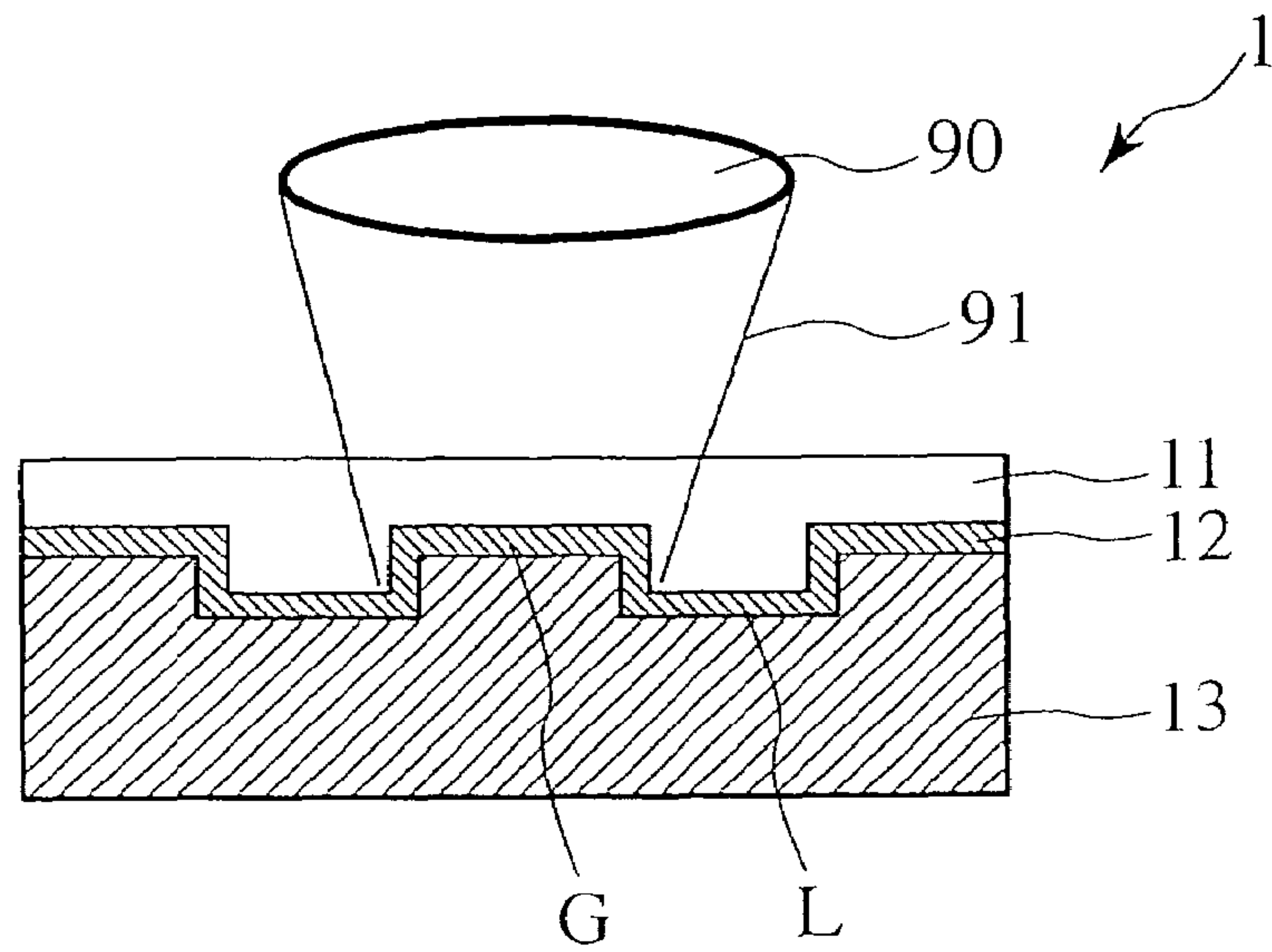
FIG. 12
