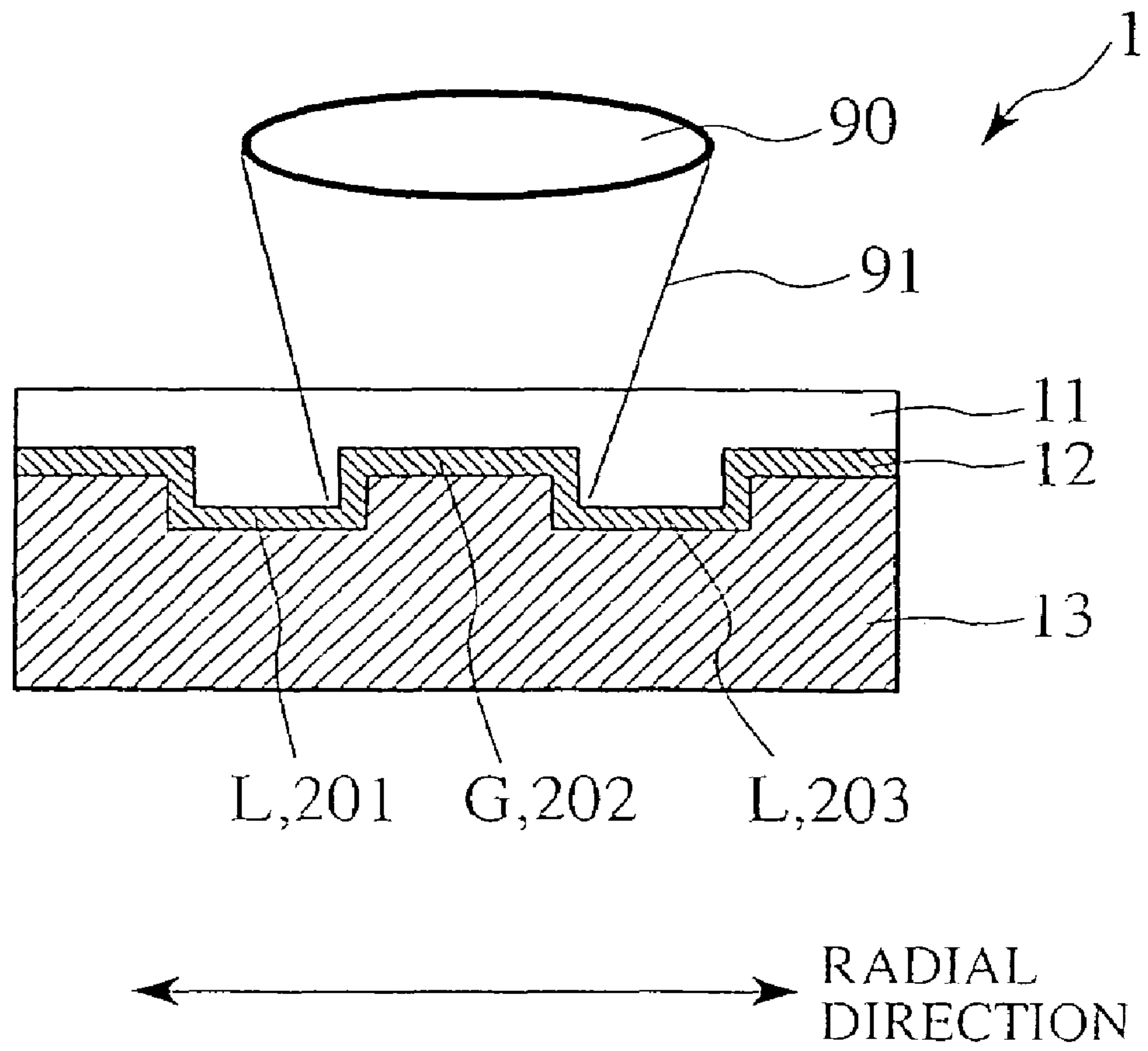
FIG. 14
