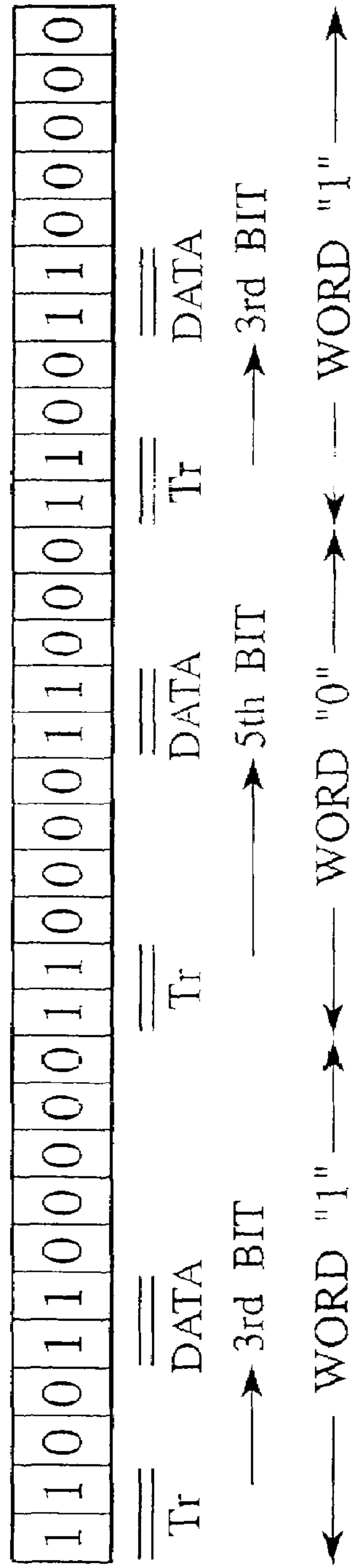
FIG.20
