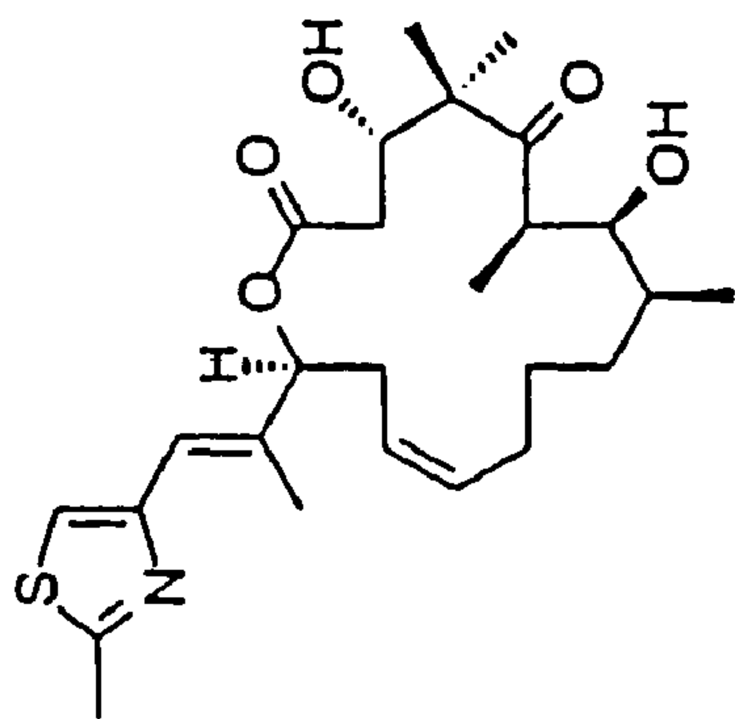
desoxyepothilone A
