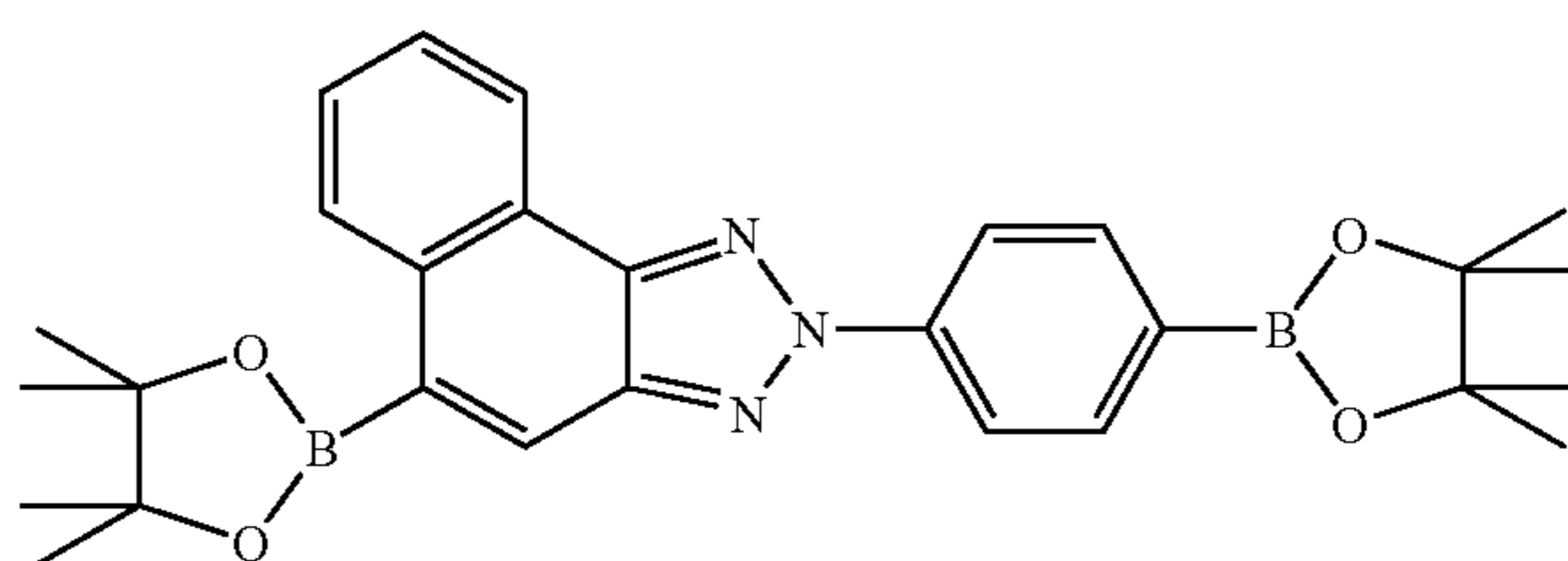
monomer 5
