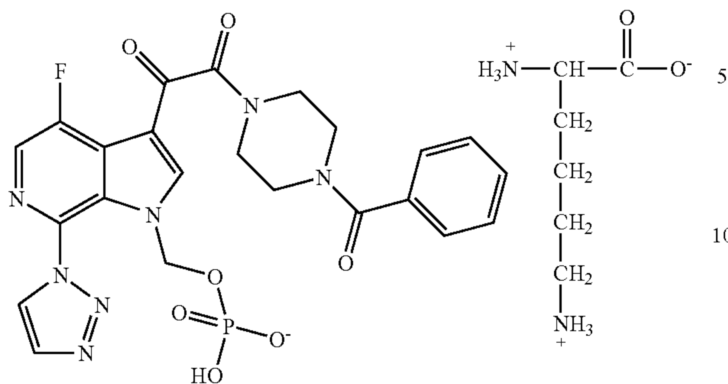
Ibb Mol. Wt. = 703.62
