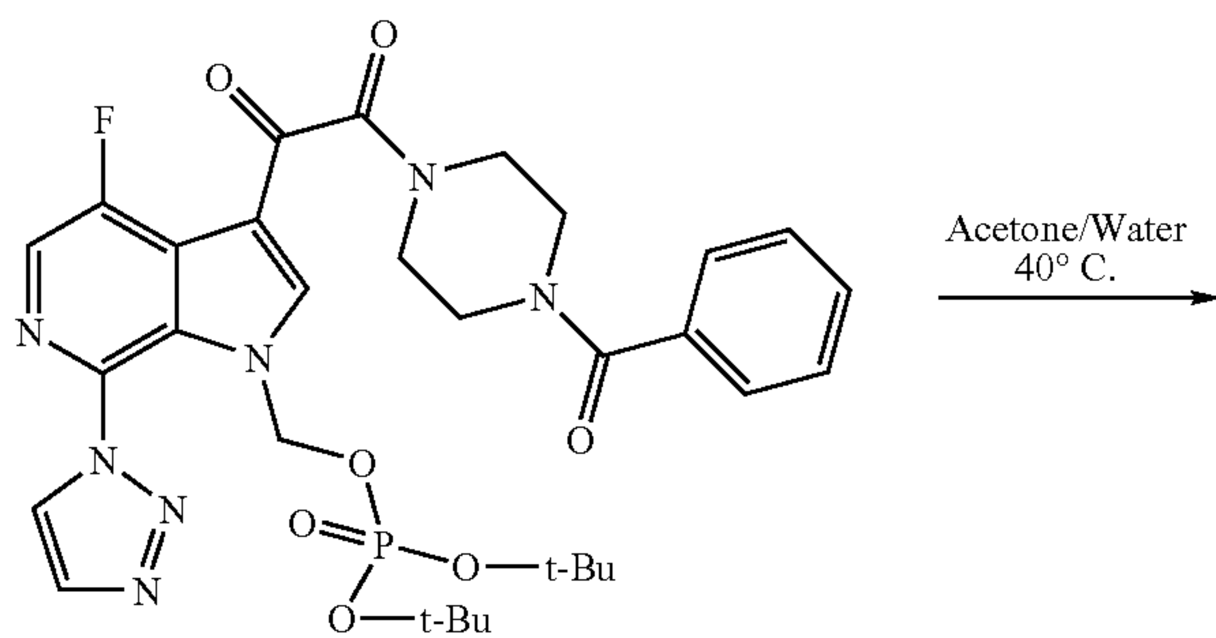
Iib Mol. Wt. = 669.64
