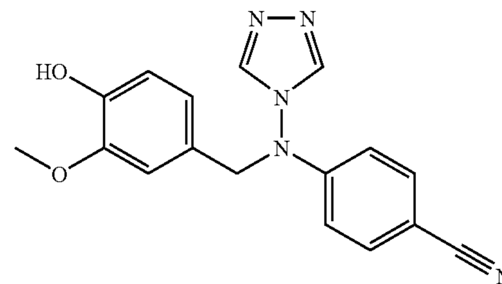
STX362
