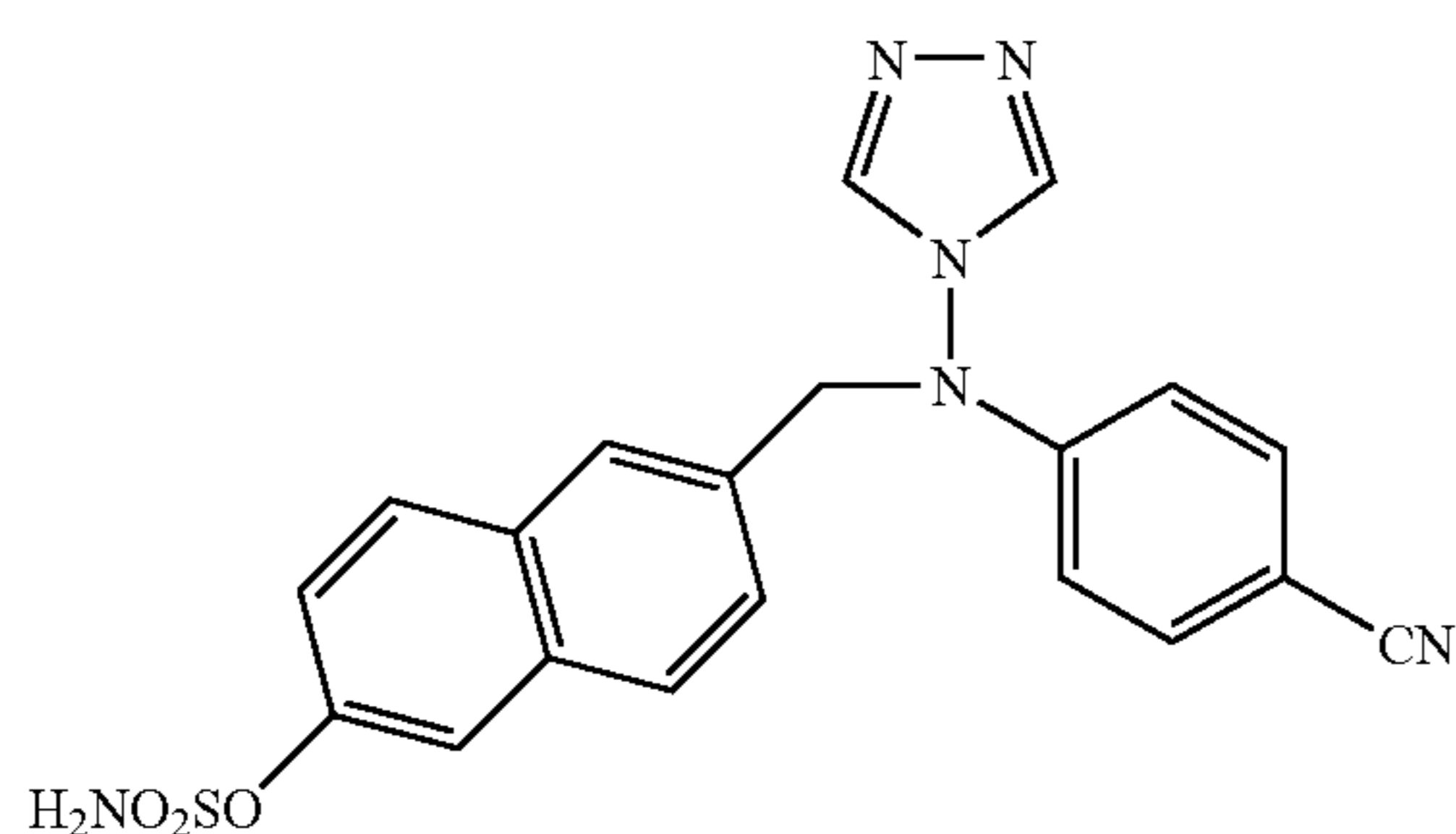
STX336
