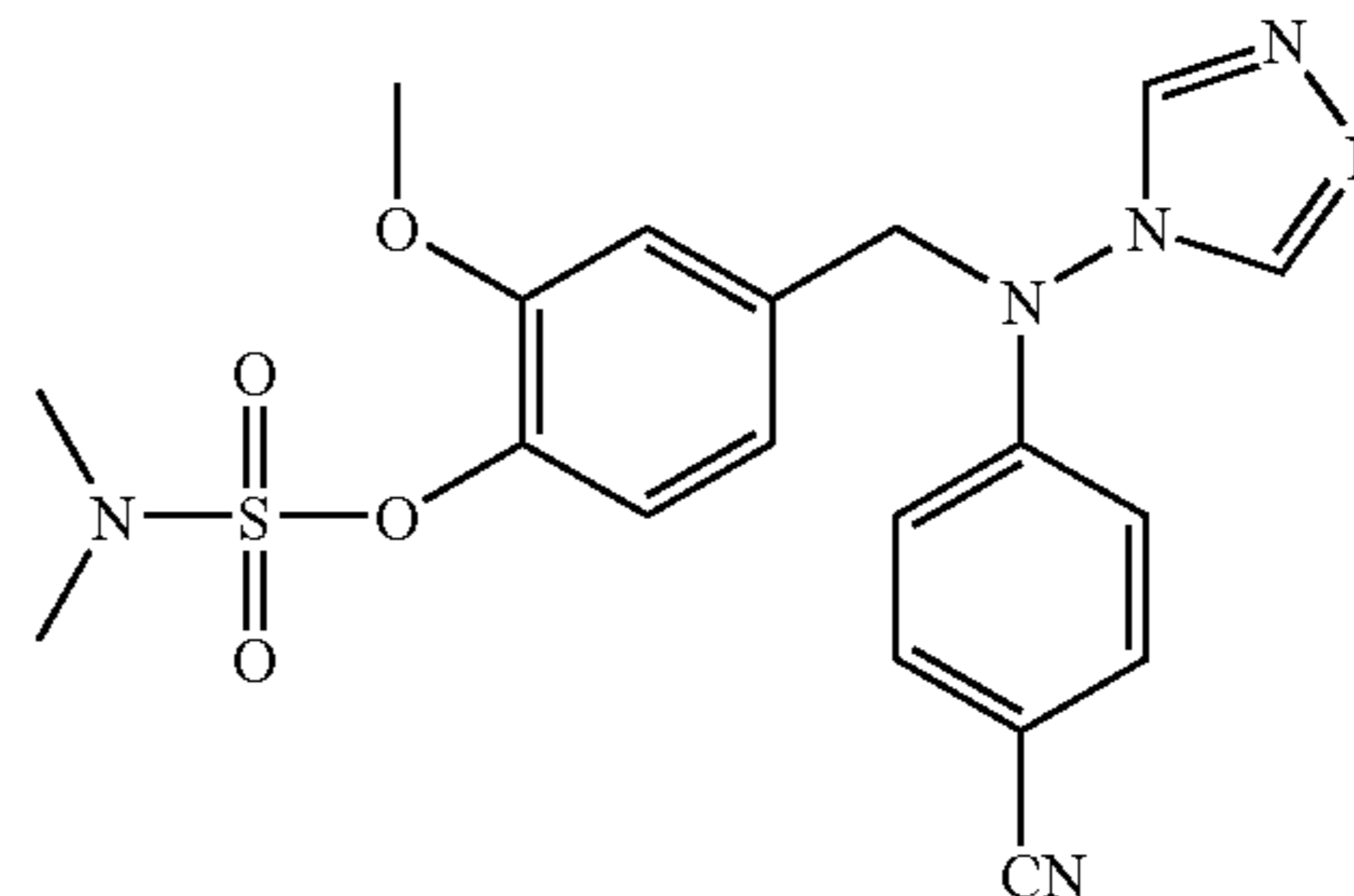
STX739
