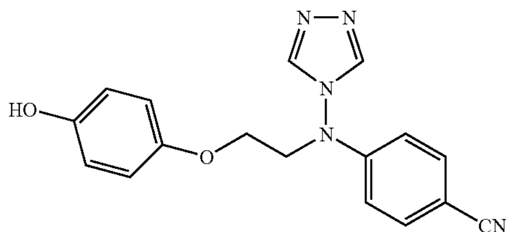
STX291
