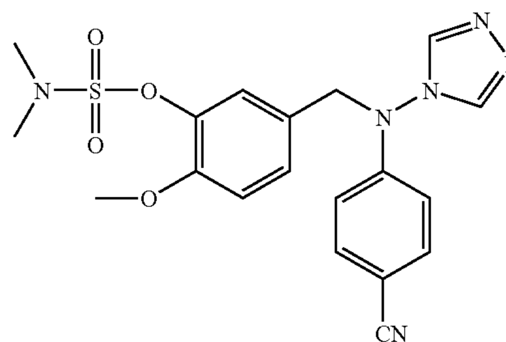
STX796
