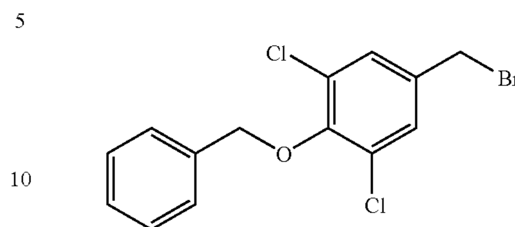
2-Benzyloxy-5-bromomethyl-1,3-dichloro-benzene (CAB02118)
