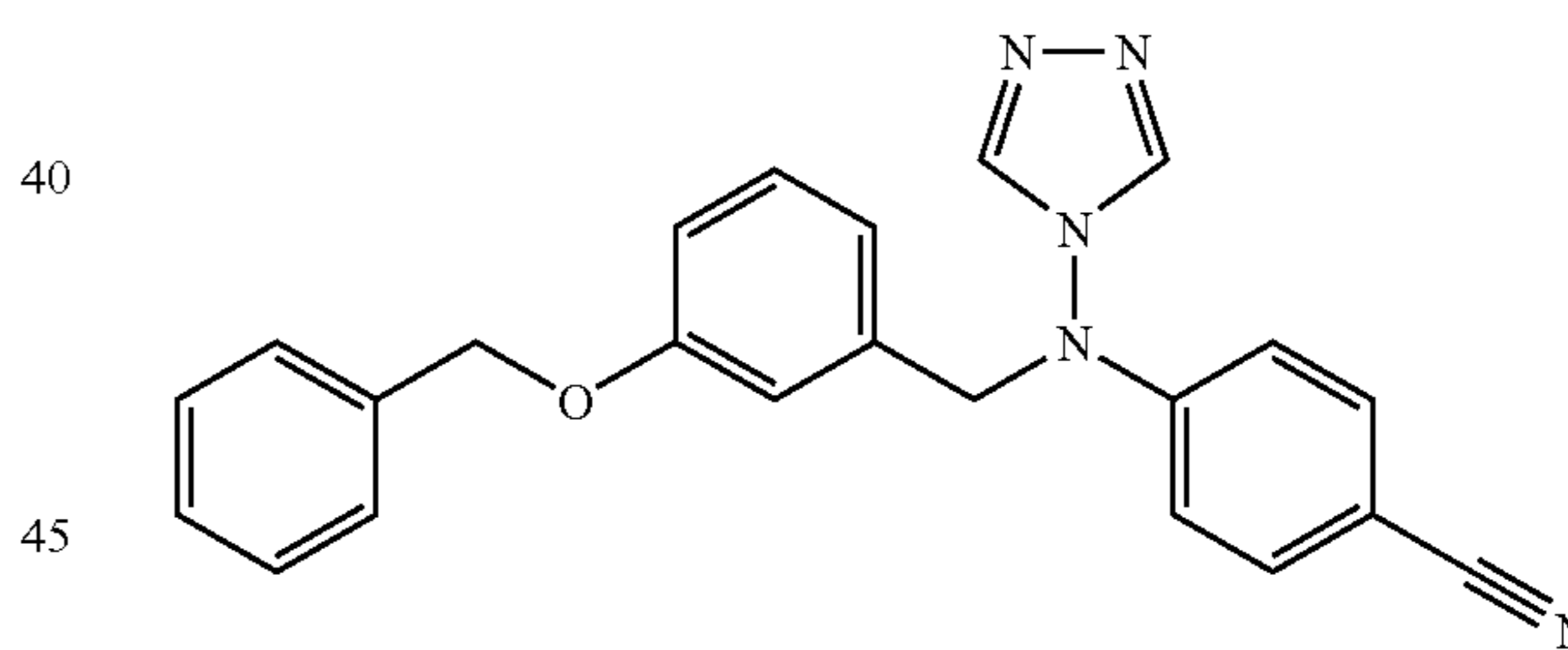
STX675
