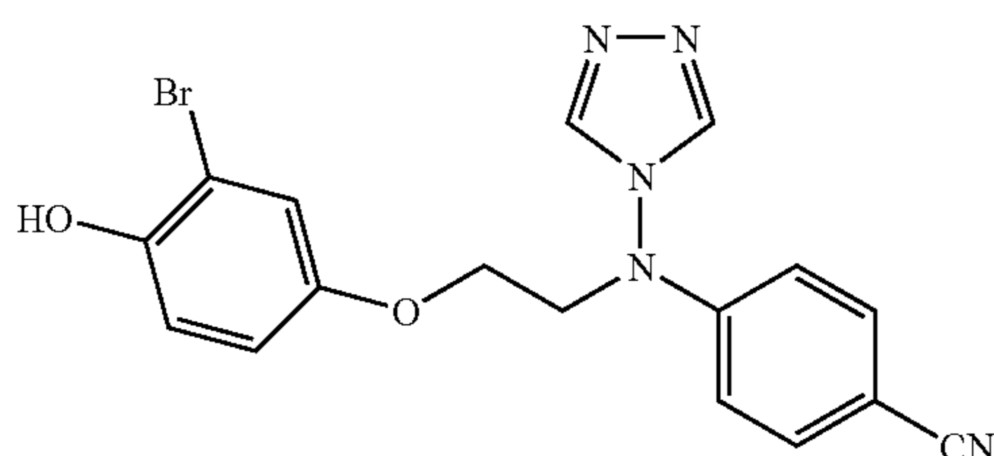
STX300
