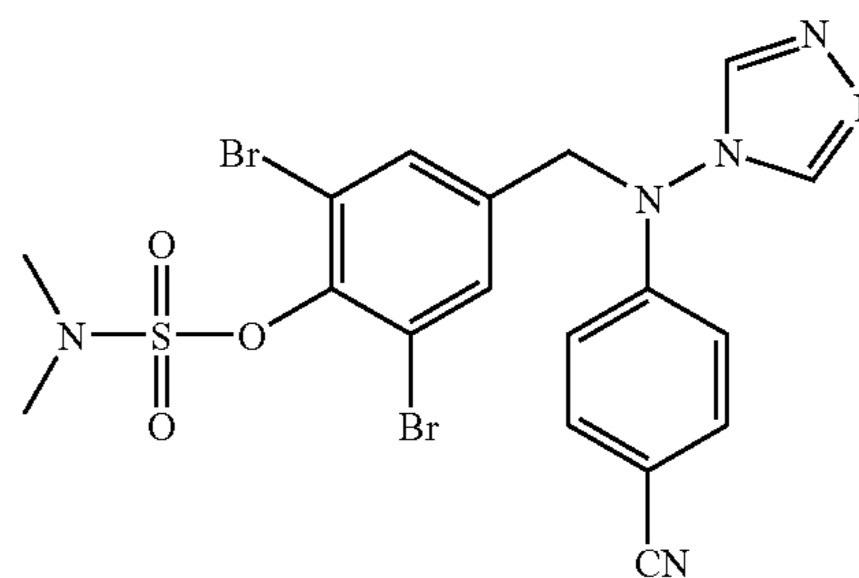
STX740
