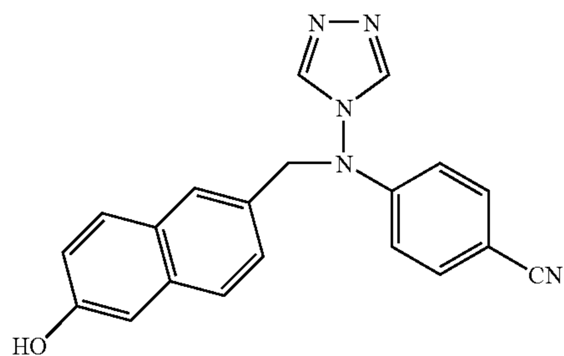
STX335
