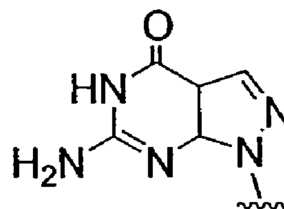
N9-(7-deaza-8-aza-G)
