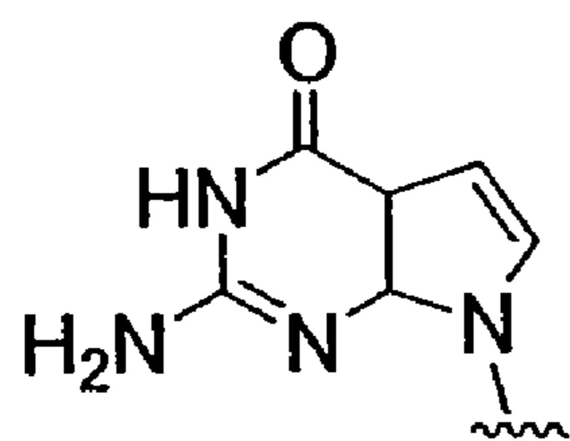
N9-(7-deaza-G)
