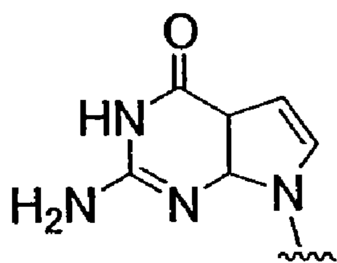
N9-(7-deaza-G)
