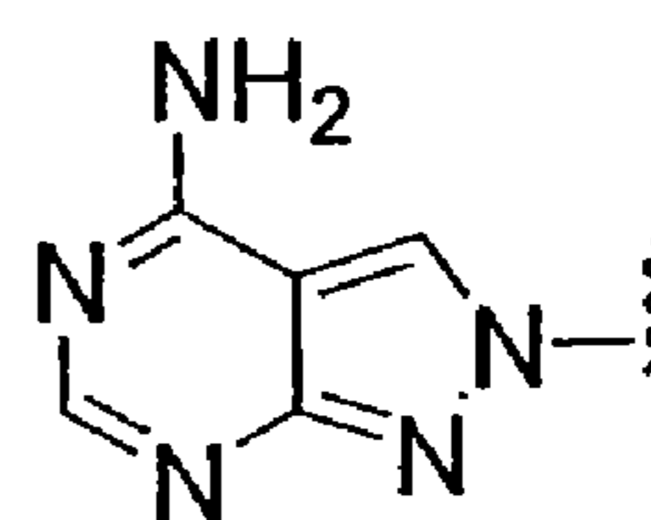
N8-(7-deaza-8-aza-A)
