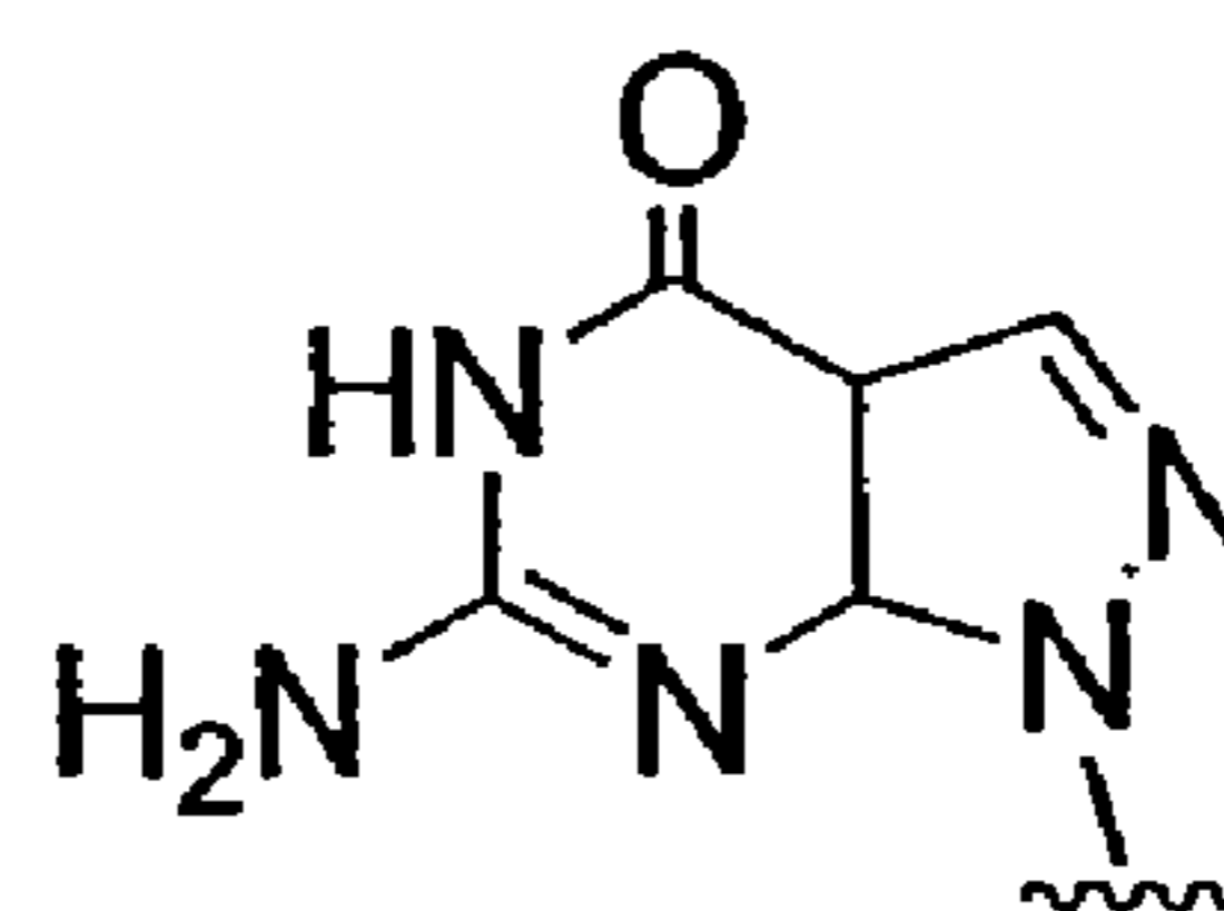
N9-(7-deaza-8-aza-G)
