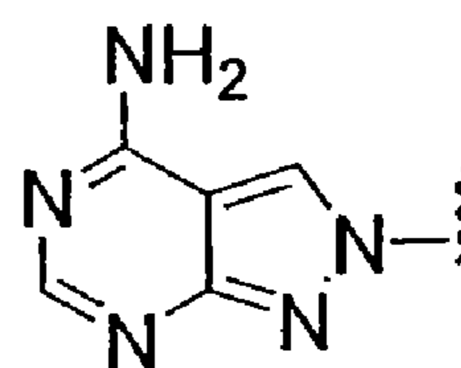
N8-(7-deaza-8-aza-A)
