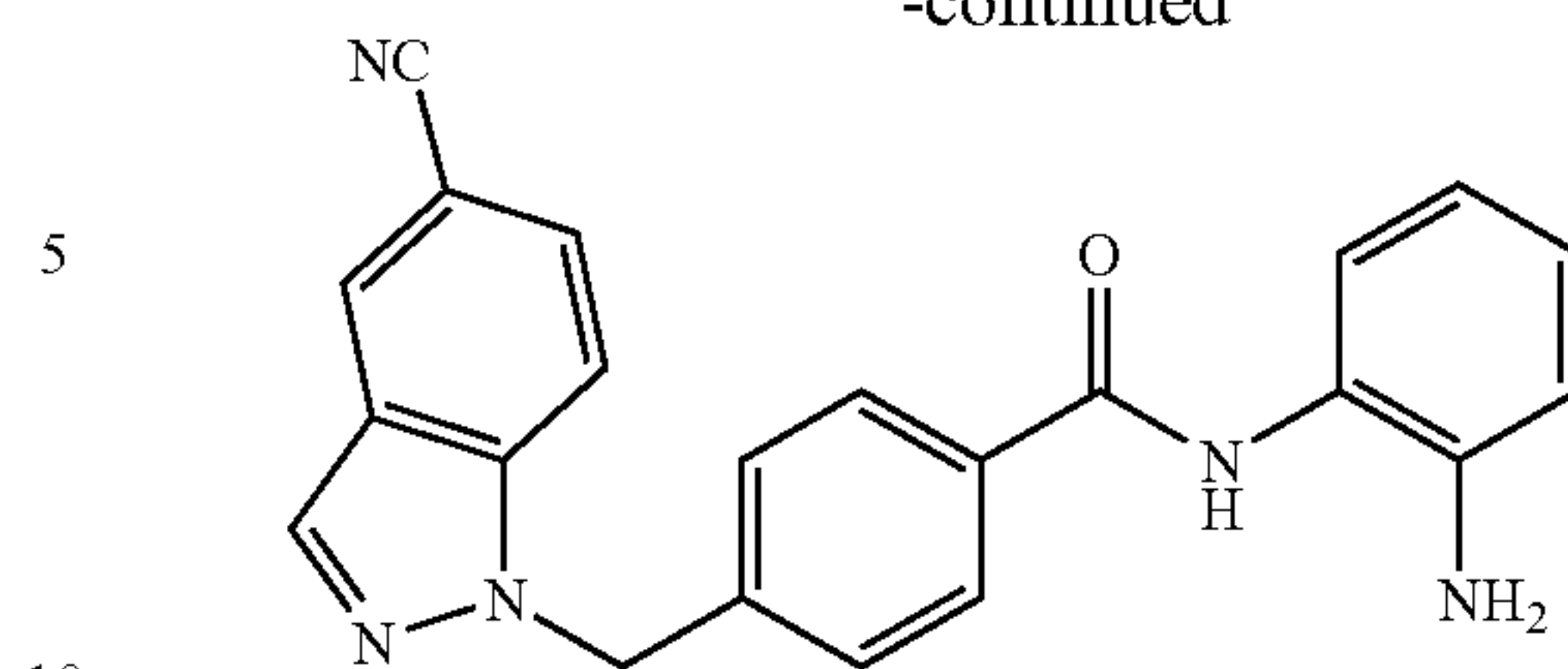
N-(2-aminophenyl)-4-((5-cyano-1H-indazol-1-yl)methyl)benzamide
