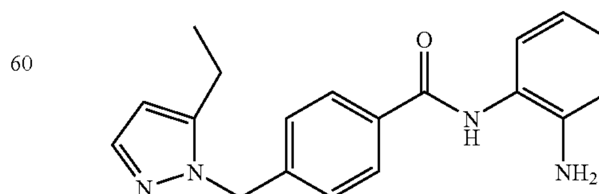
N-(2-aminophenyl)-4-((5-ethyl-1H-pyrazol-1-yl)methyl)benzamide
