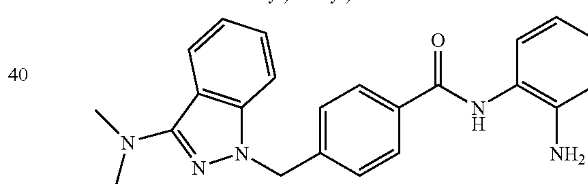
N-(2-aminophenyl)-4-((3-(dimethylamino)-1H-indazol-1-yl)methyl)benzamide
