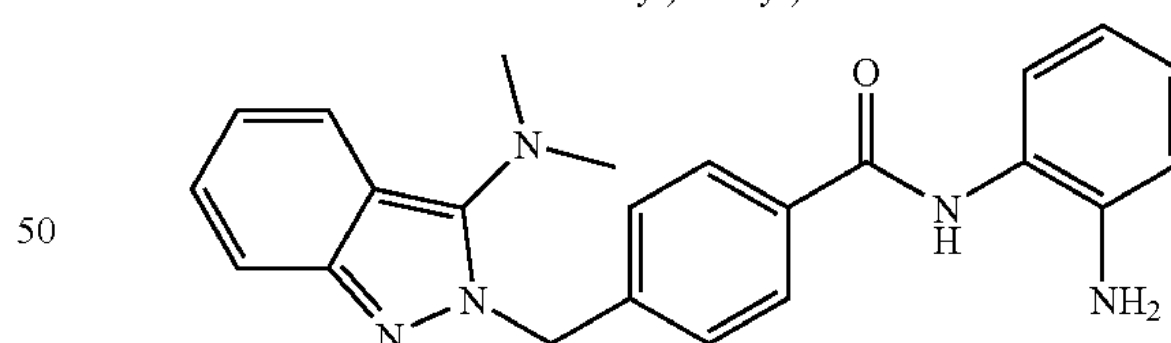
N-(2-aminophenyl)-4-((3-(dimethylamino)-2H-indazol-2-yl)methyl)benzamide
