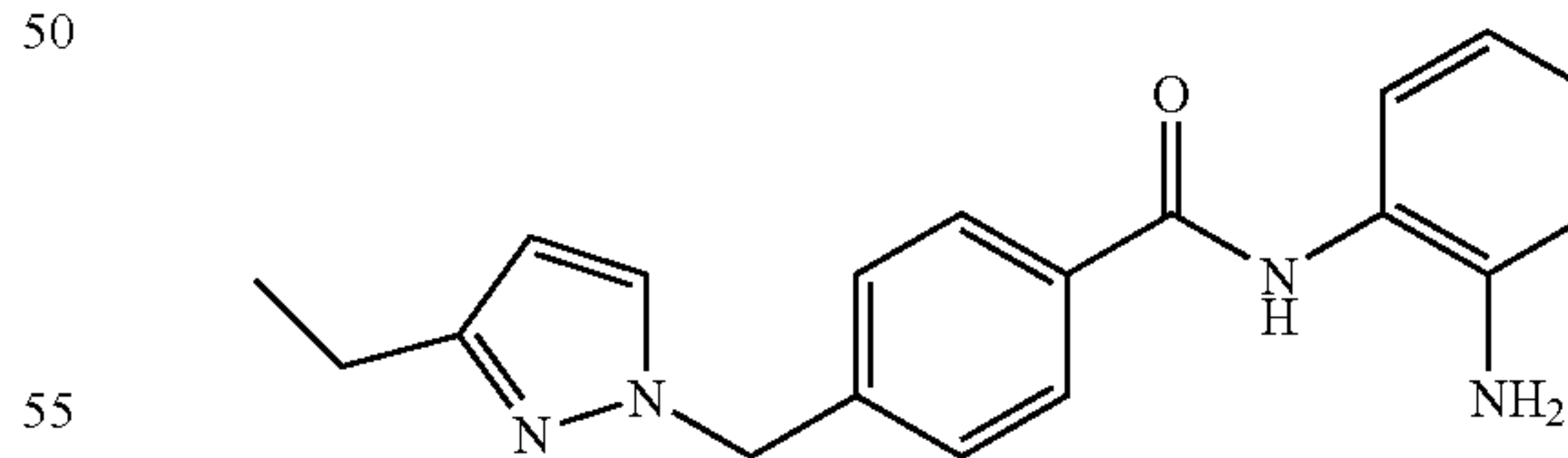
N-(2-aminophenyl)-4-((3-ethyl-1H-pyrazol-1-yl)methyl)benzamide
