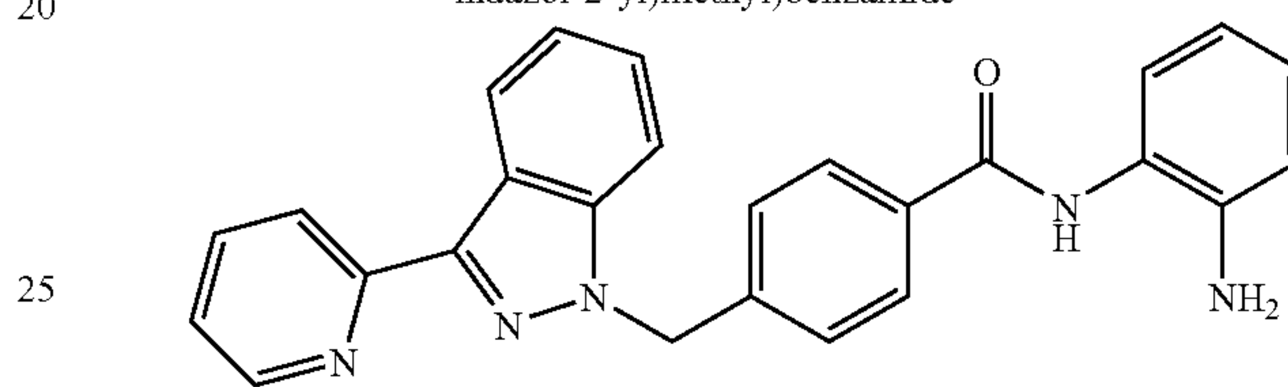
N-(2-aminophenyl)-4-((3-(pyridin-2-yl)-1H-indazol-1-yl)methyl)benzamide
