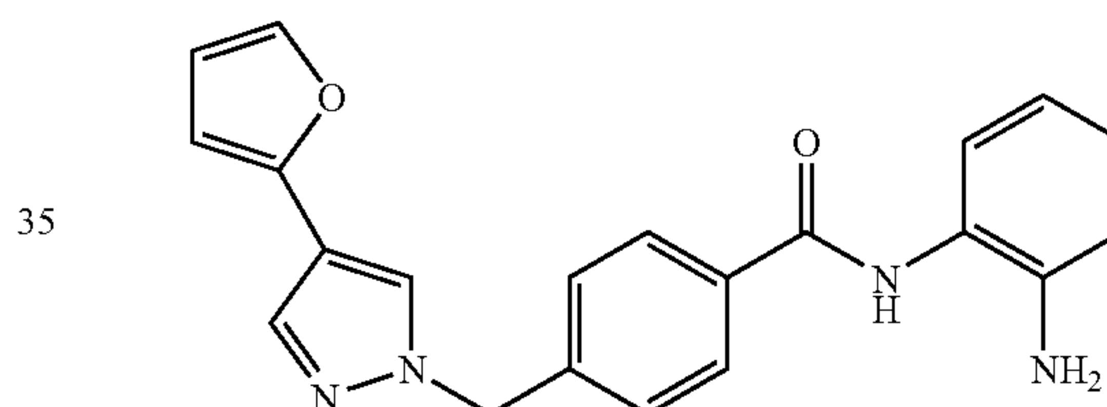
N-(2-aminophenyl)-4-((4-furan-2-yl)-1H-pyrazol-1-yl)methyl)benzamide
