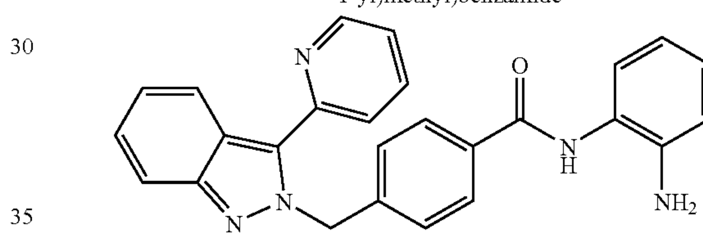
N-(2-aminophenyl)-4-((3-(pyridin-2-yl)-2H-indazol-2-yl)methyl)benzamide
