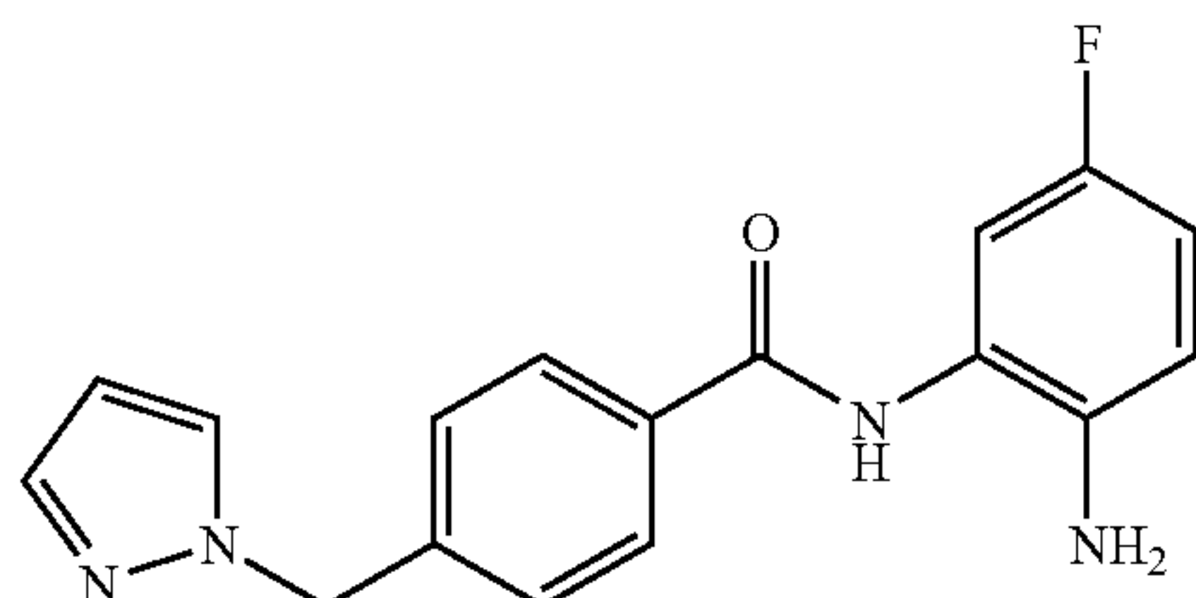
4-((1H-pyrazol-1-yl)methyl)-N-(2-amino-5-fluorophenyl)benzamide
