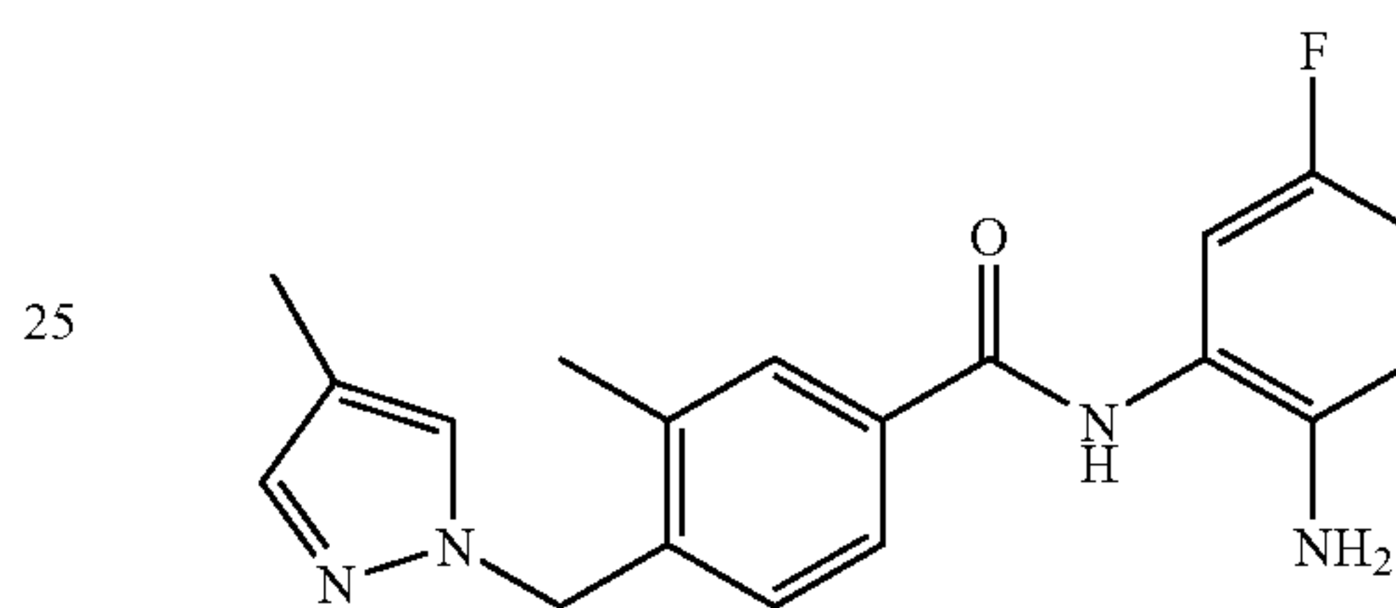
N-(2-amino-5-fluorophenyl)-3-methyl-4-((4-methyl-1H-pyrazol-1-yl)methyl)benzamide
