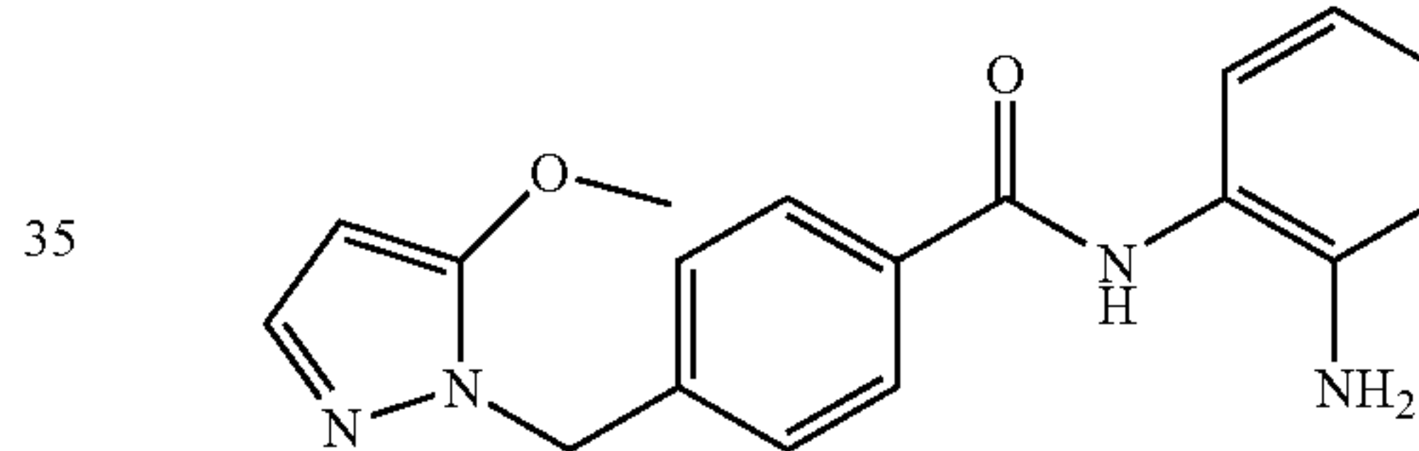
N-(2-aminophenyl)-4-((5-methoxy-1H-pyrazol-1-yl)methyl)benzamide
