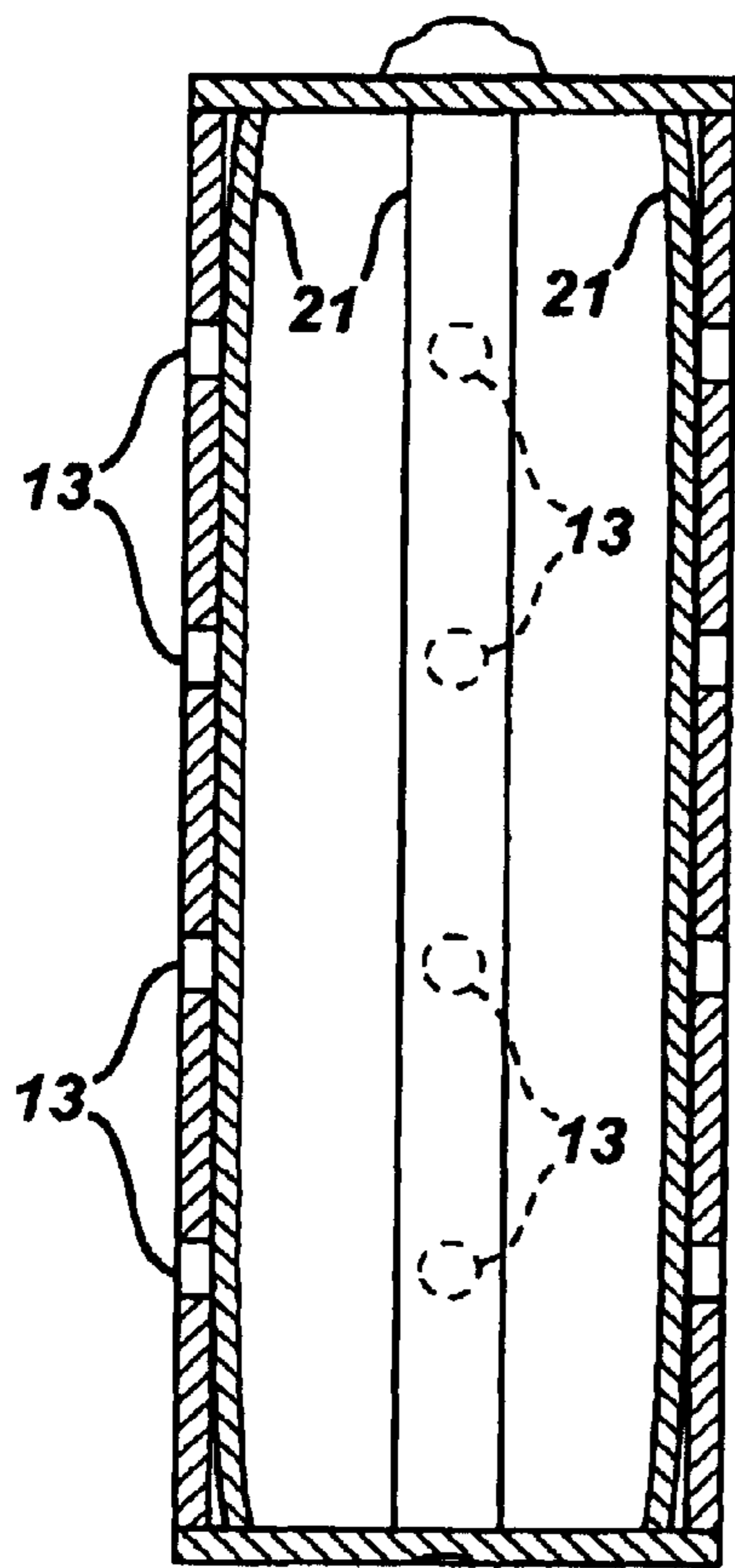
FIG. 2A
