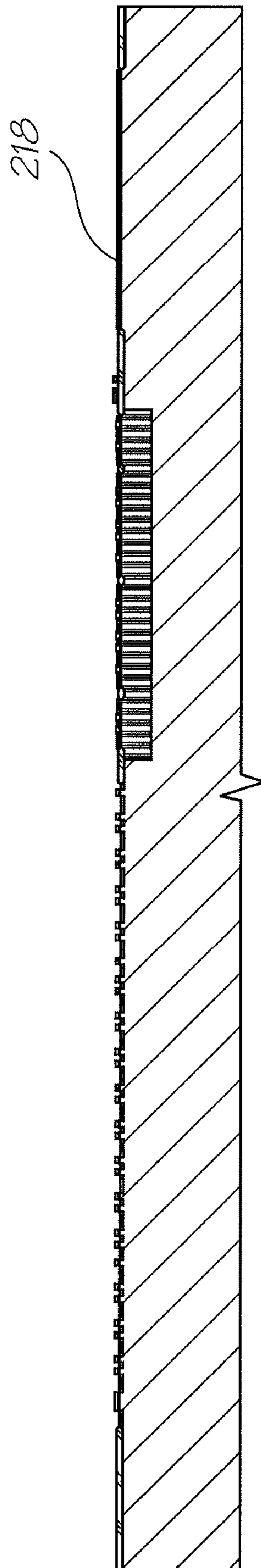
p+ implant
