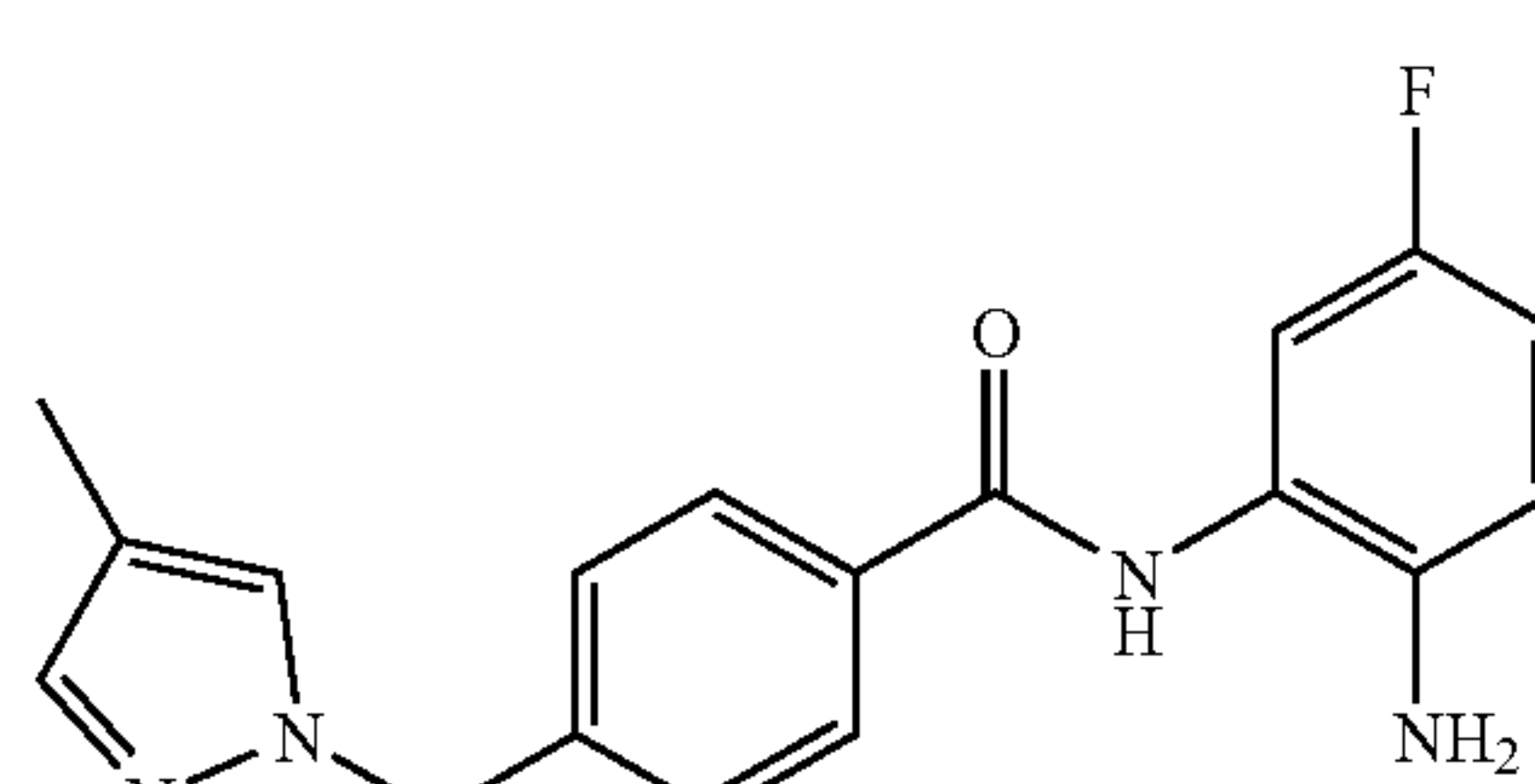
N-(2-amino-5-fluorophenyl)-4-((4-methyl-1H-pyrazol-1-yl)methyl)benzamide
