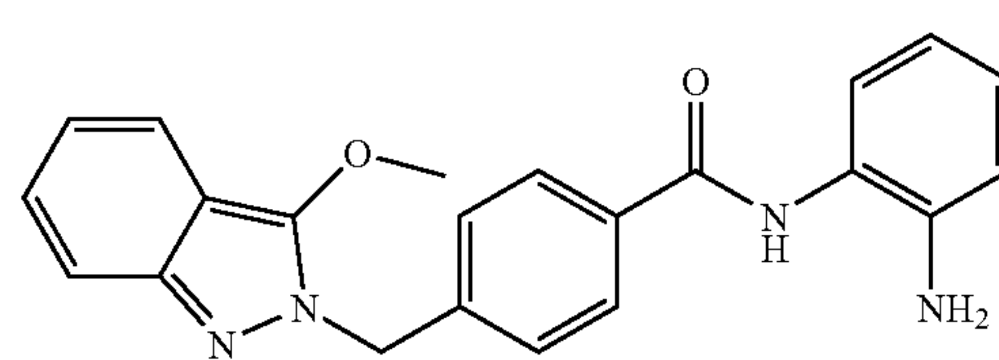
N-(2-aminophenyl)-4-((3-methoxy-2H-indazol-2-yl)methyl)benzamide
