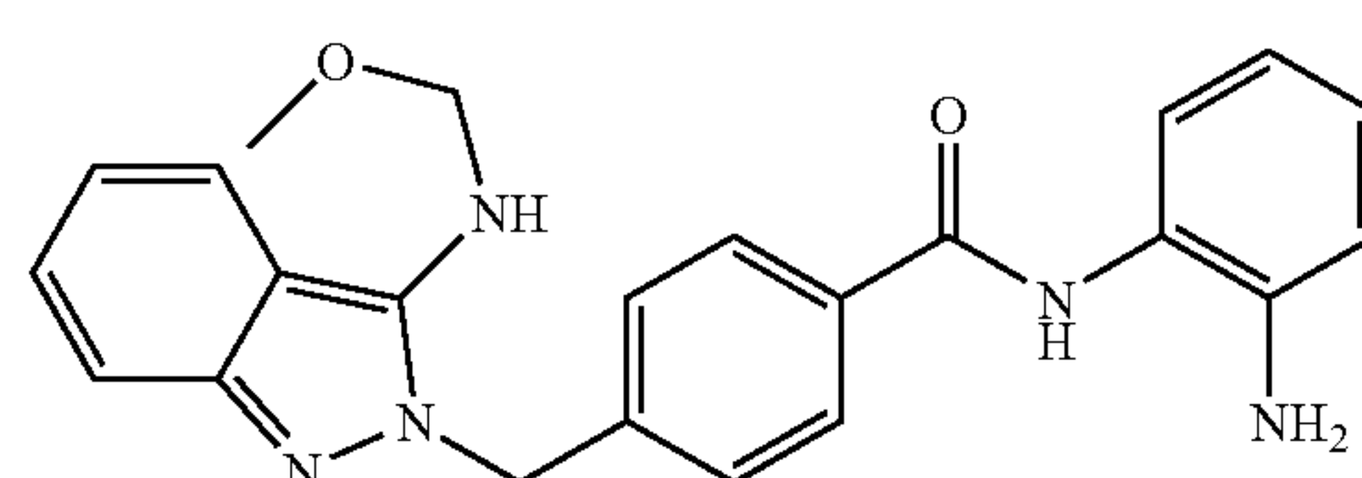
N-(2-aminophenyl)-4-((3-(methoxymethylamino)-2H-indazol-2-yl)methyl)benzamide
