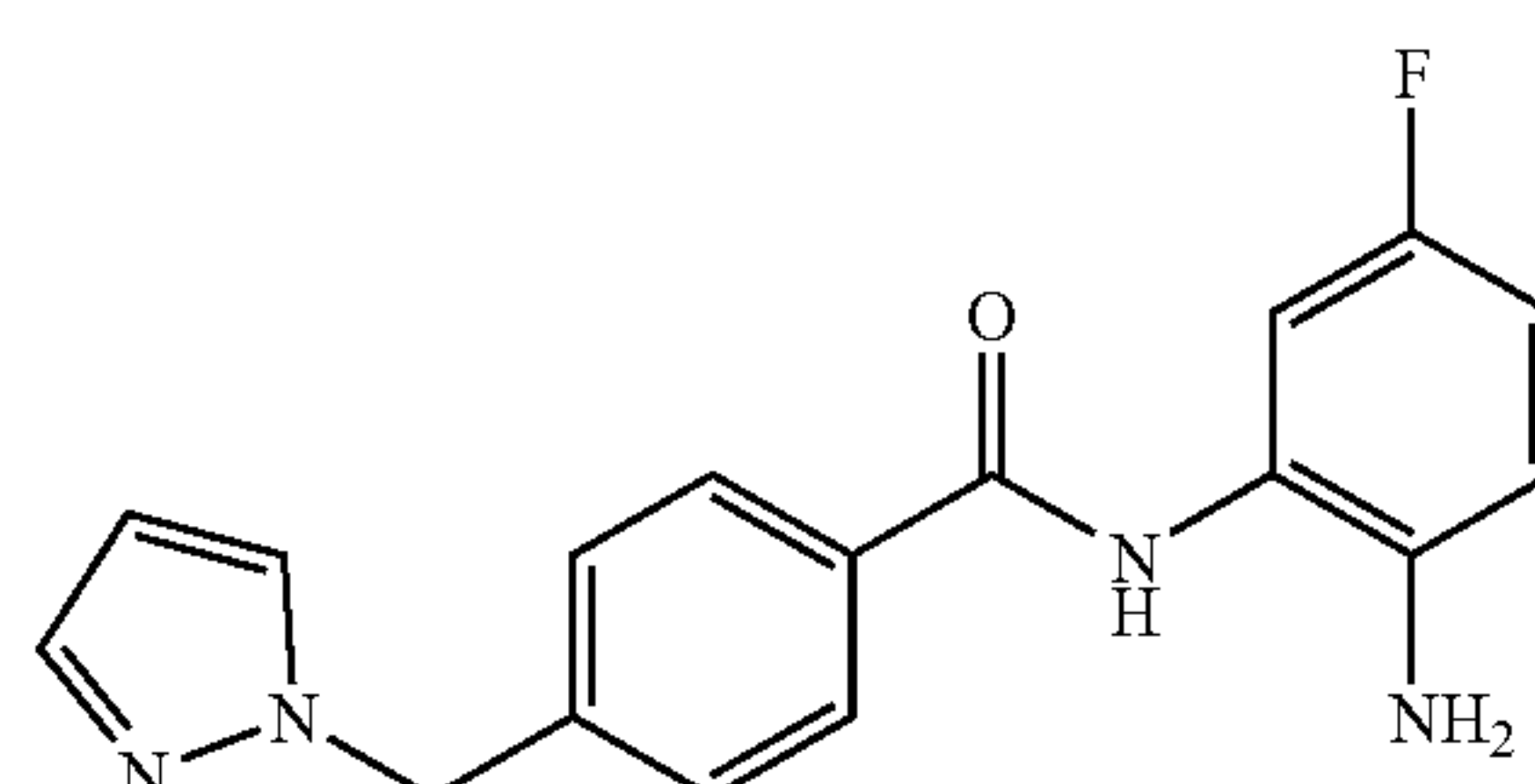
4-((1H-pyrazol-1-yl)methyl)-N-(2-amino-5-fluorophenyl)benzamide
