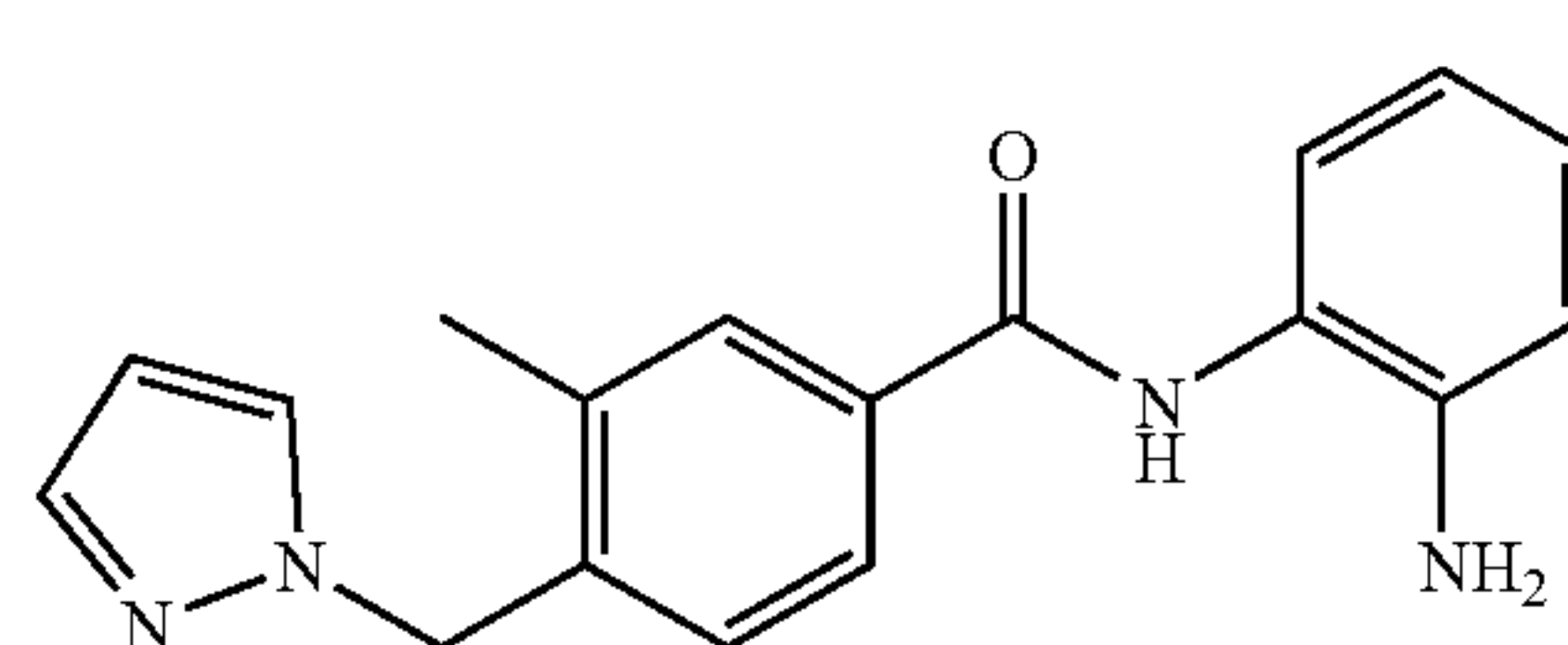
4-((1H-pyrazol-1-yl)methyl)-N-(2-aminophenyl)-3-methylbenzamide
