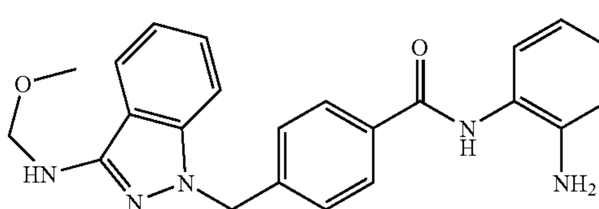
N-(2-aminophenyl)-4-((3-(methoxymethylamino)-1H-indazol-1-yl)methyl)benzamide
