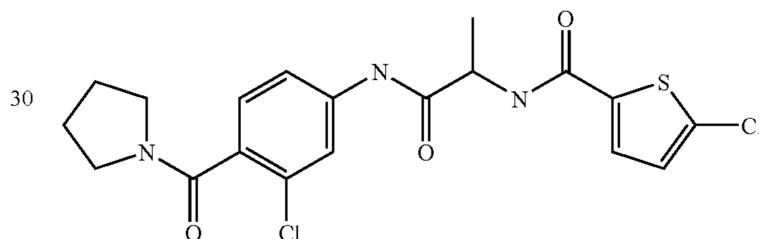
(a) 3-chloro-4-(pyrrolidin-1-yl-carbonyl)-1-nitro-benzene
