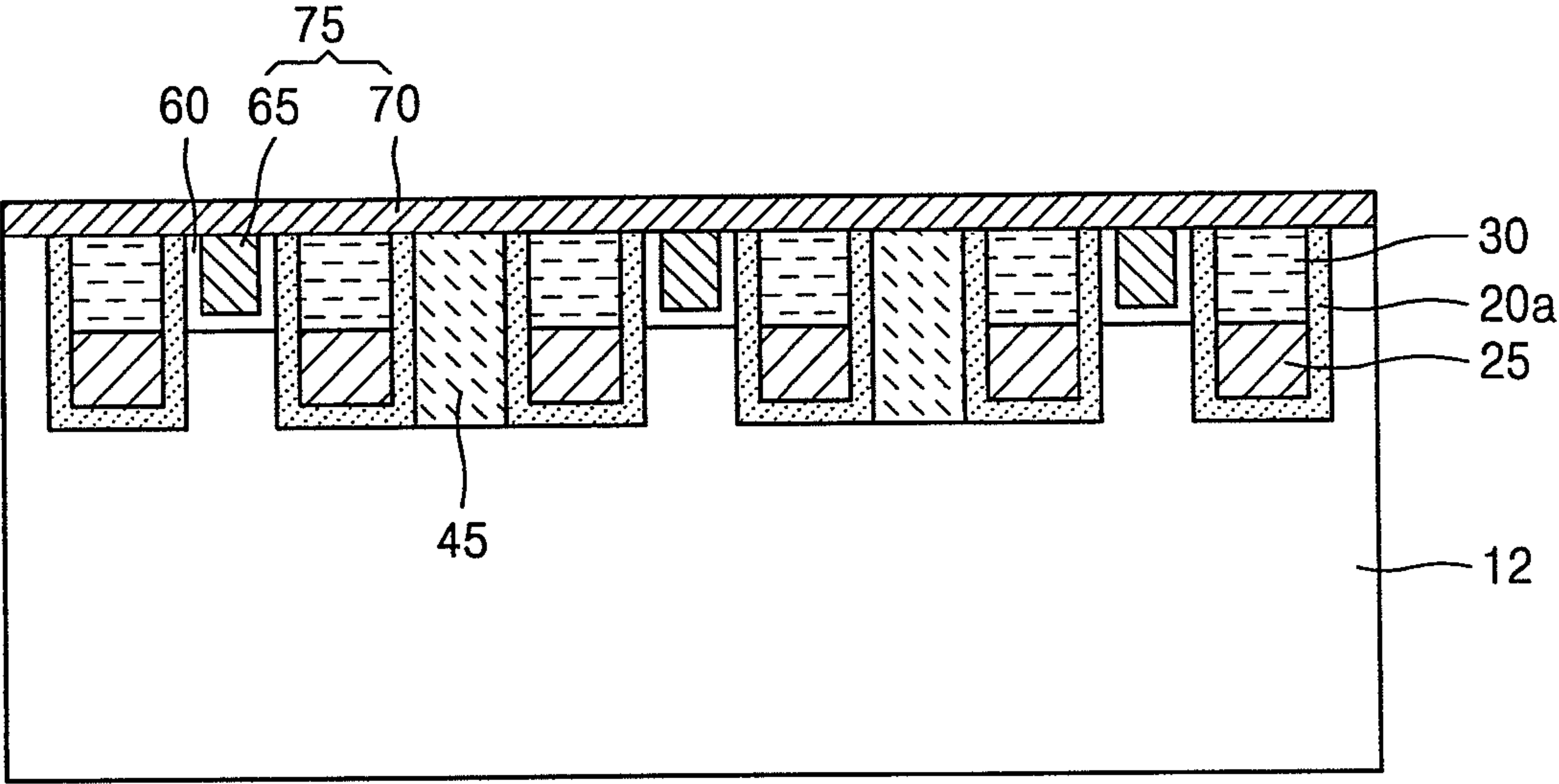
FIG. 16A
