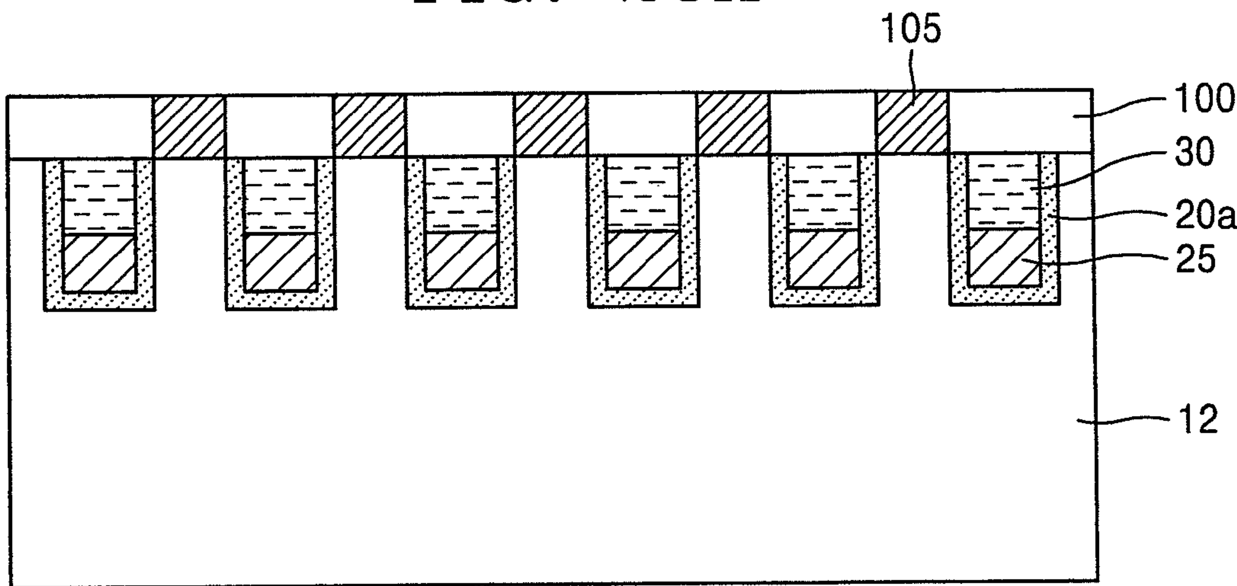
FIG. 23A
