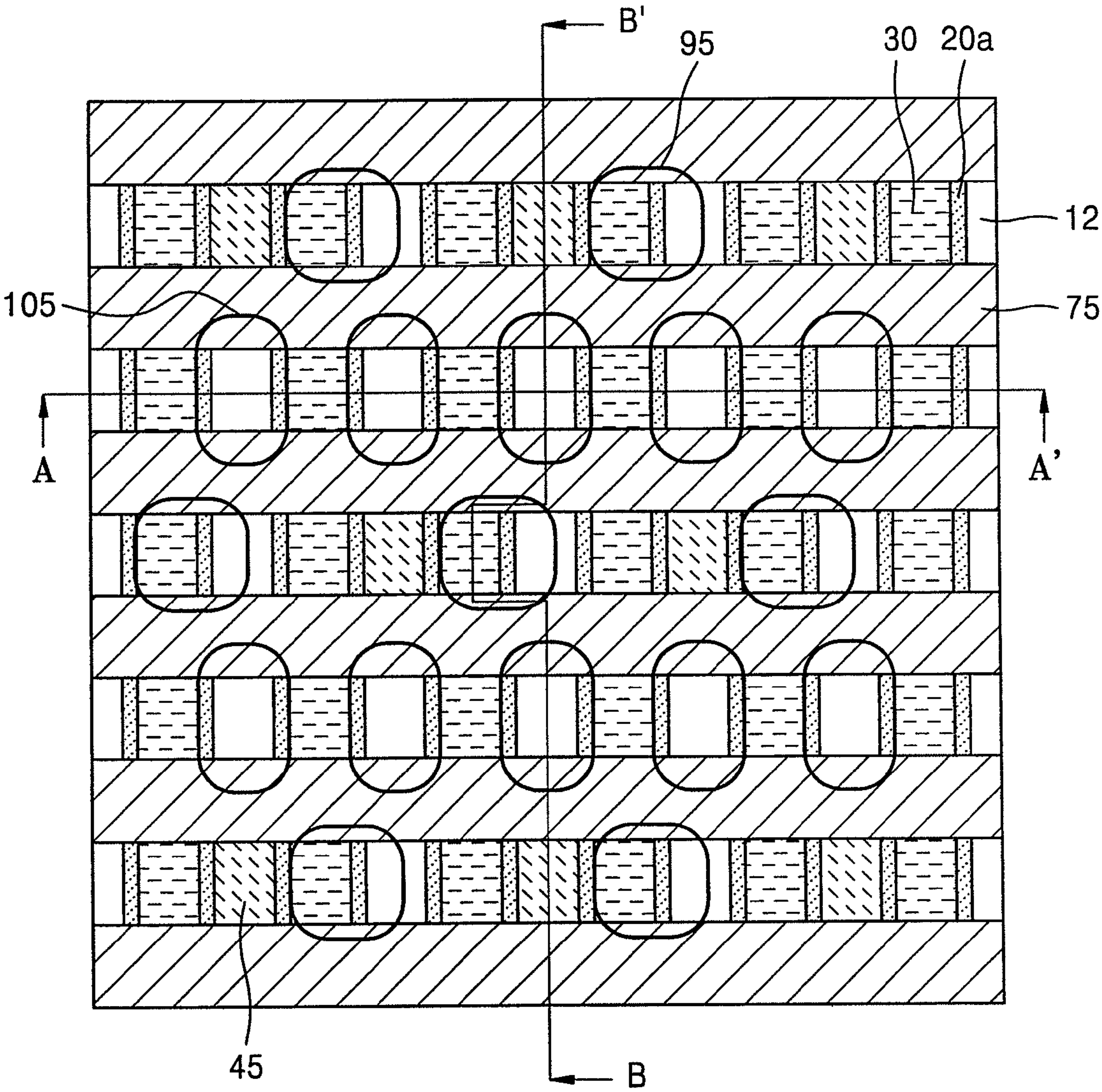
FIG. 22
