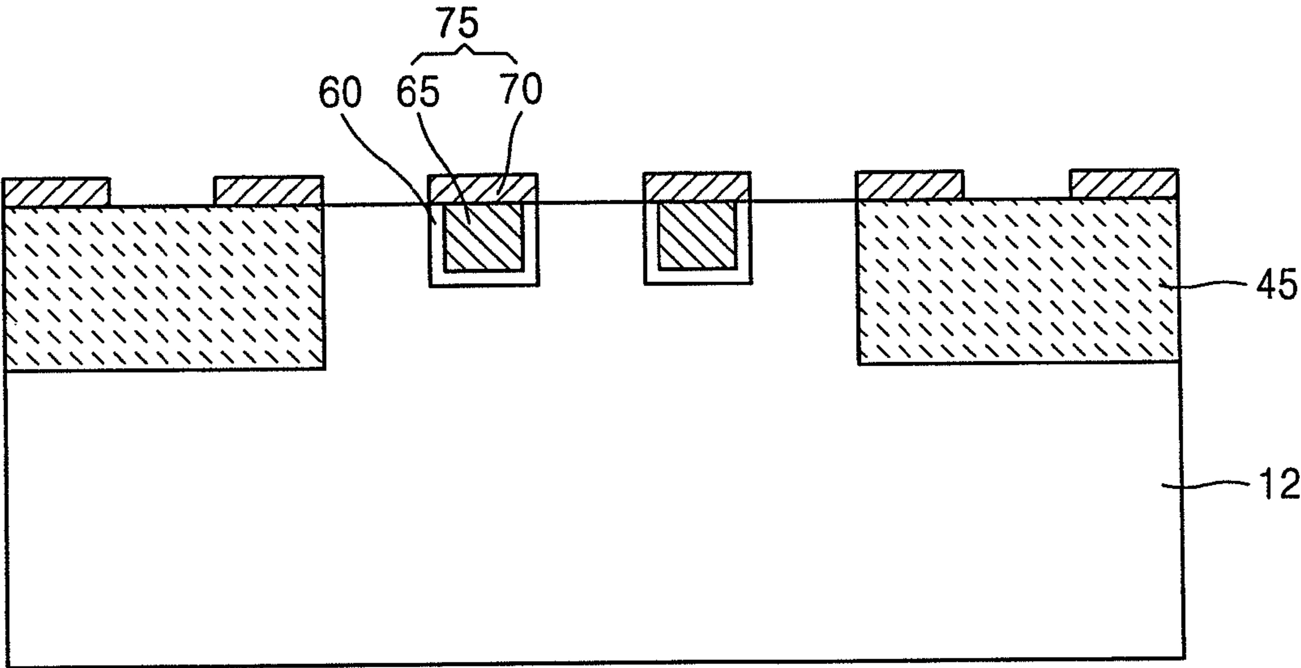
FIG. 16B
