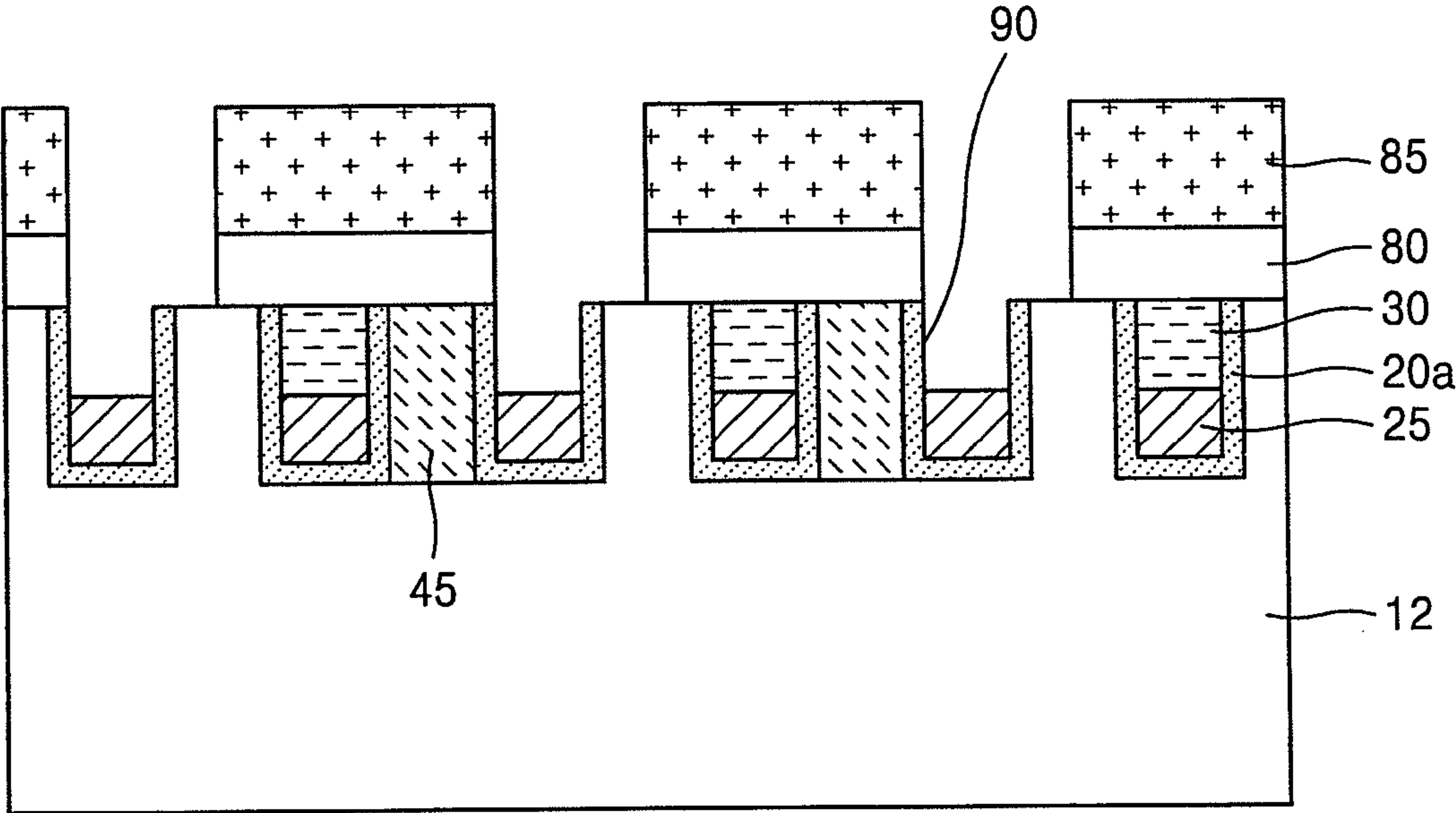
FIG. 19A
