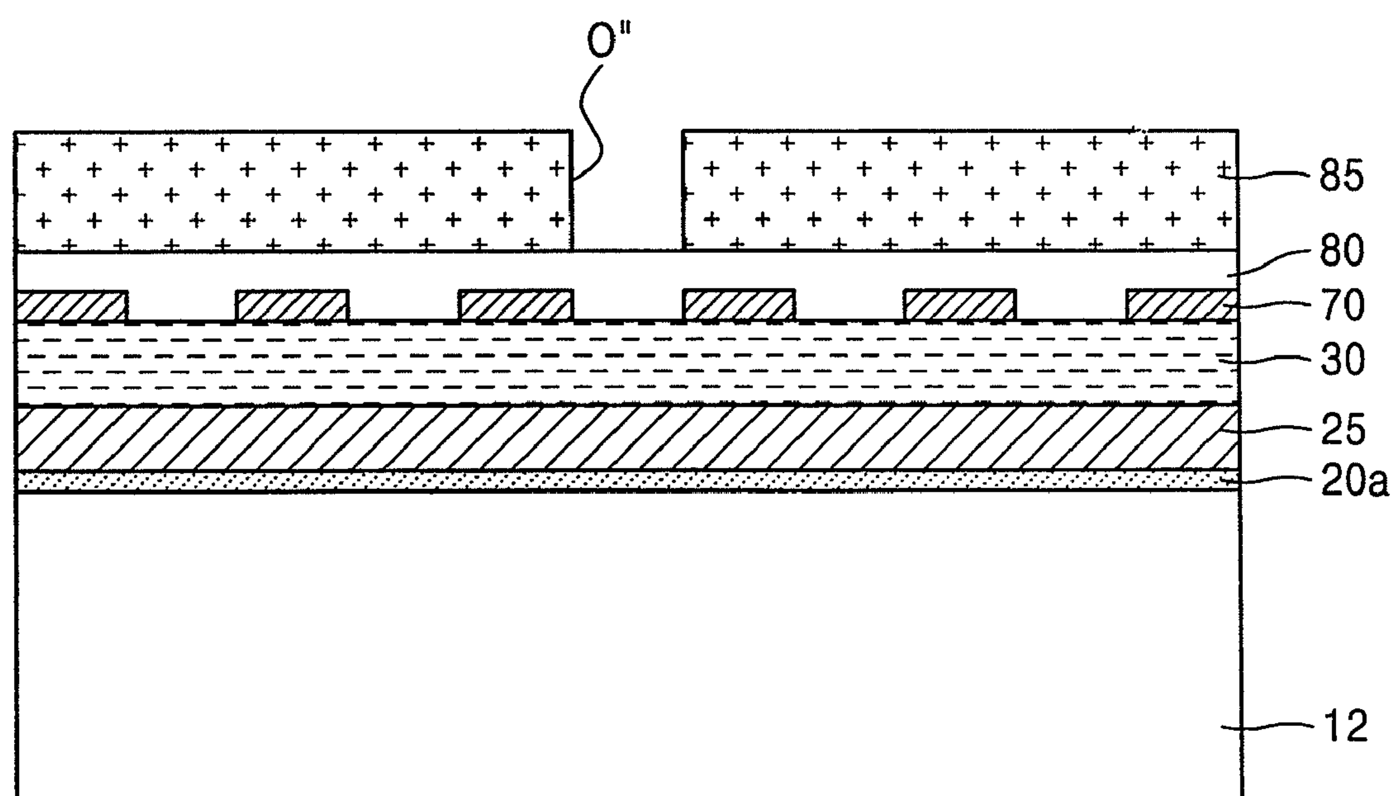
FIG. 18B
