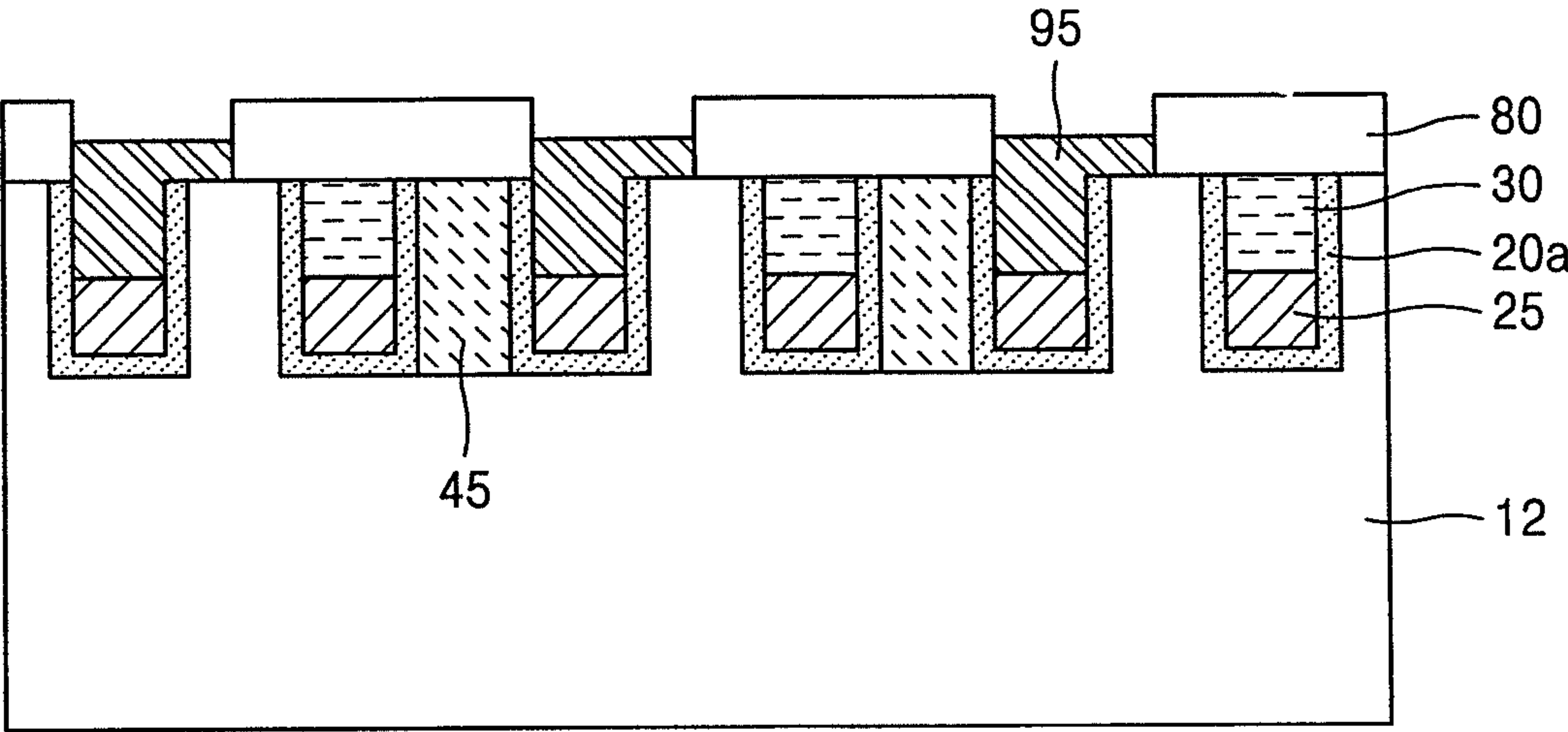
FIG. 20A
