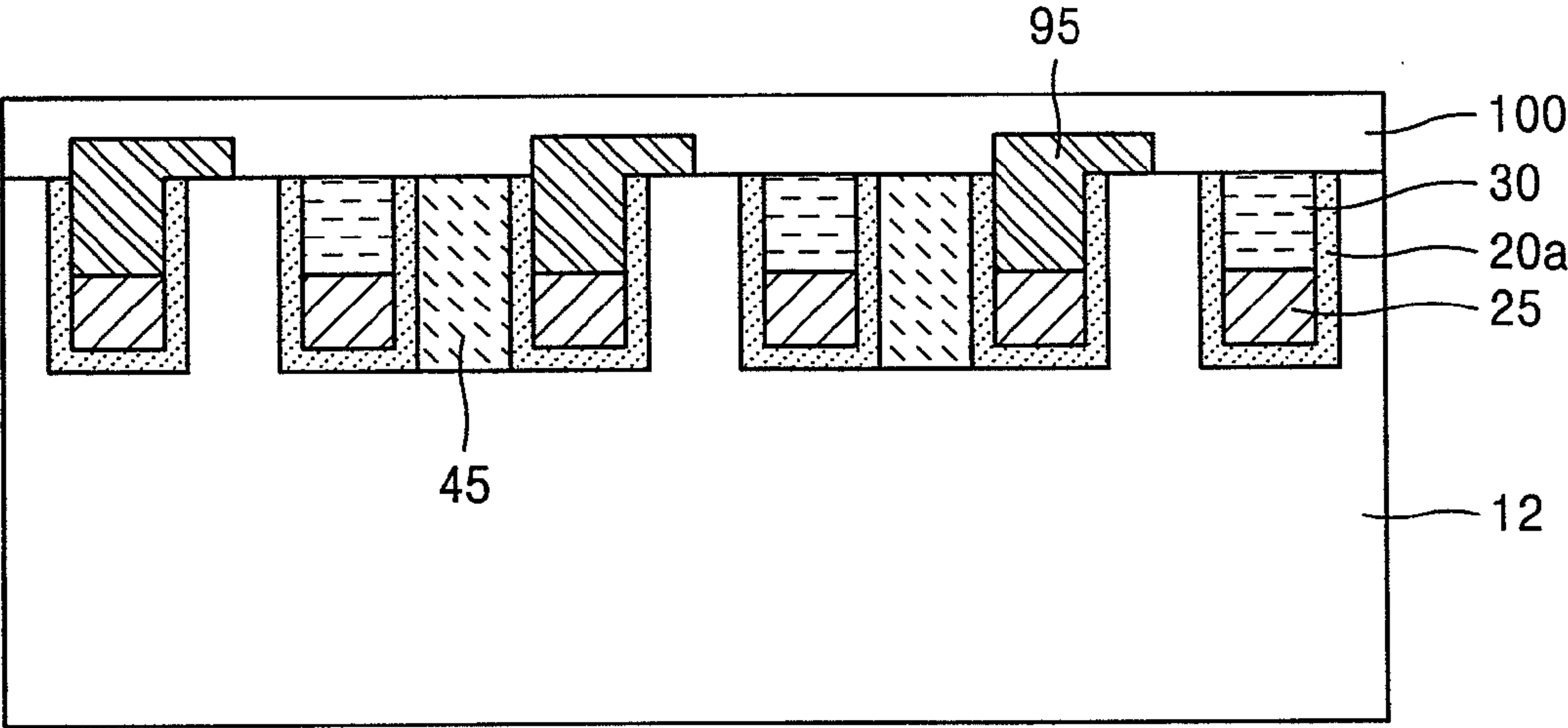
FIG. 21A
