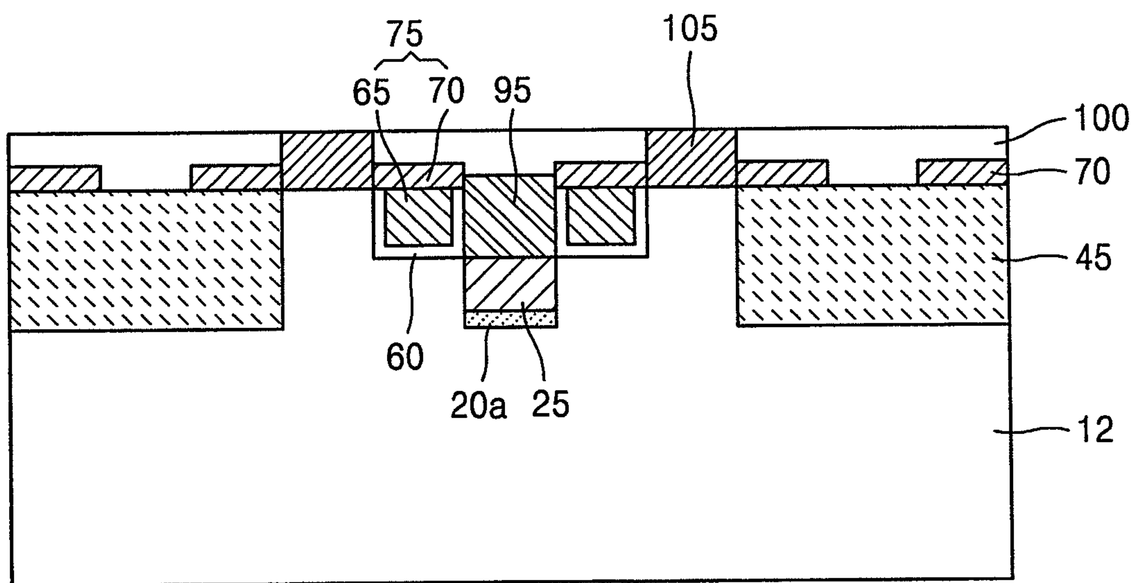
FIG. 23B
