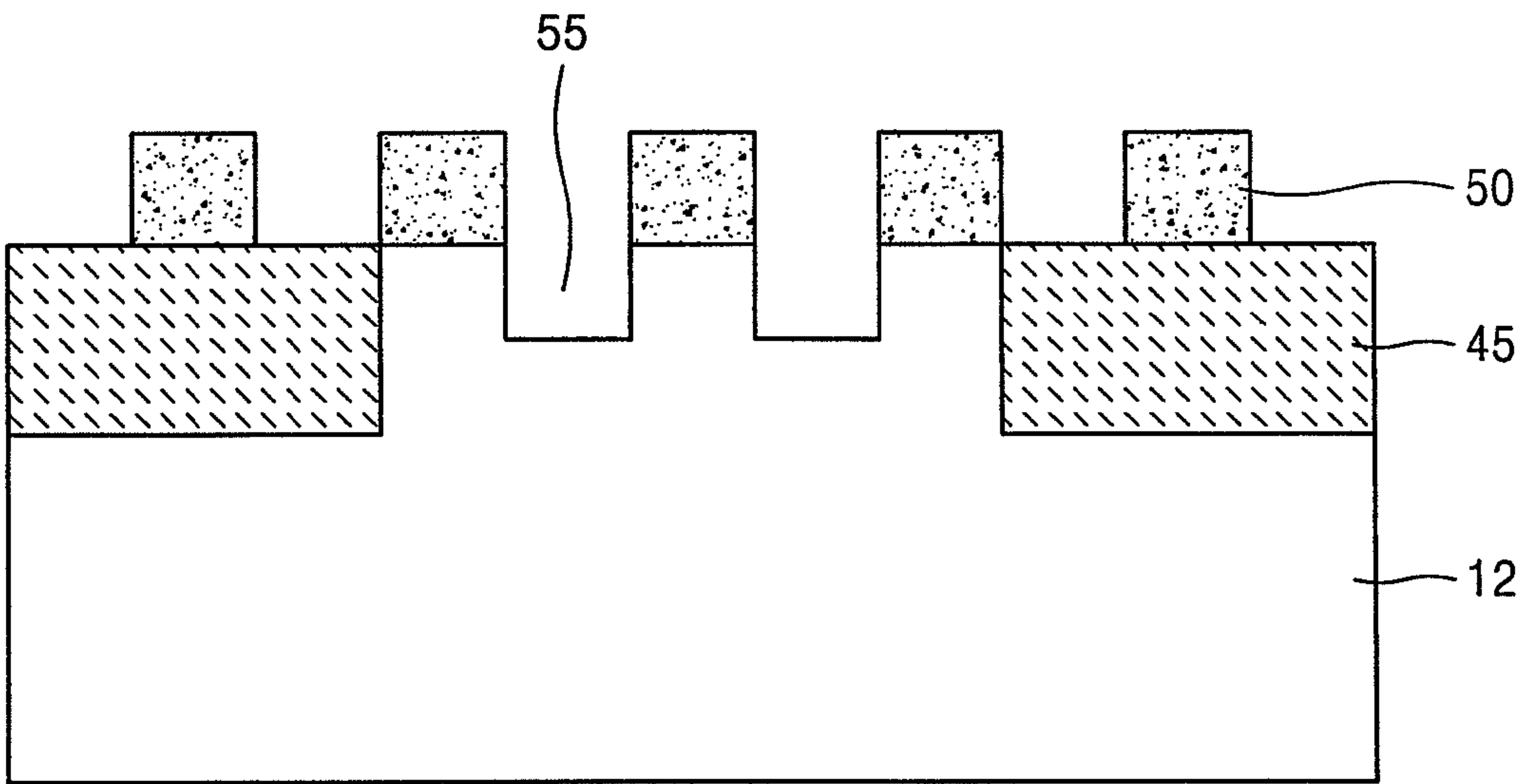
FIG. 15B
