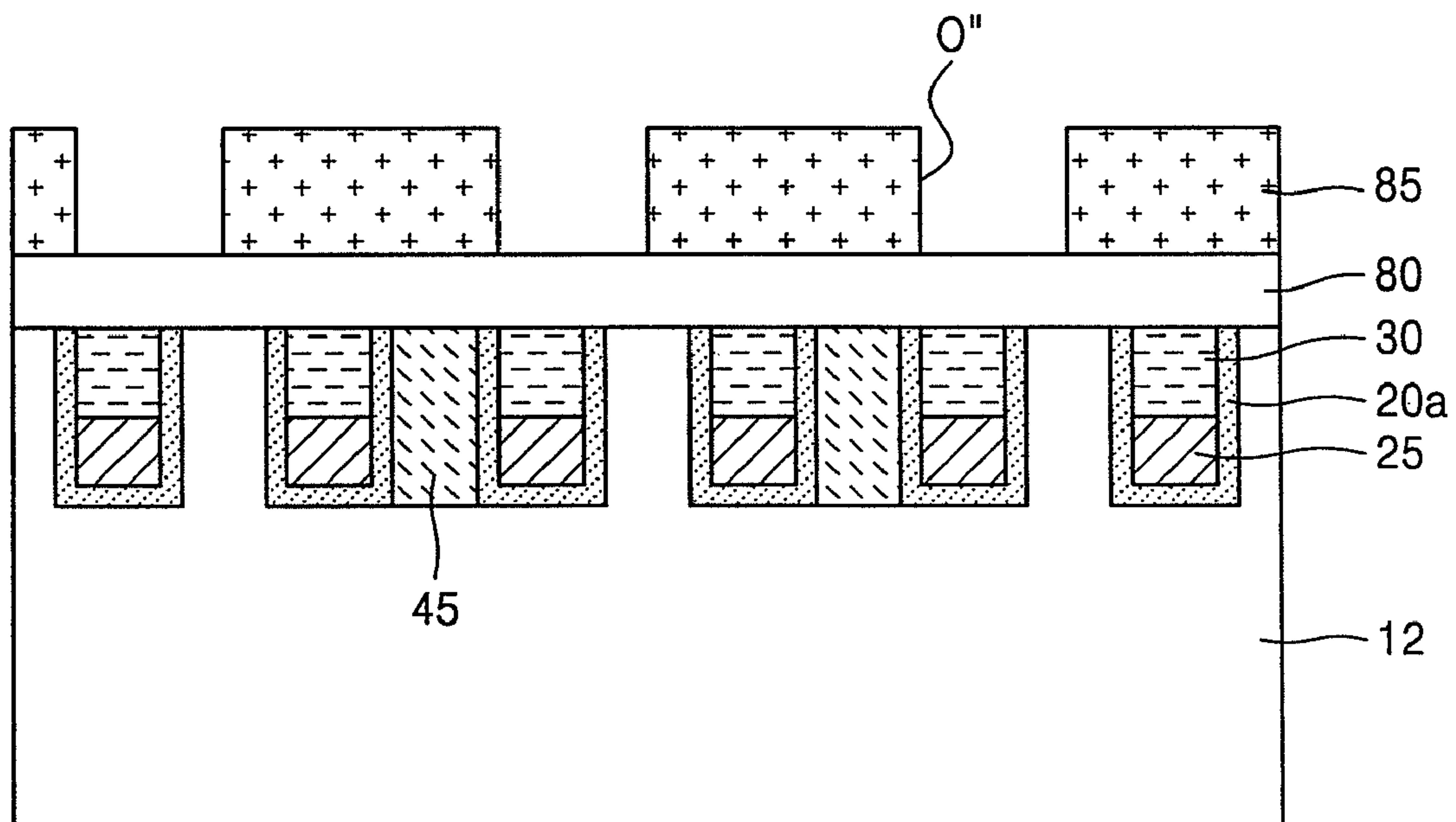
FIG. 18A
