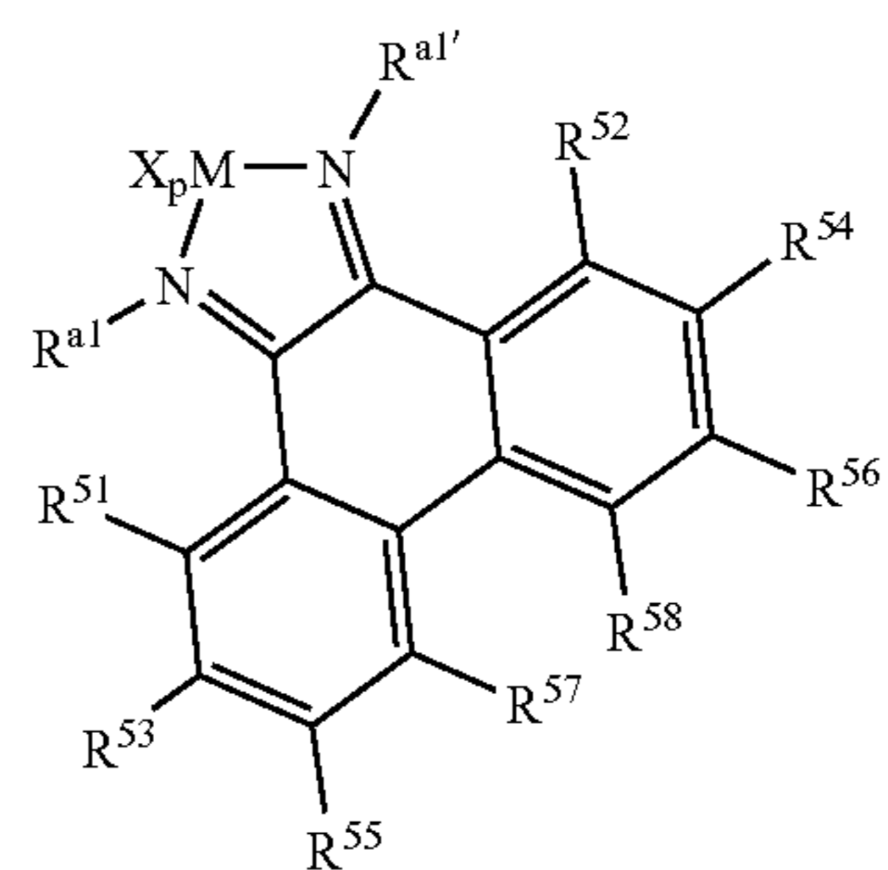
Structure 12e
