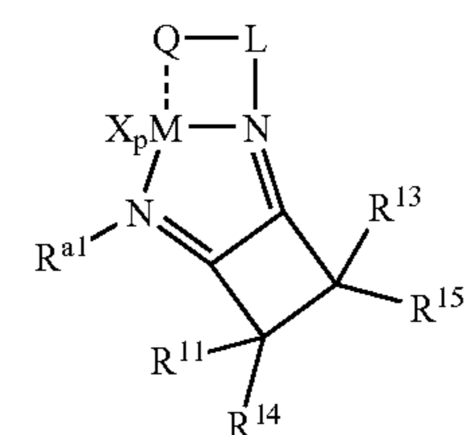
Structure 16e
