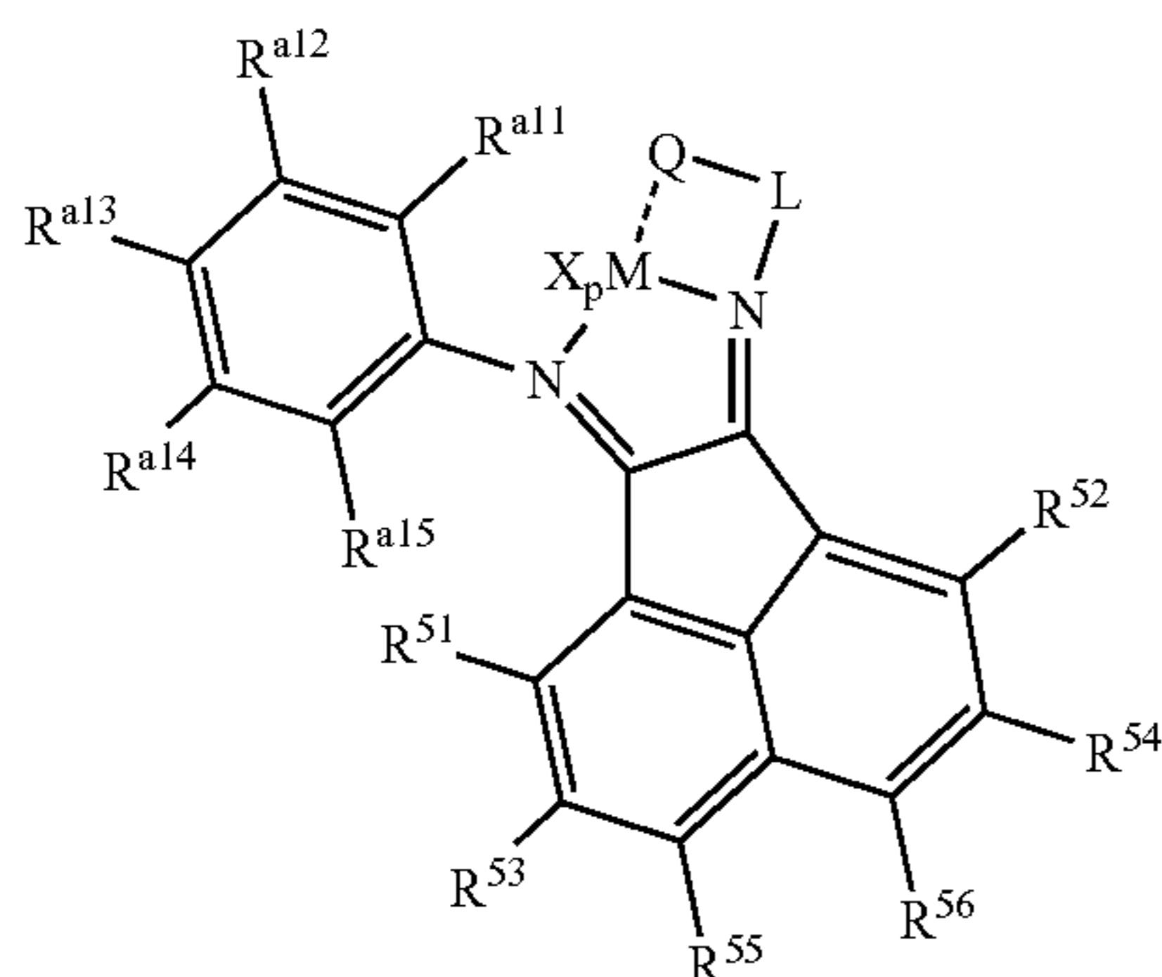
Structure 37e
