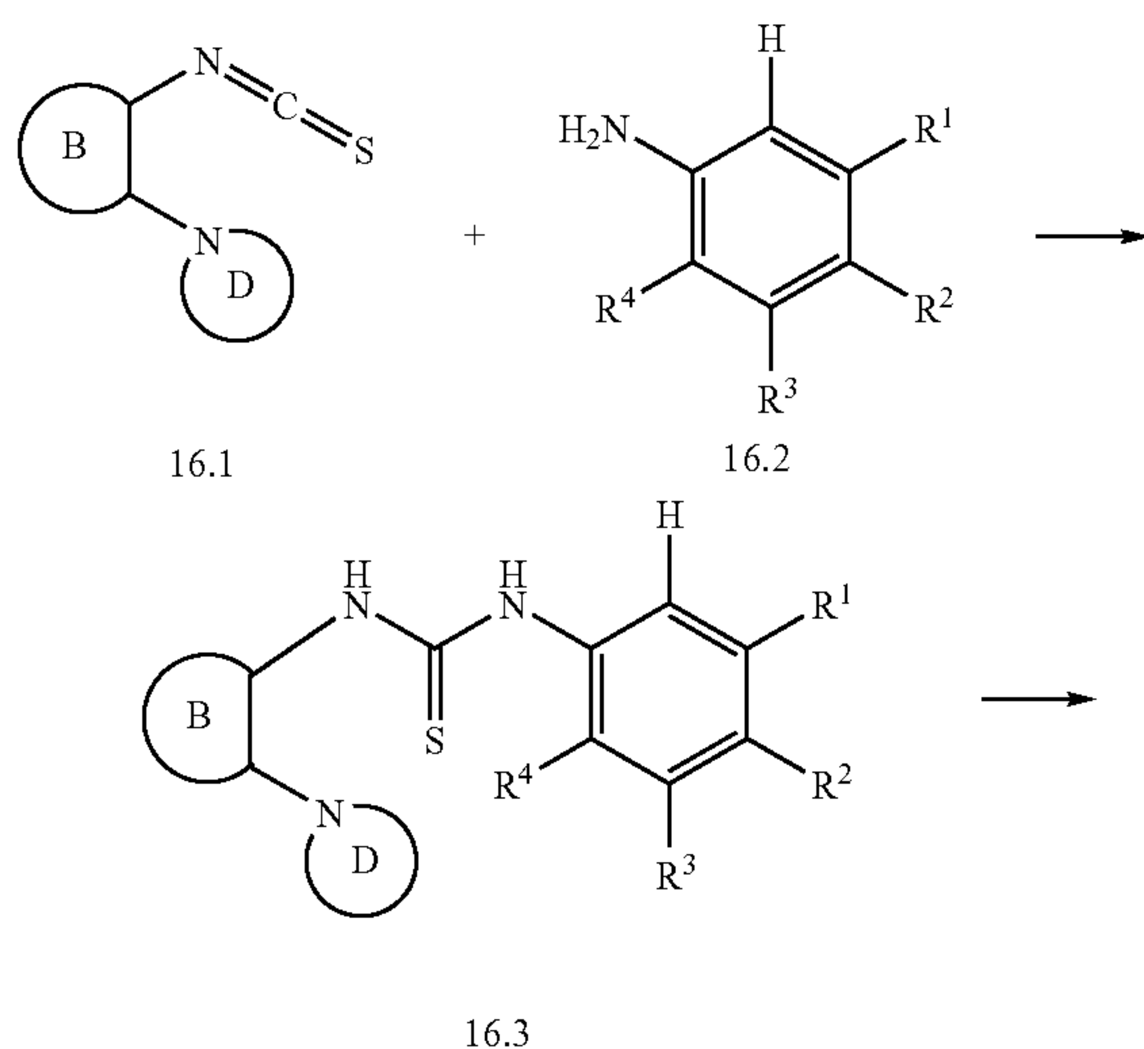
Scheme 16-a
