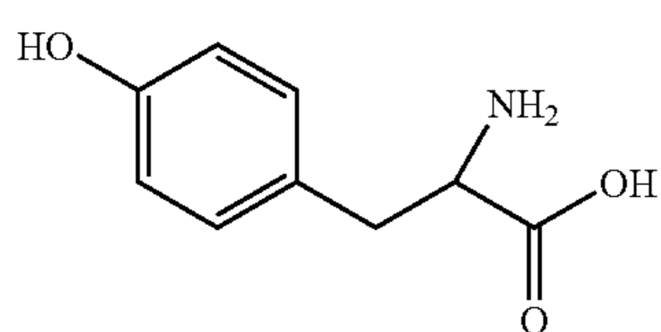
tyrosine
