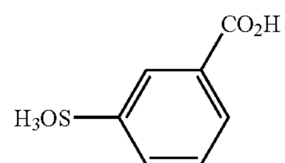
3-sulphonbenzoic acid
