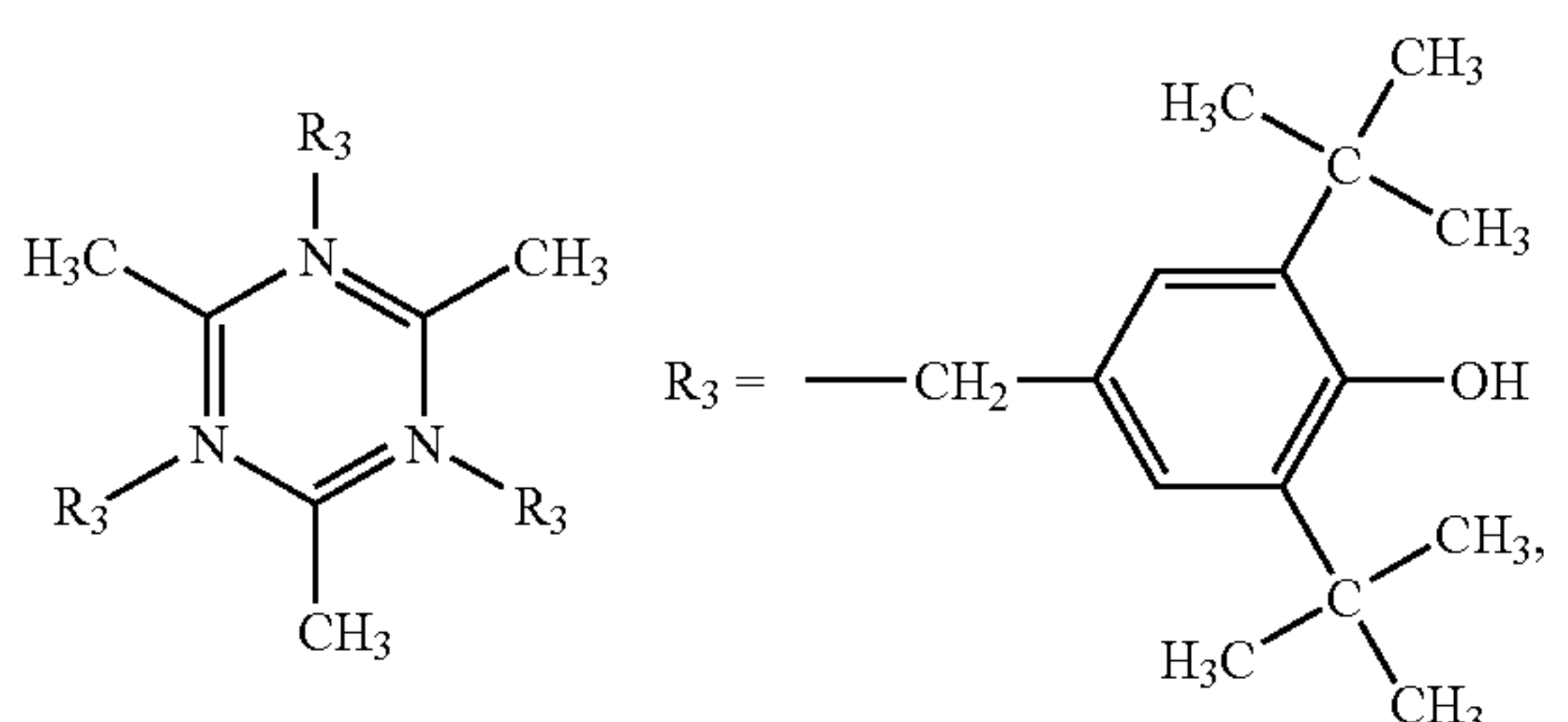
Irganox® 1330.
