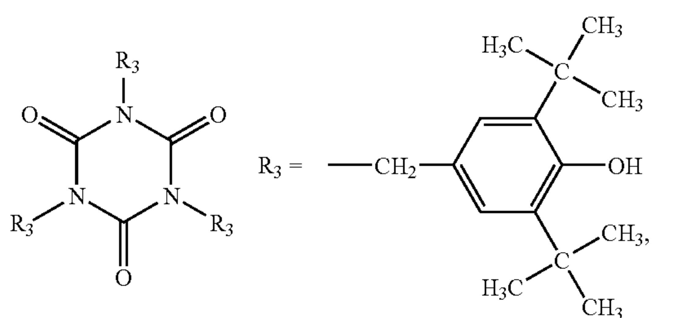
Irganox® 3114
