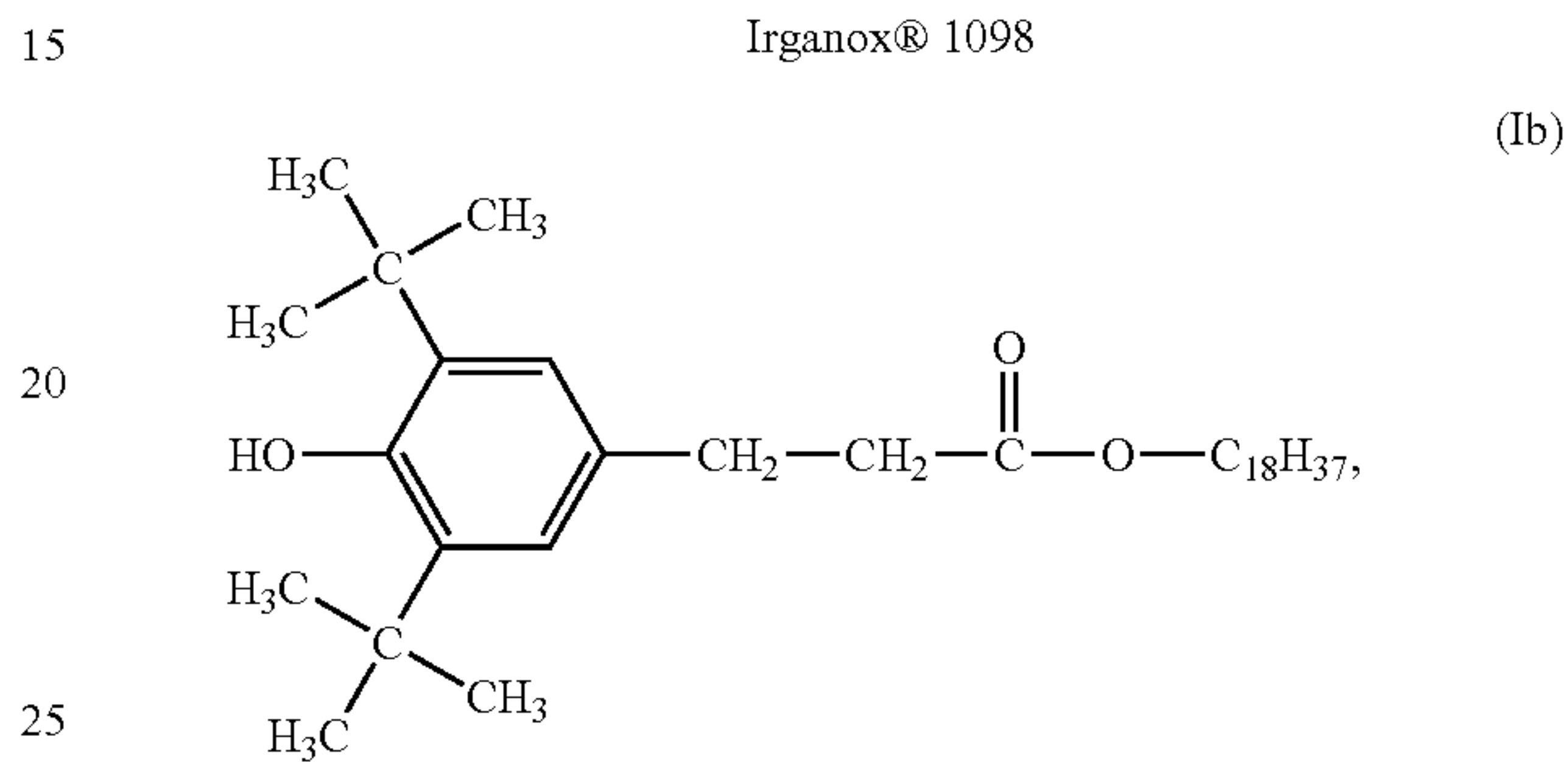
Irganox® 1076
