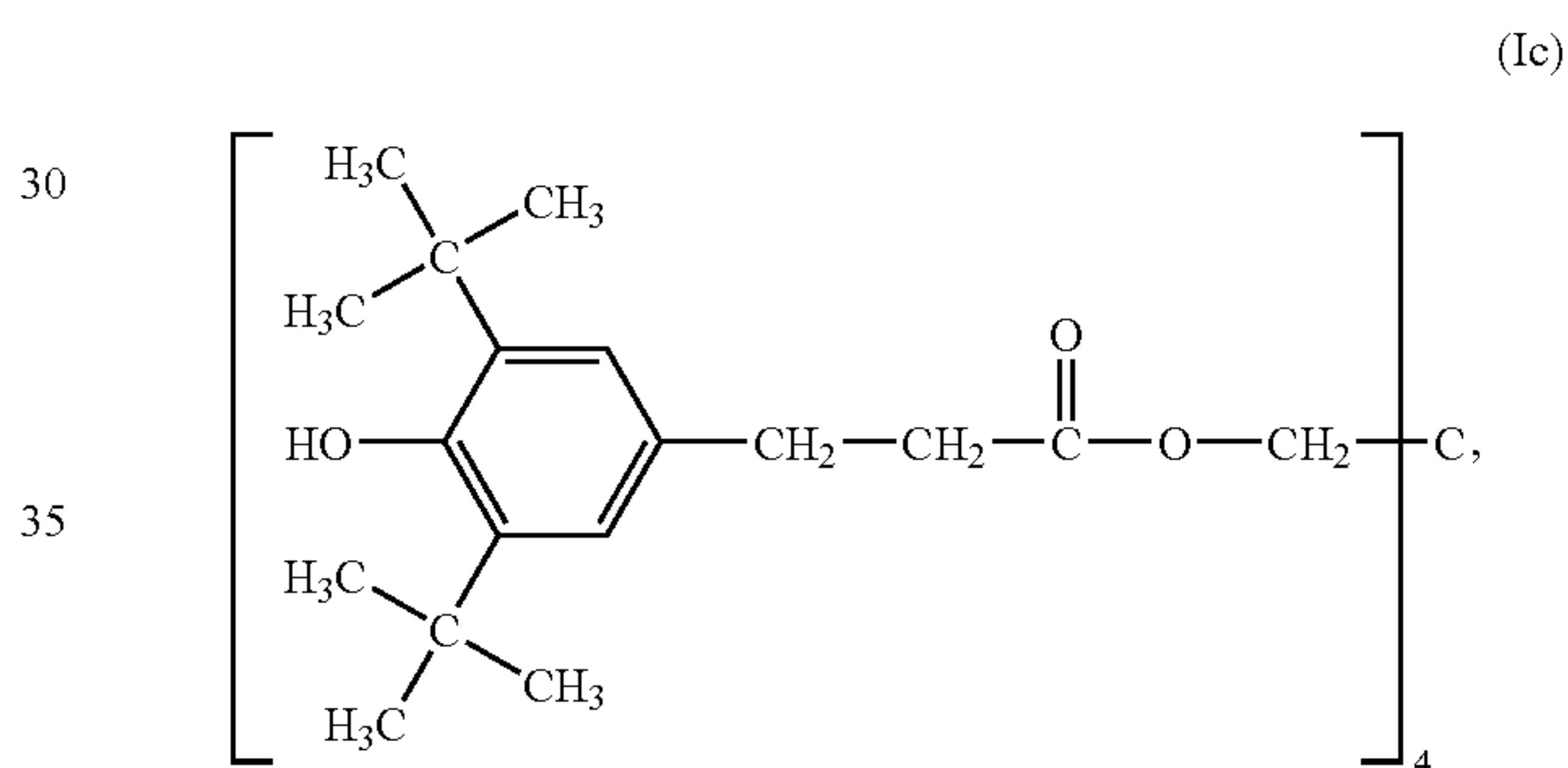
Irganox® 1010
