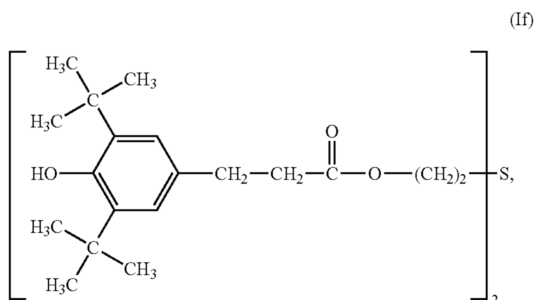
Irganox® 1035
