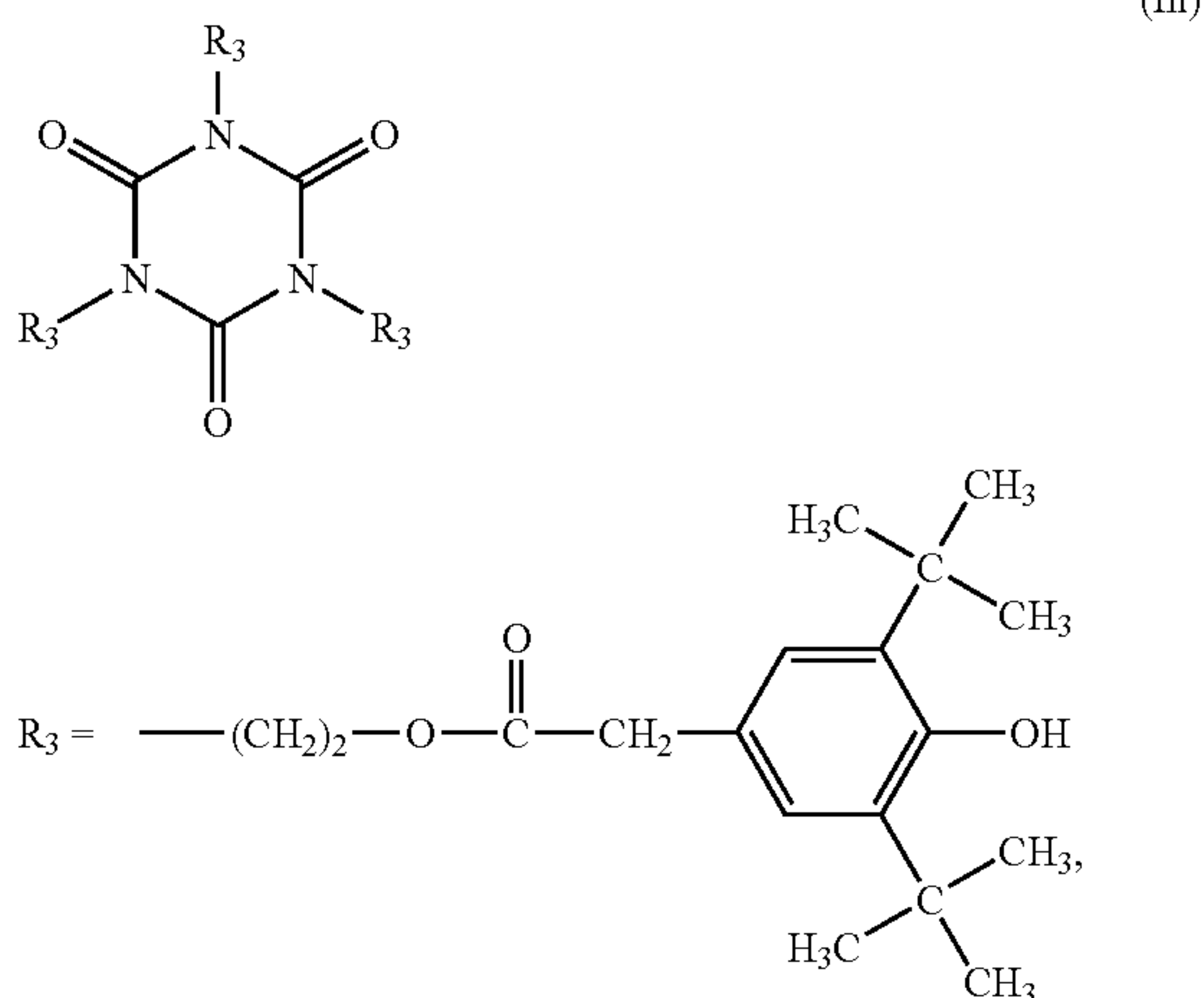
Irganox® 3125.
