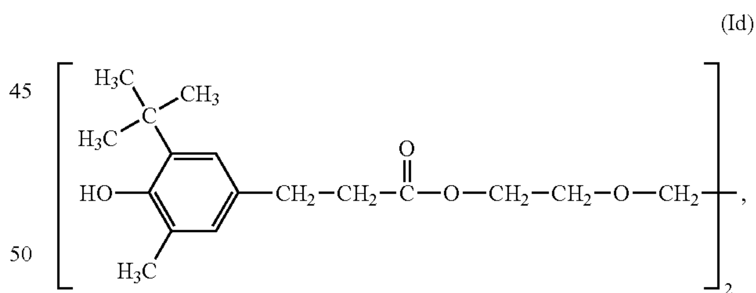
Irganox® 245
