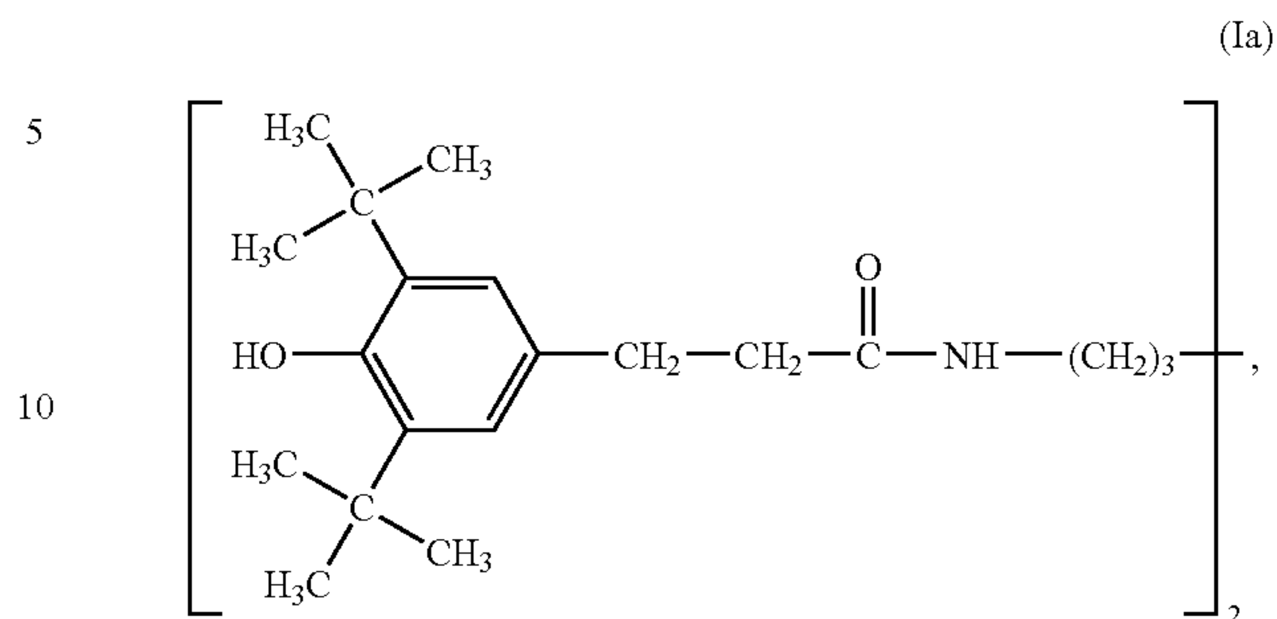
Irganox® 1098
