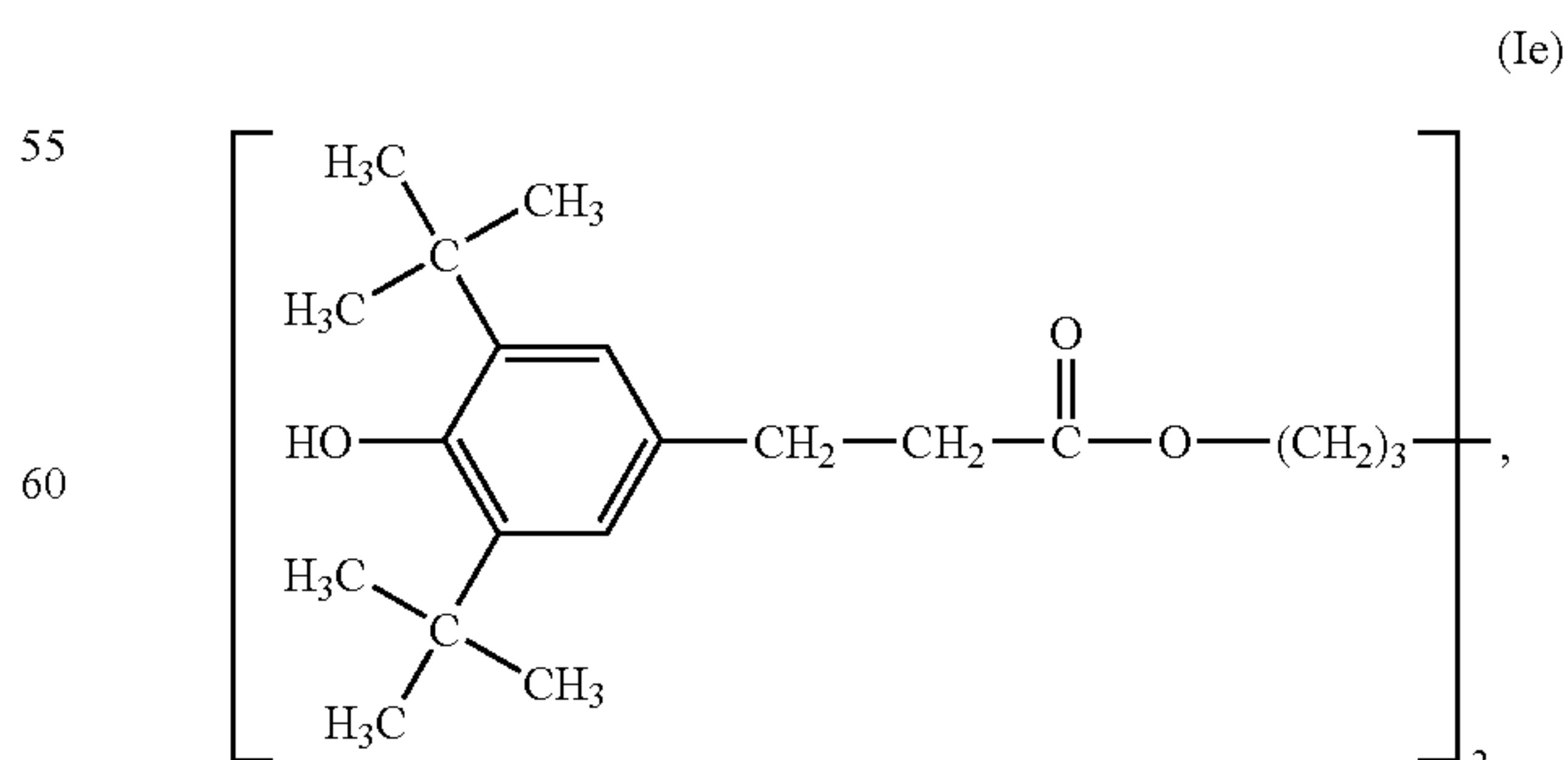
Irganox® 259
