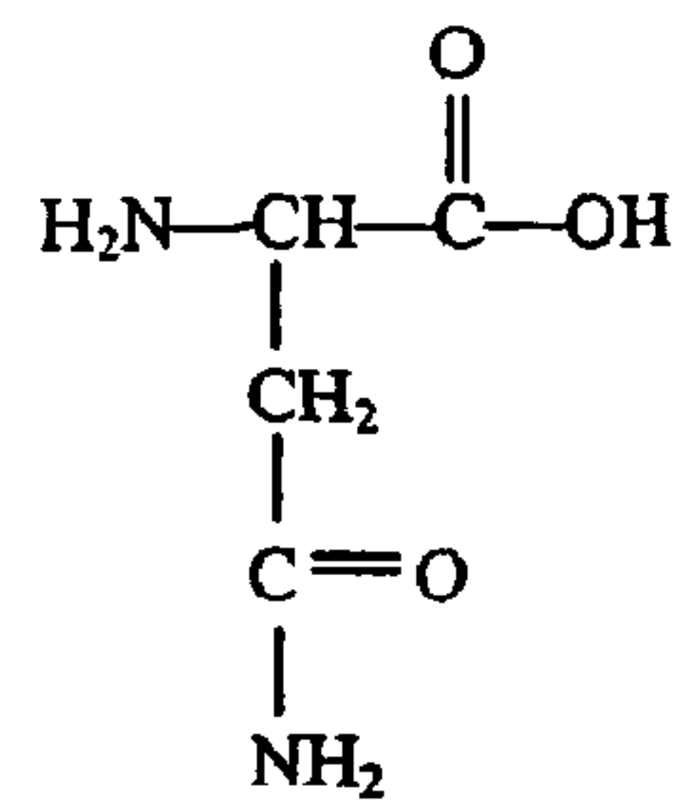
Asparagine (N)
