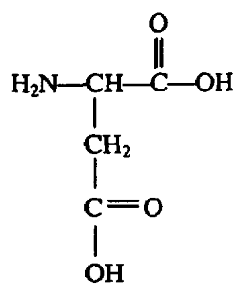
Aspartate (D)
