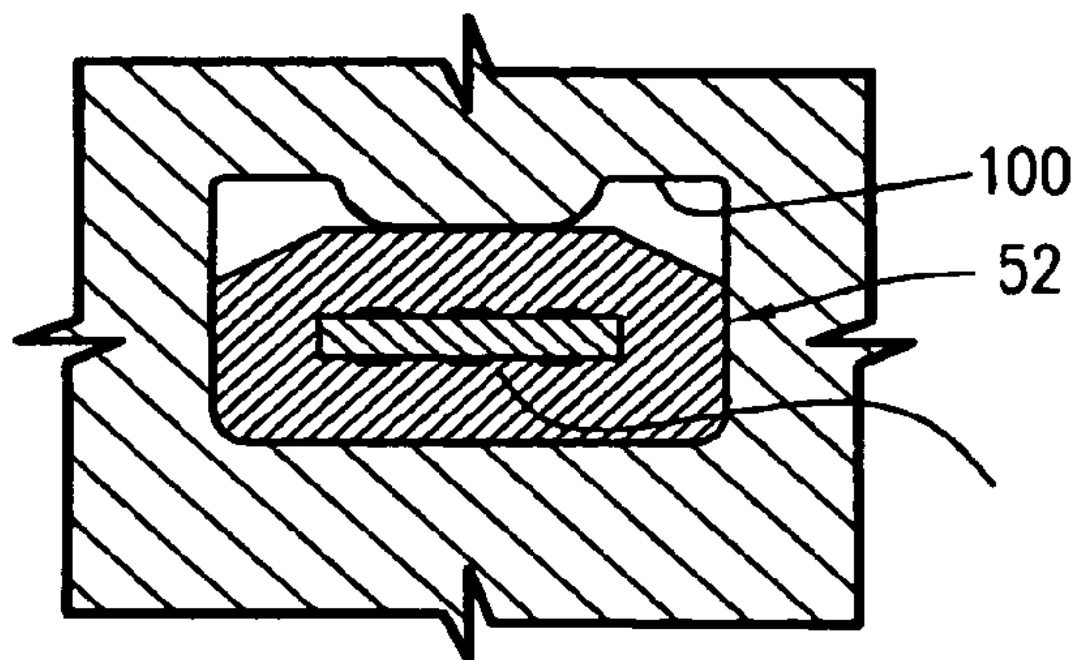
FIG. 18M PLUG
