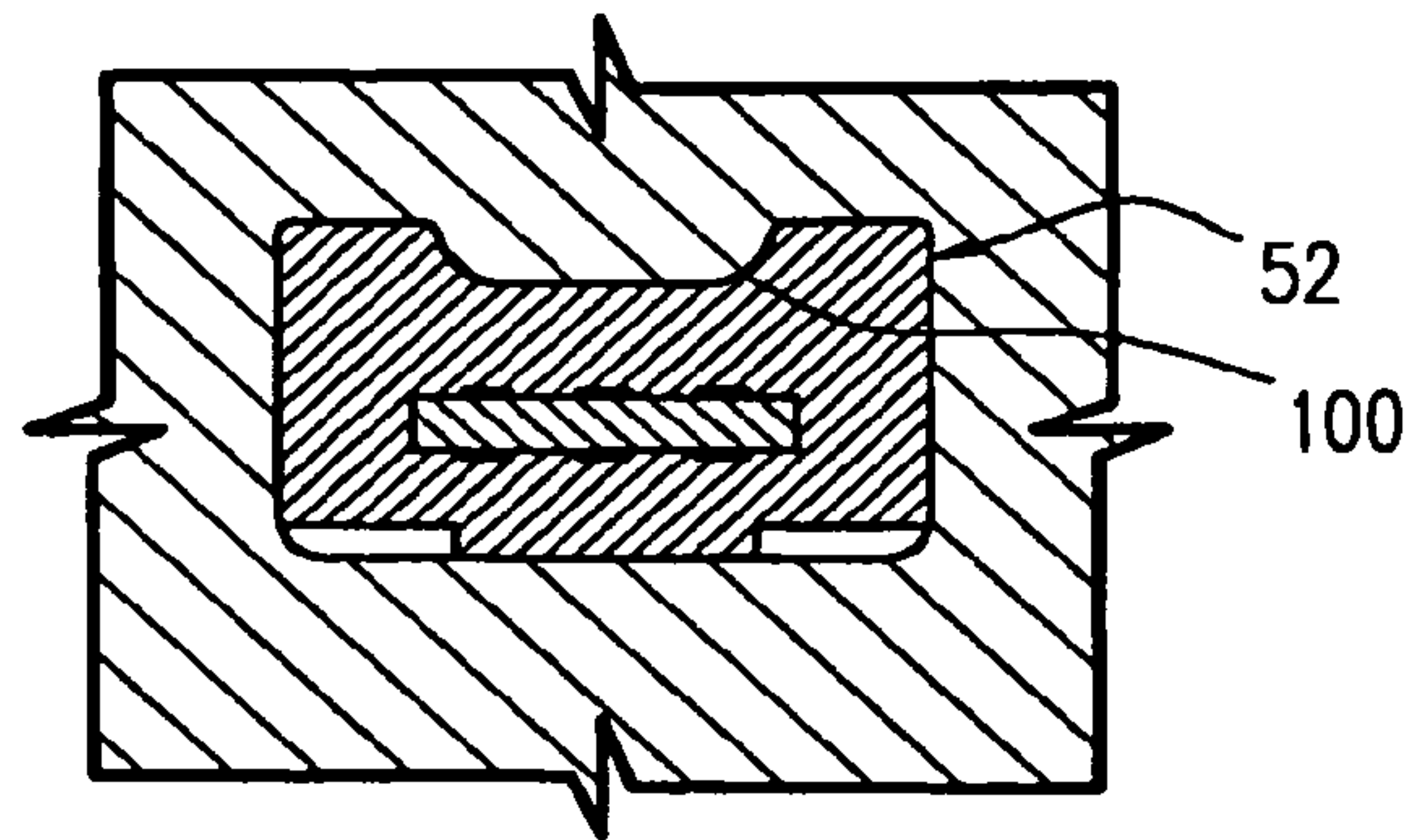
FIG. 18E PLUG
