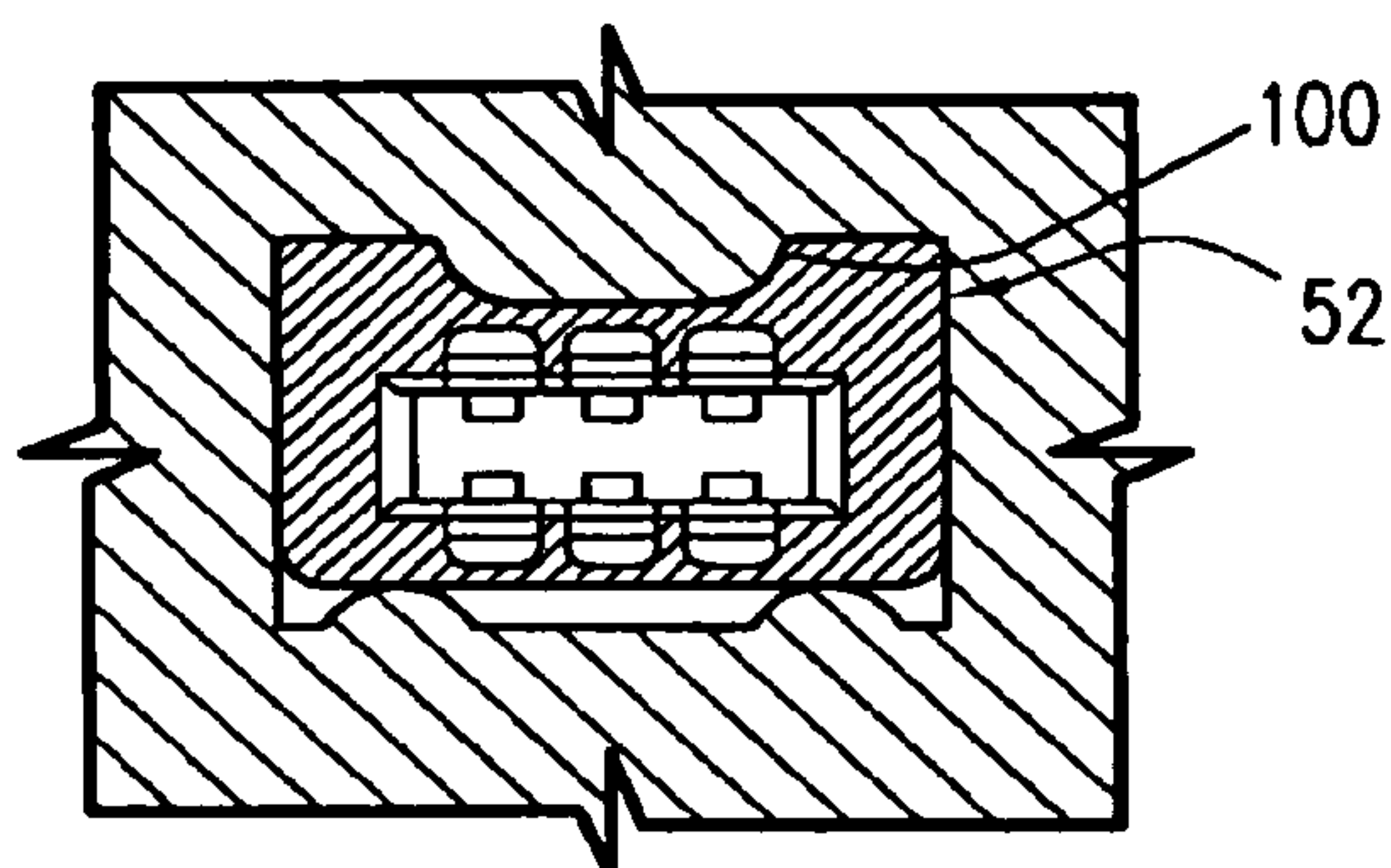
FIG. 17C SOCKET
