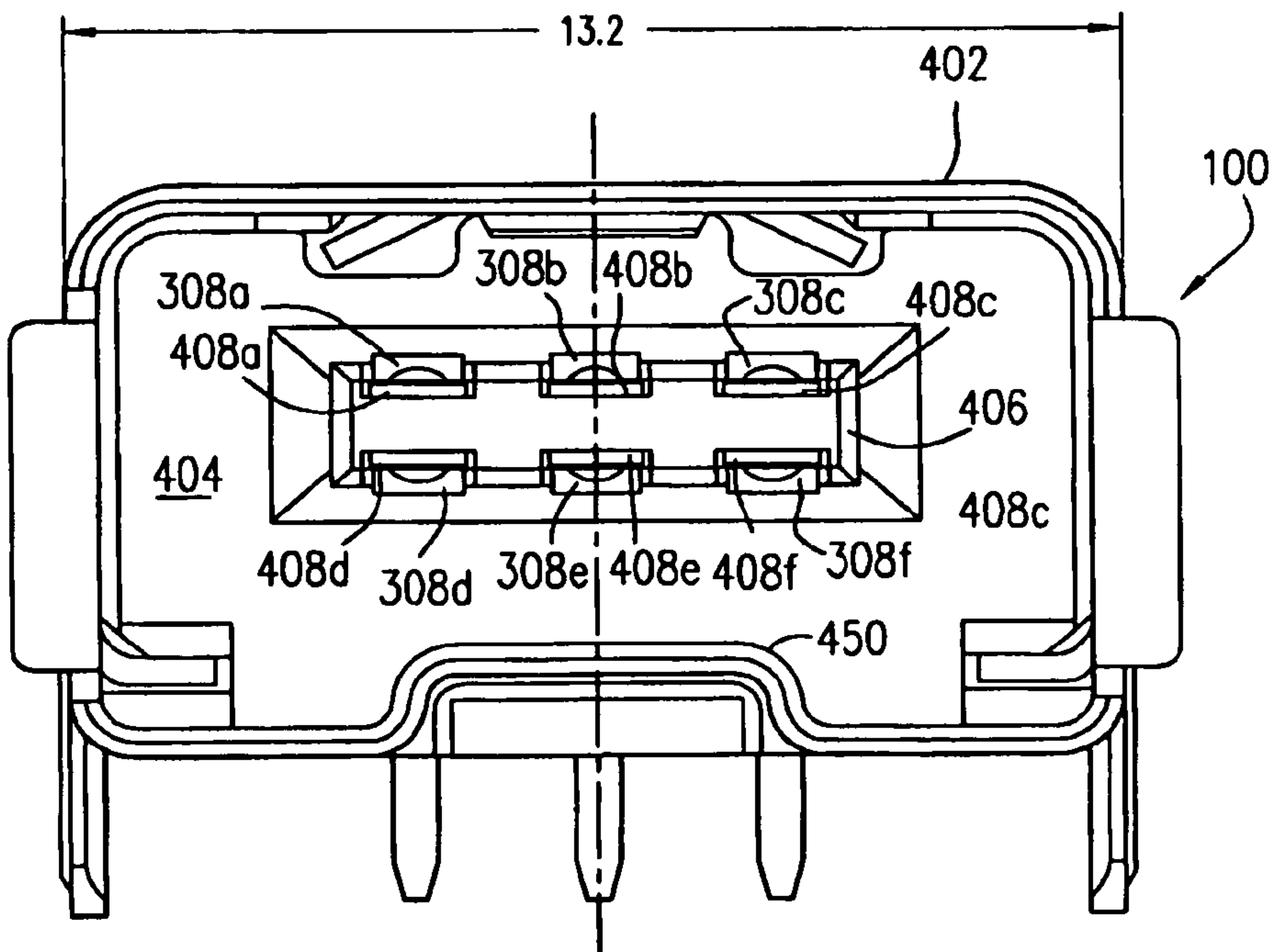
FIG. 12 SOCKET
