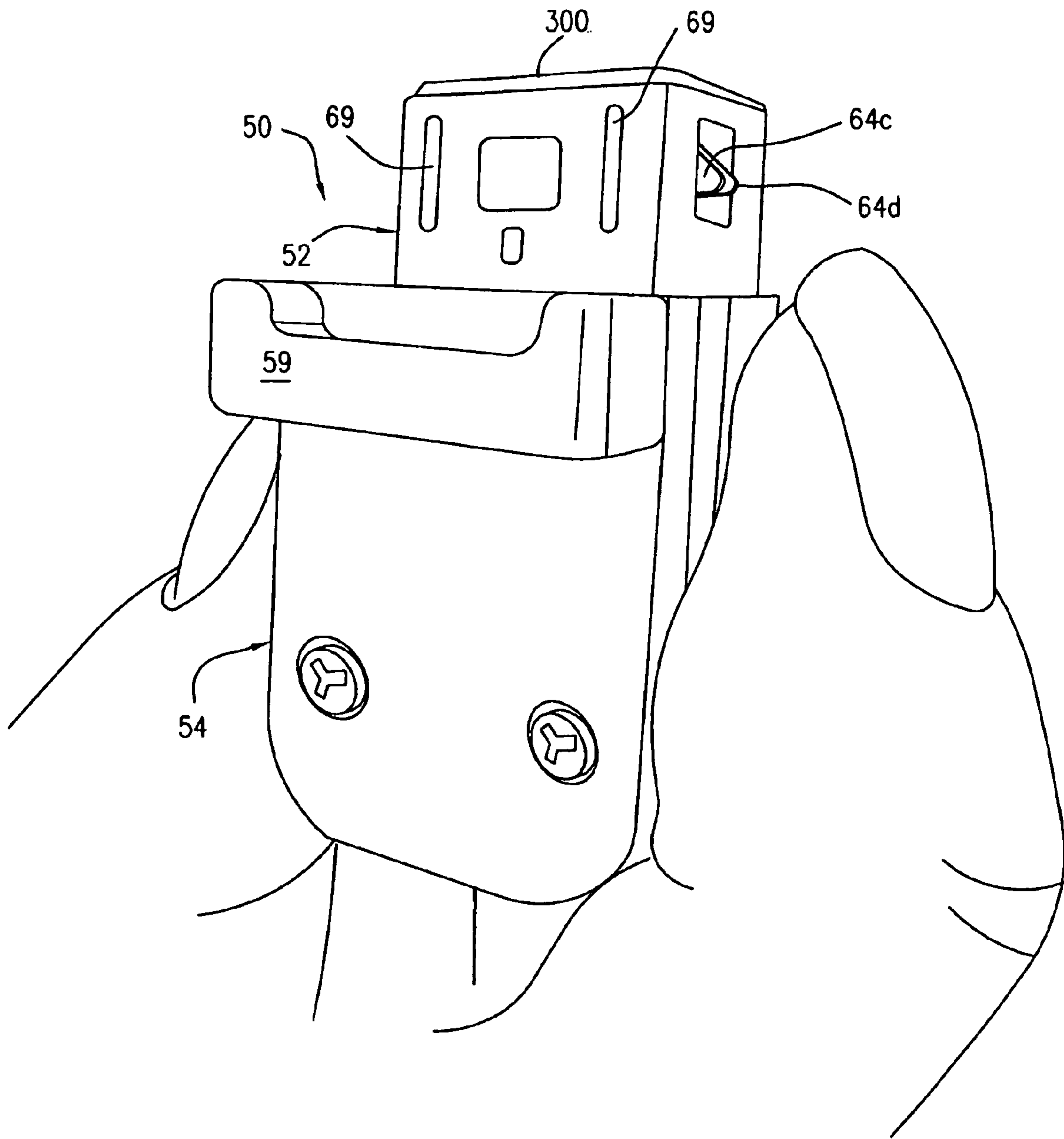
FIG. 2B PLUG
