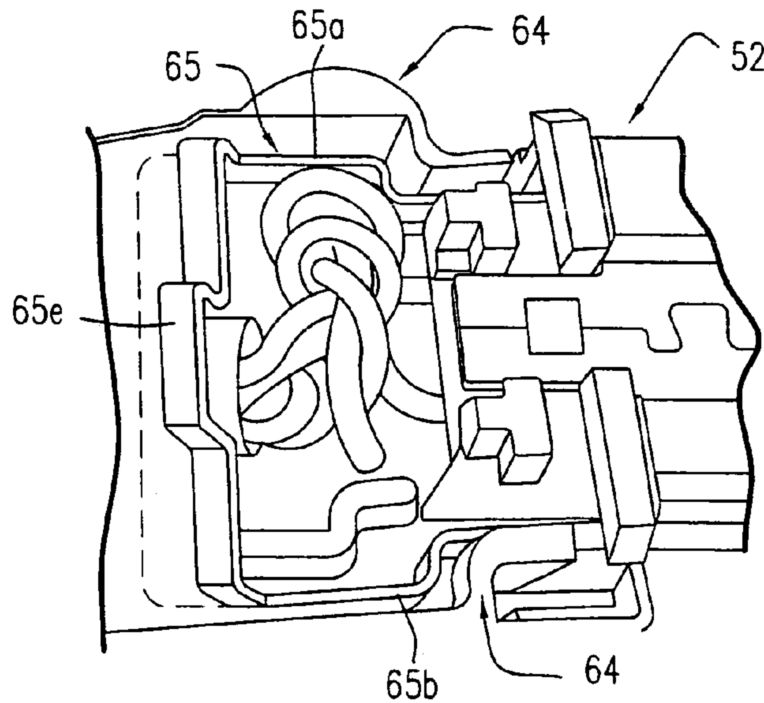
FIG. 8A PLUG
