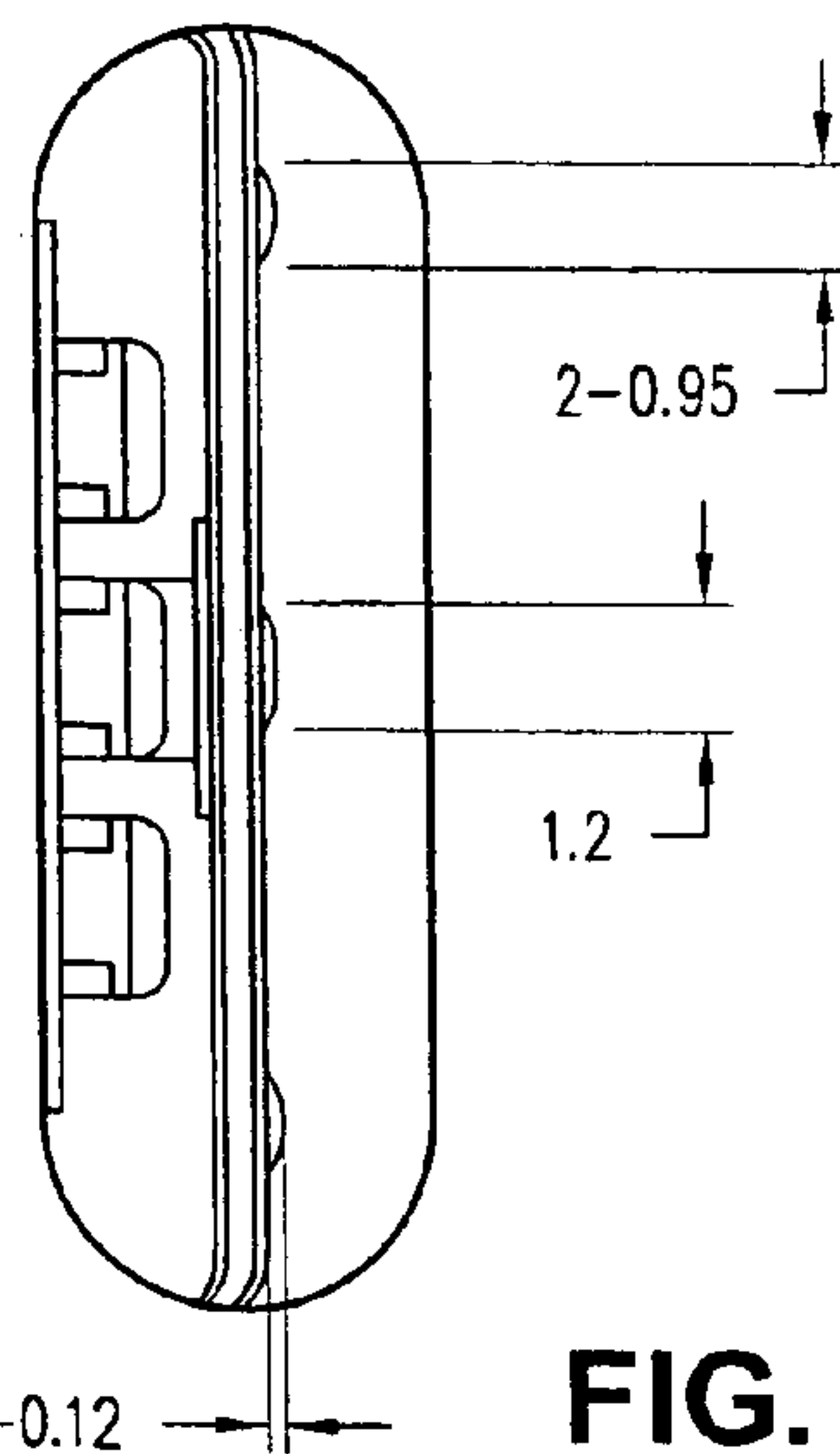
FIG. 8A PLUG
