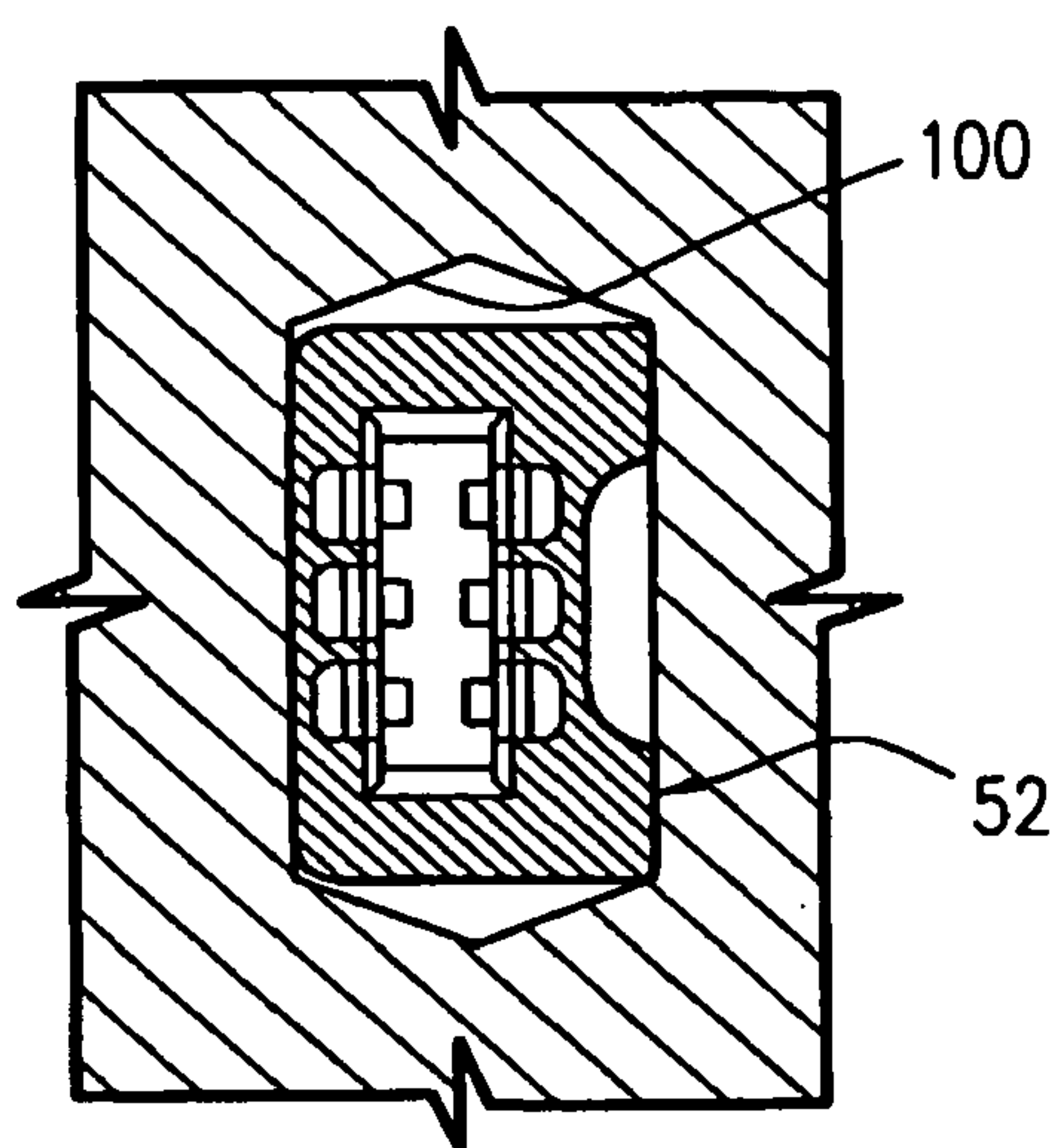
FIG. 17K SOCKET
