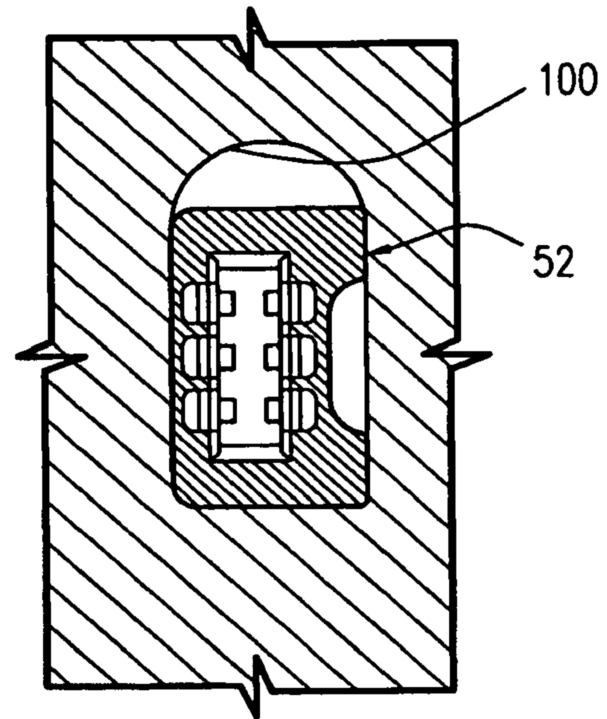
FIG. 17J SOCKET
