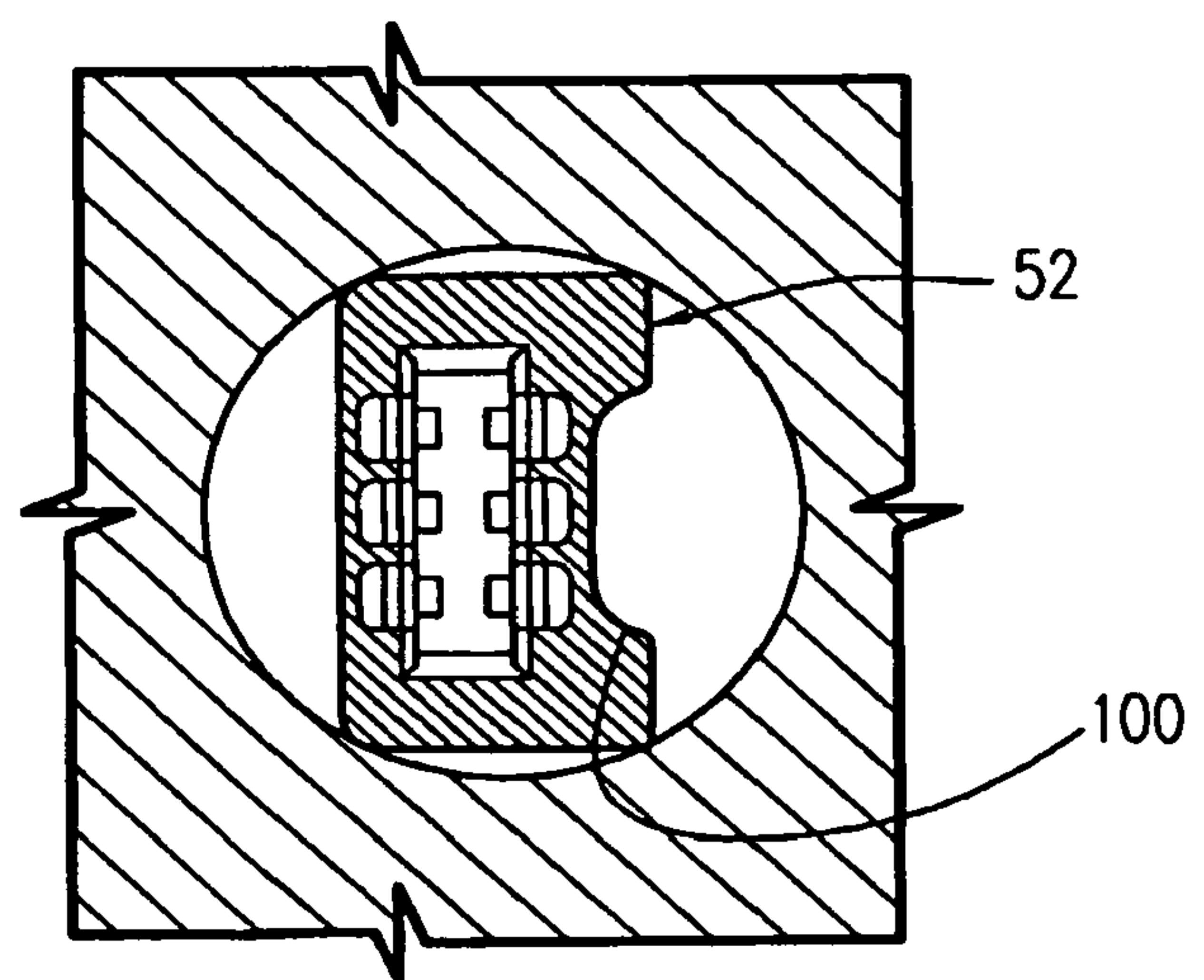
FIG. 17L SOCKET
