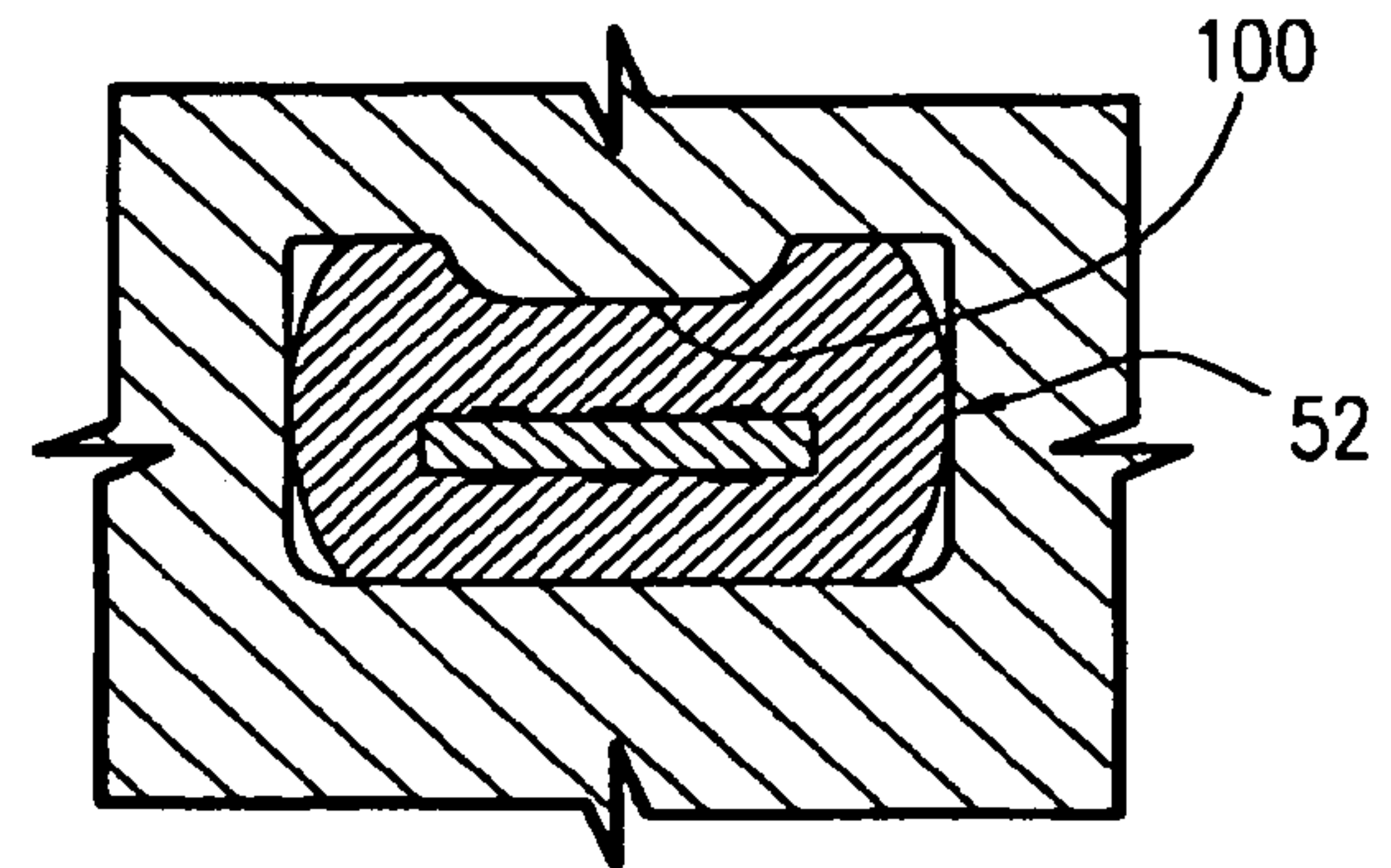
FIG. 18F PLUG
