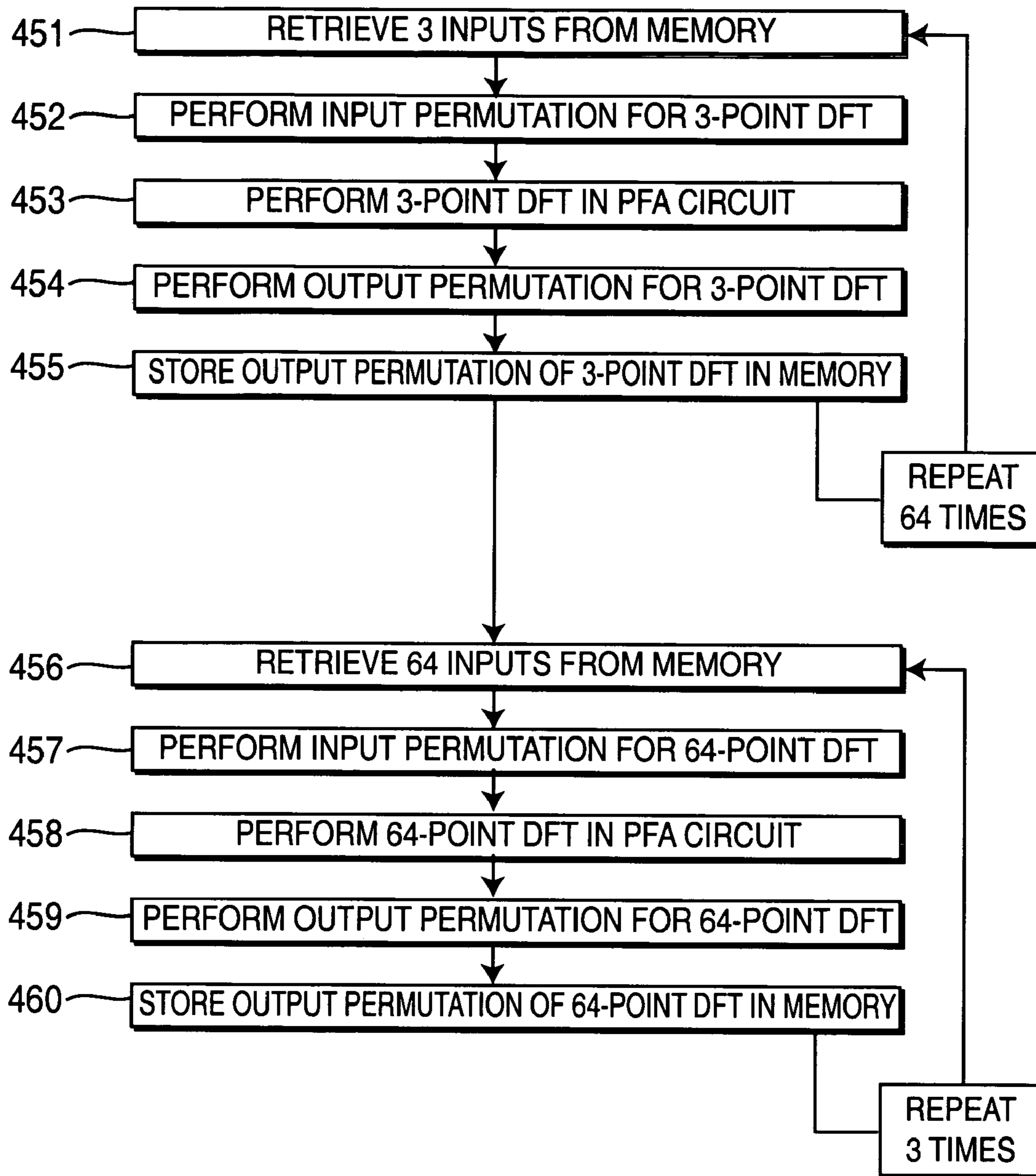
192 POINT DFT USING PFA
