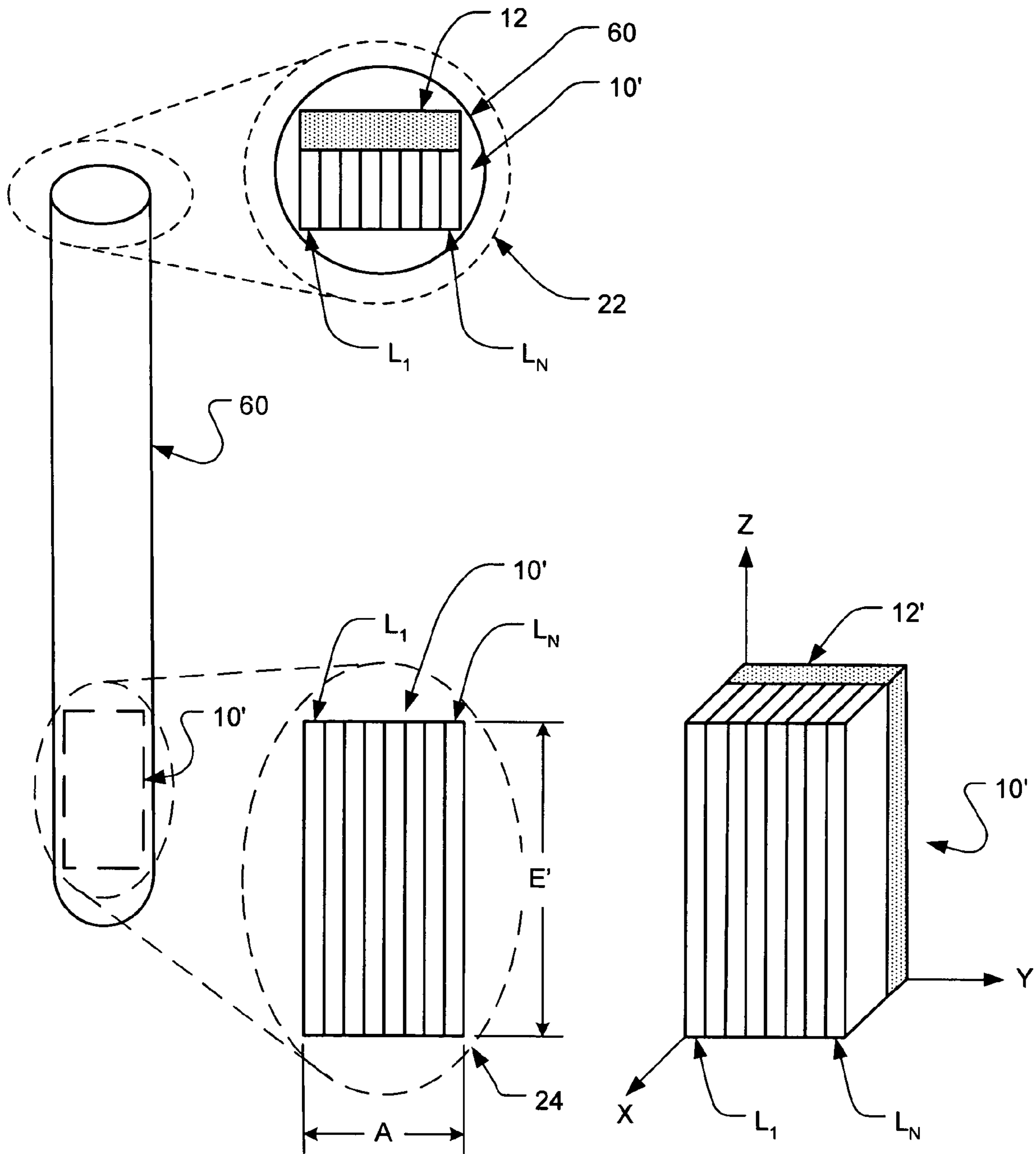
FIG. 8A
