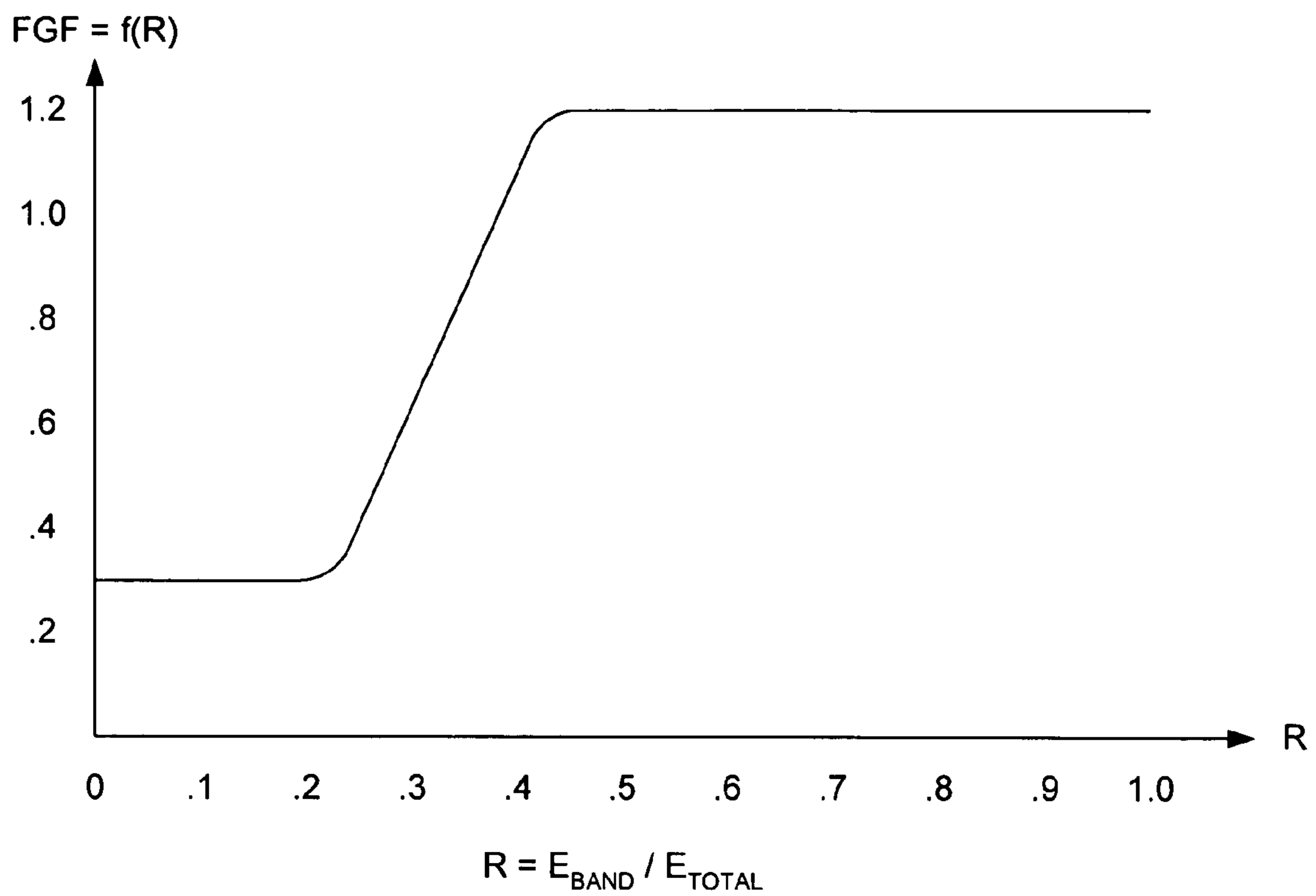
FIG. 15
