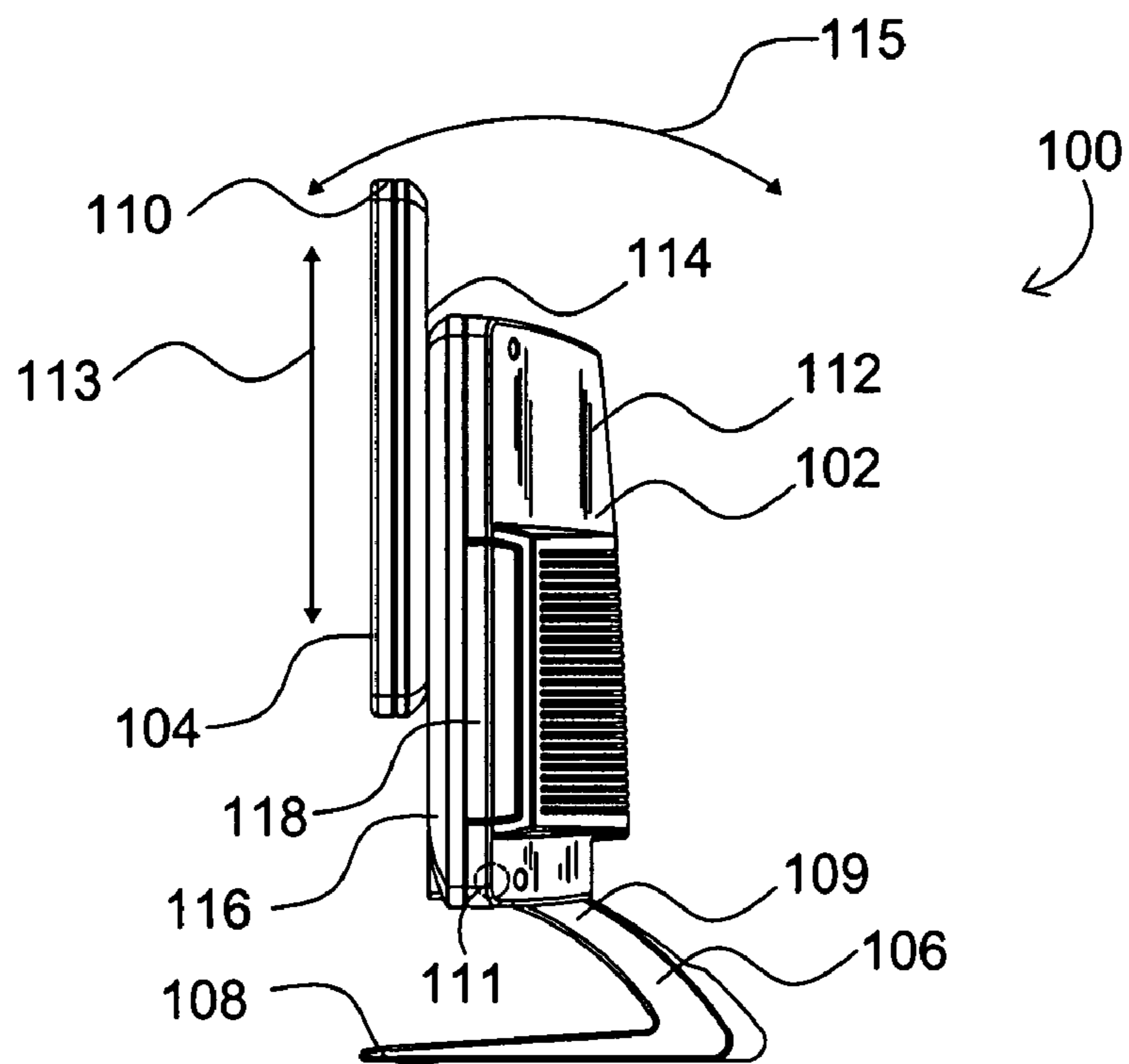
FIG. 2A
