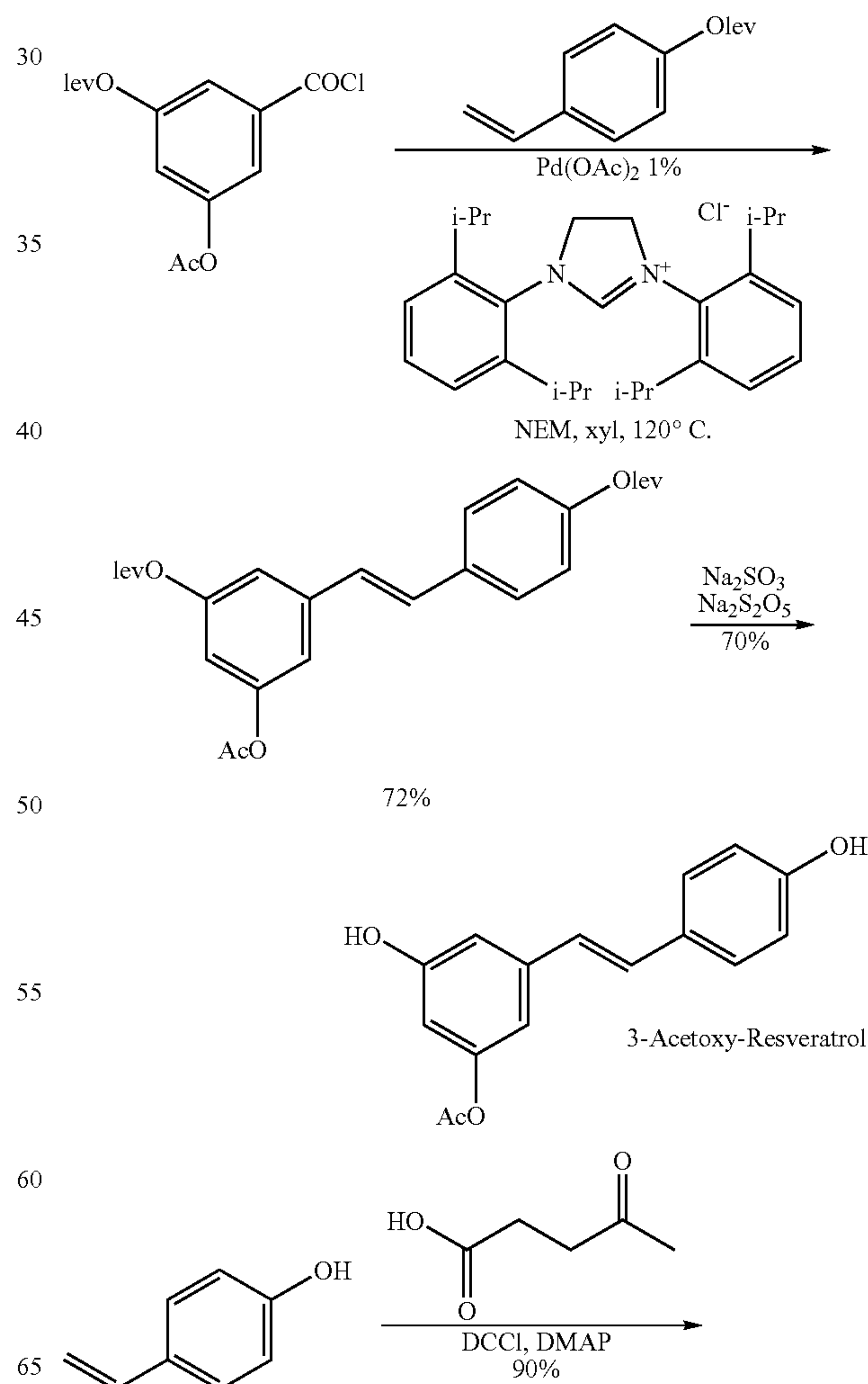
Scheme 14.
