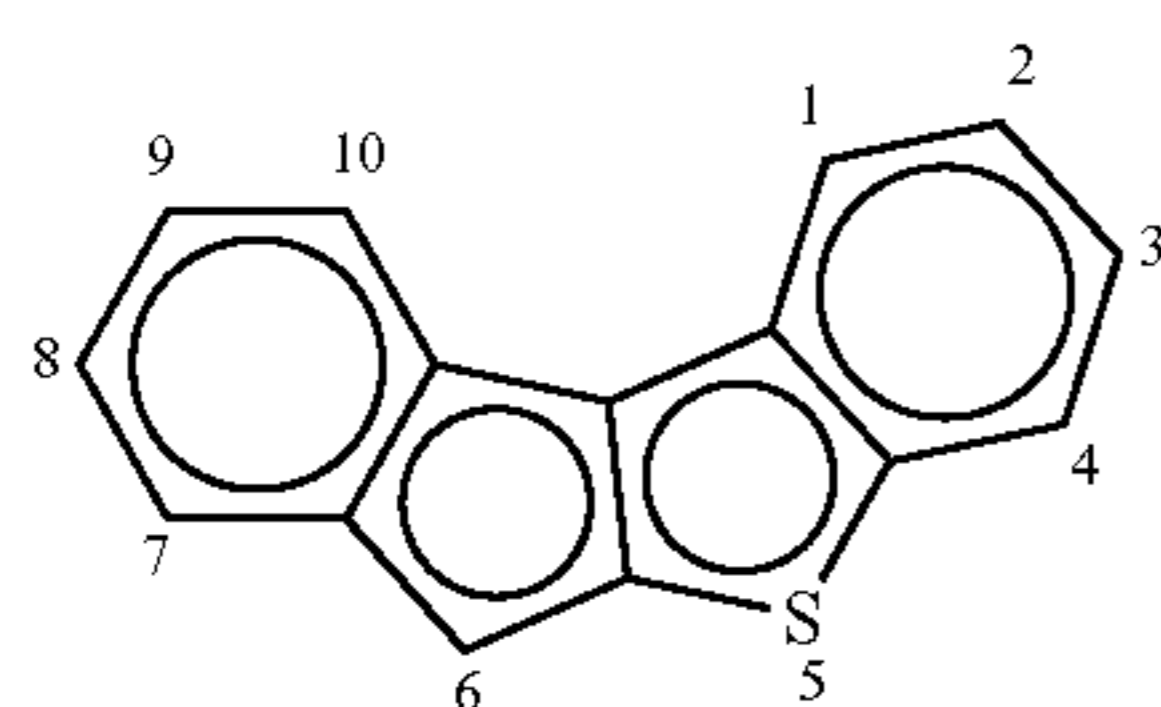
indeno[2,1-b][1]benzothieryl
