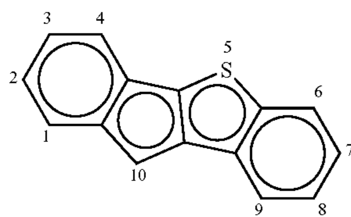
indeno[1,2-b][1]benzothieryl
