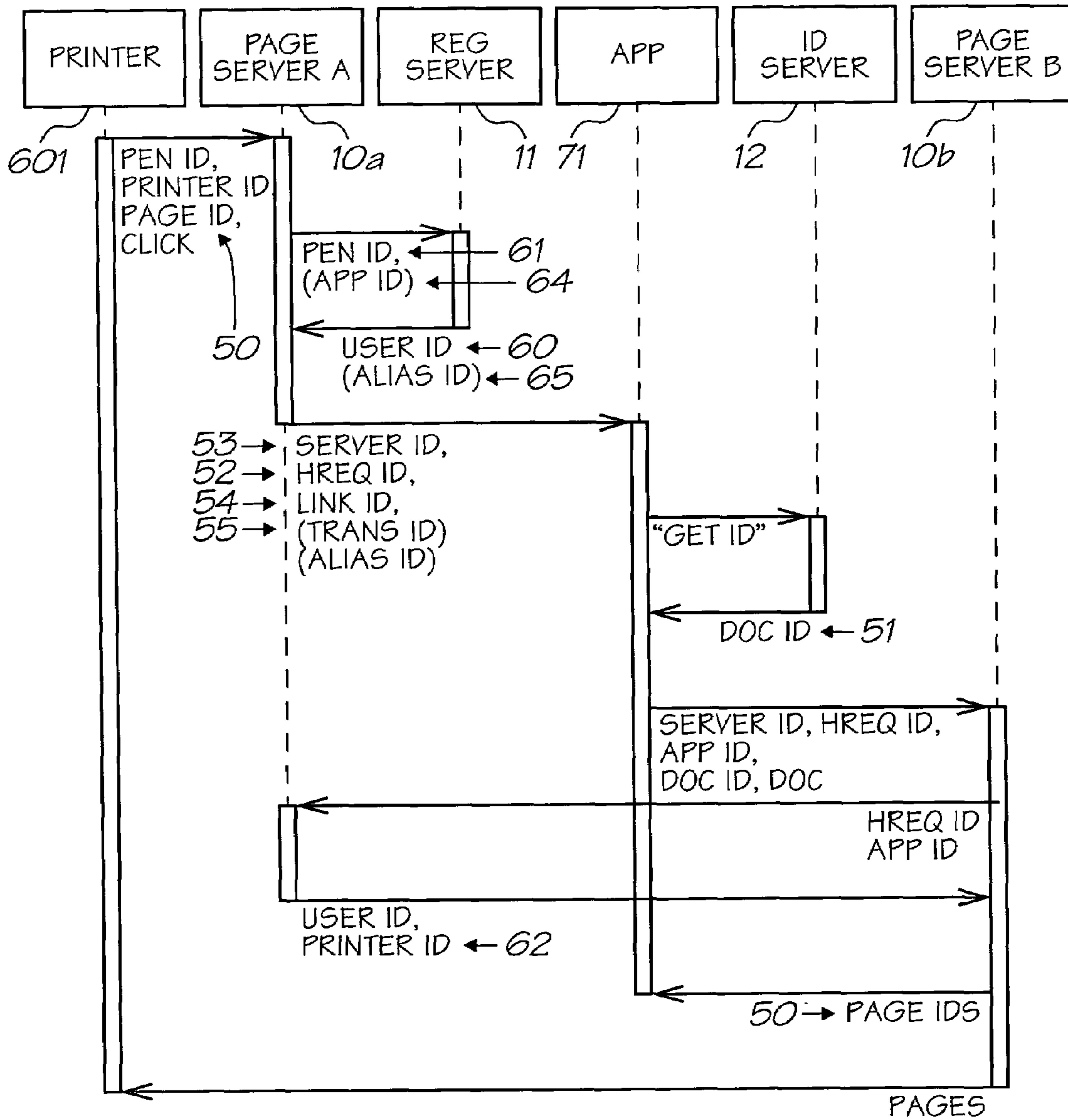
FIG. 45
