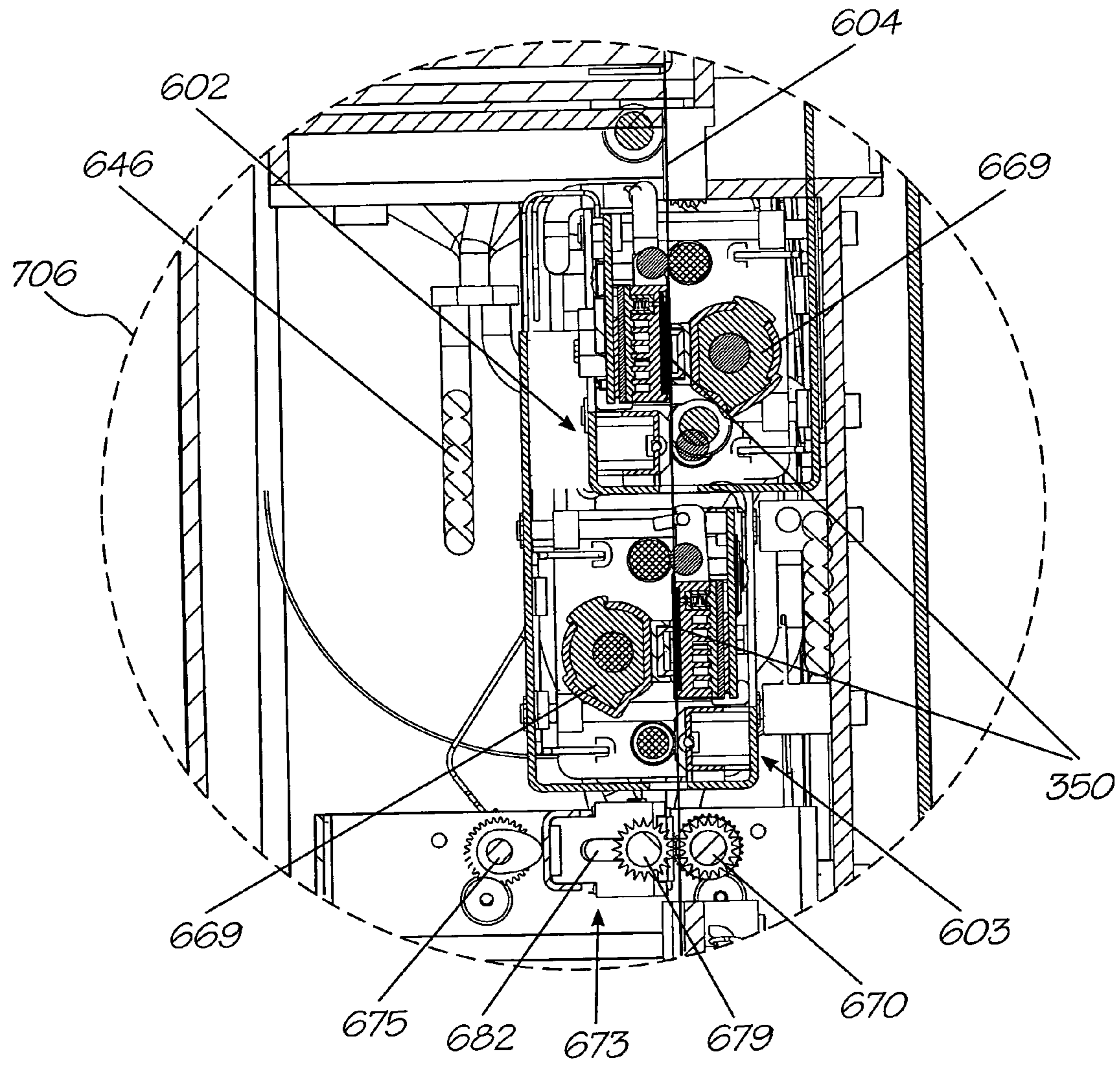
FIG. 12a
