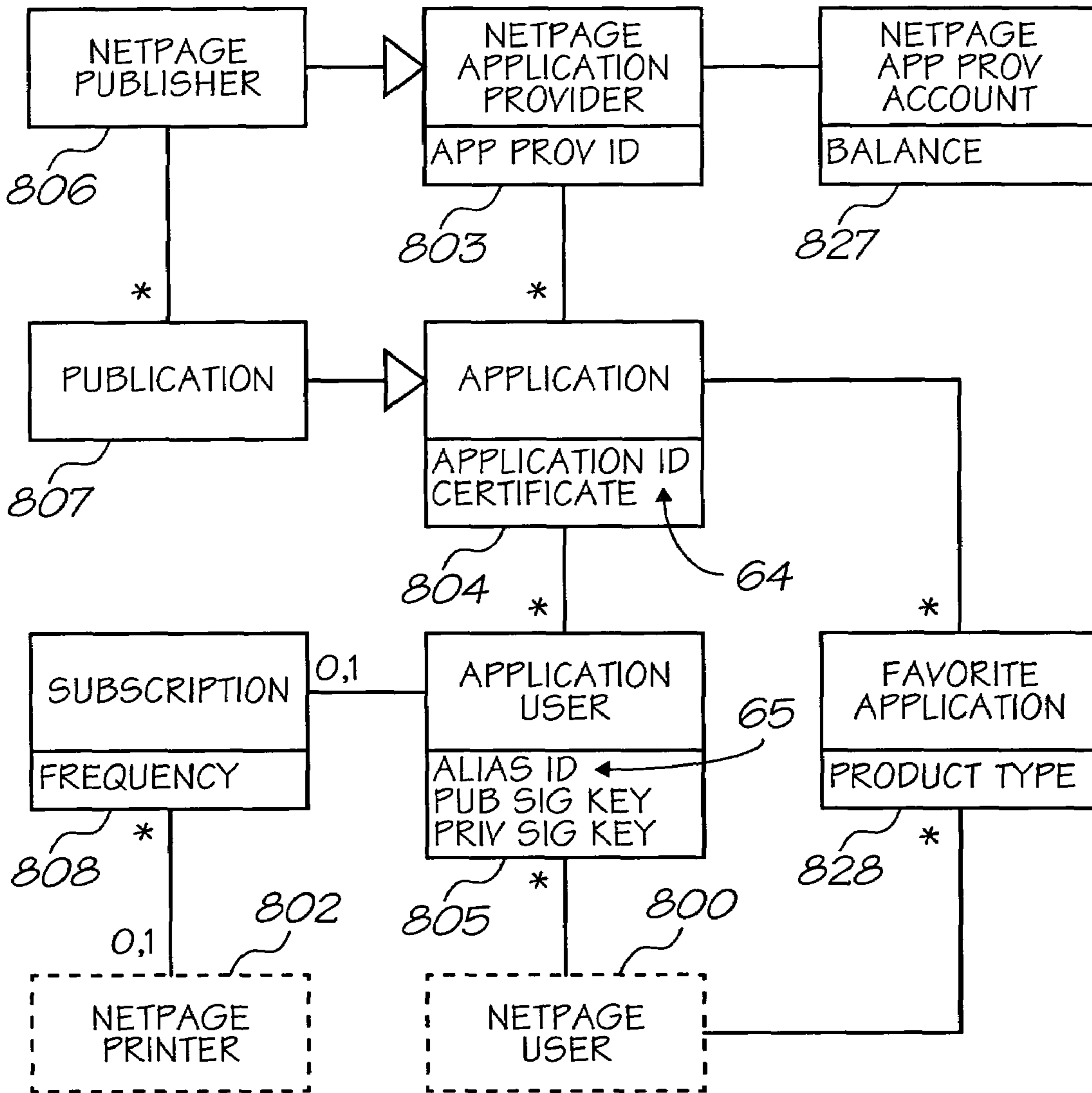
FIG. 24
