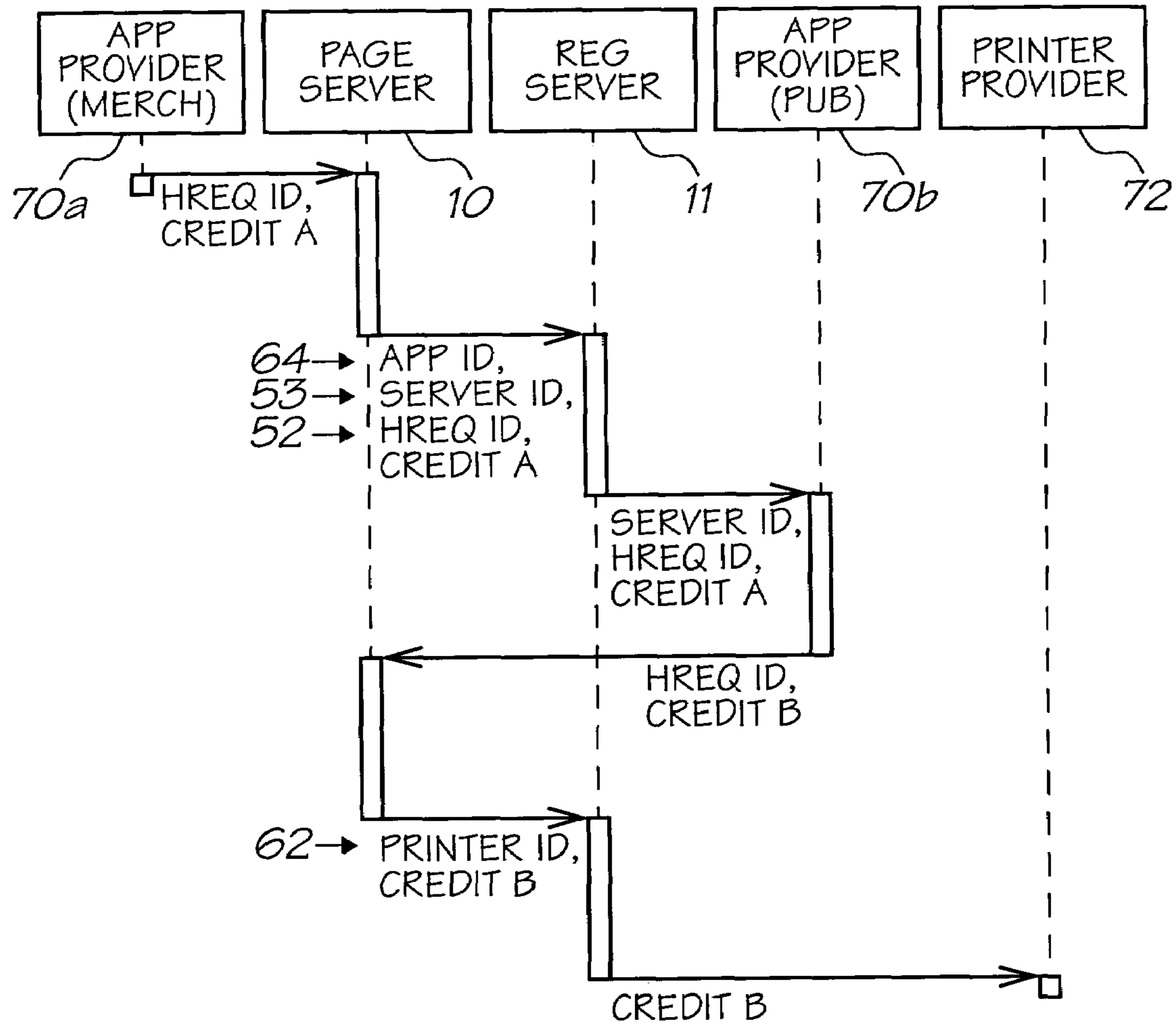
FIG. 47
