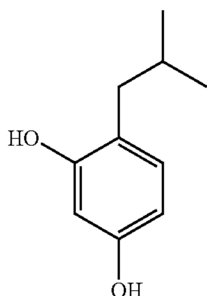
4-Isobutyl-benzene-1,3-diol
