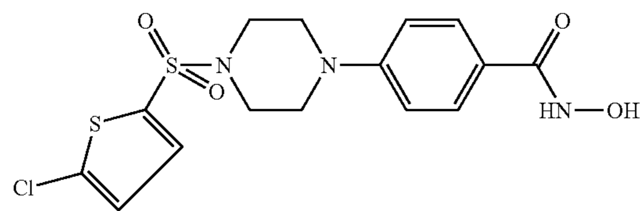
Co. No. 66; Ex. [B1]; mp. 231° C.
