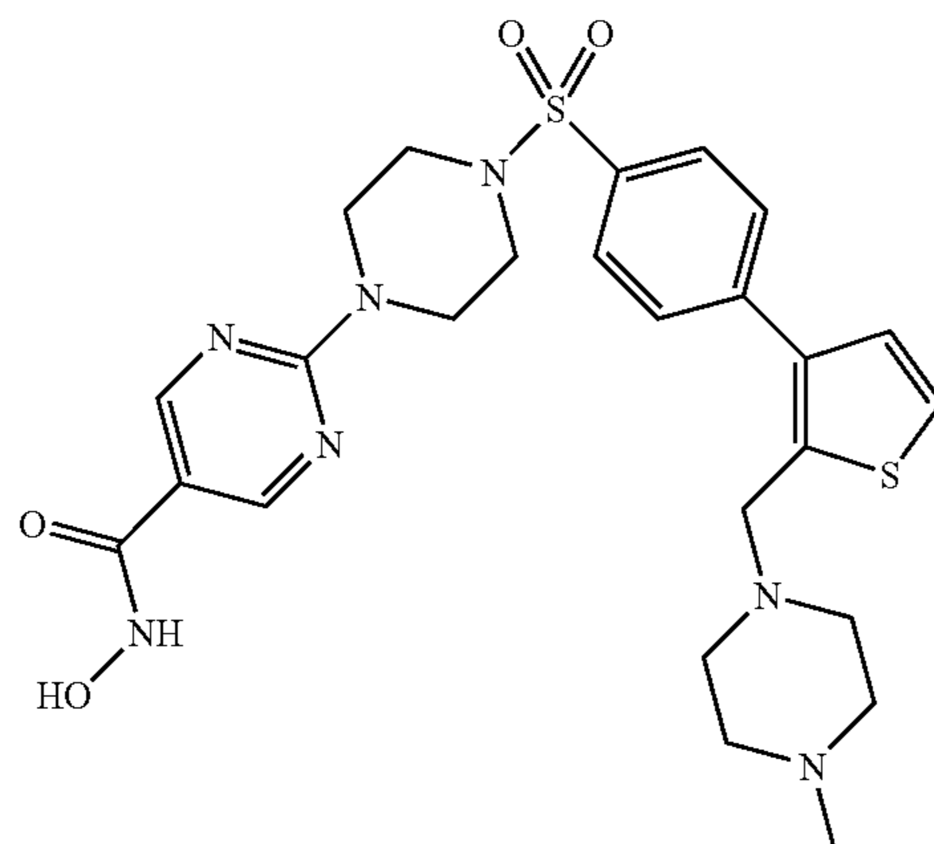
.0.65 \text{ H}_2\text{O} \cdot \text{C}_2\text{HF}_3\text{O}_2 ; Co. No. 144
