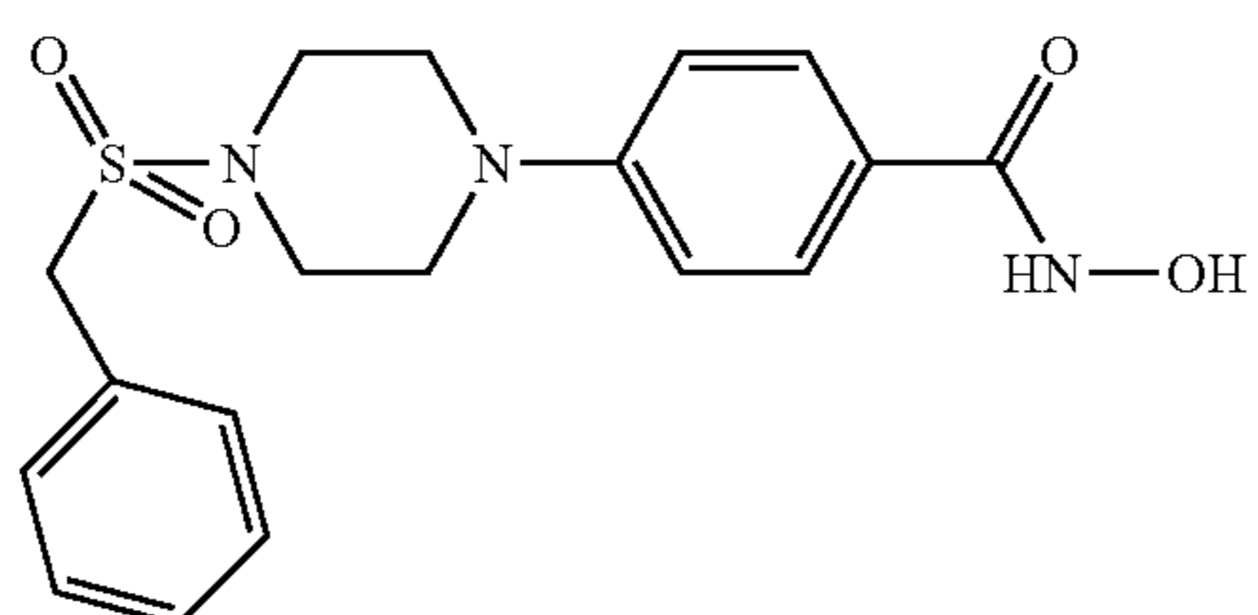
Co. No. 73; Ex. [B1]
