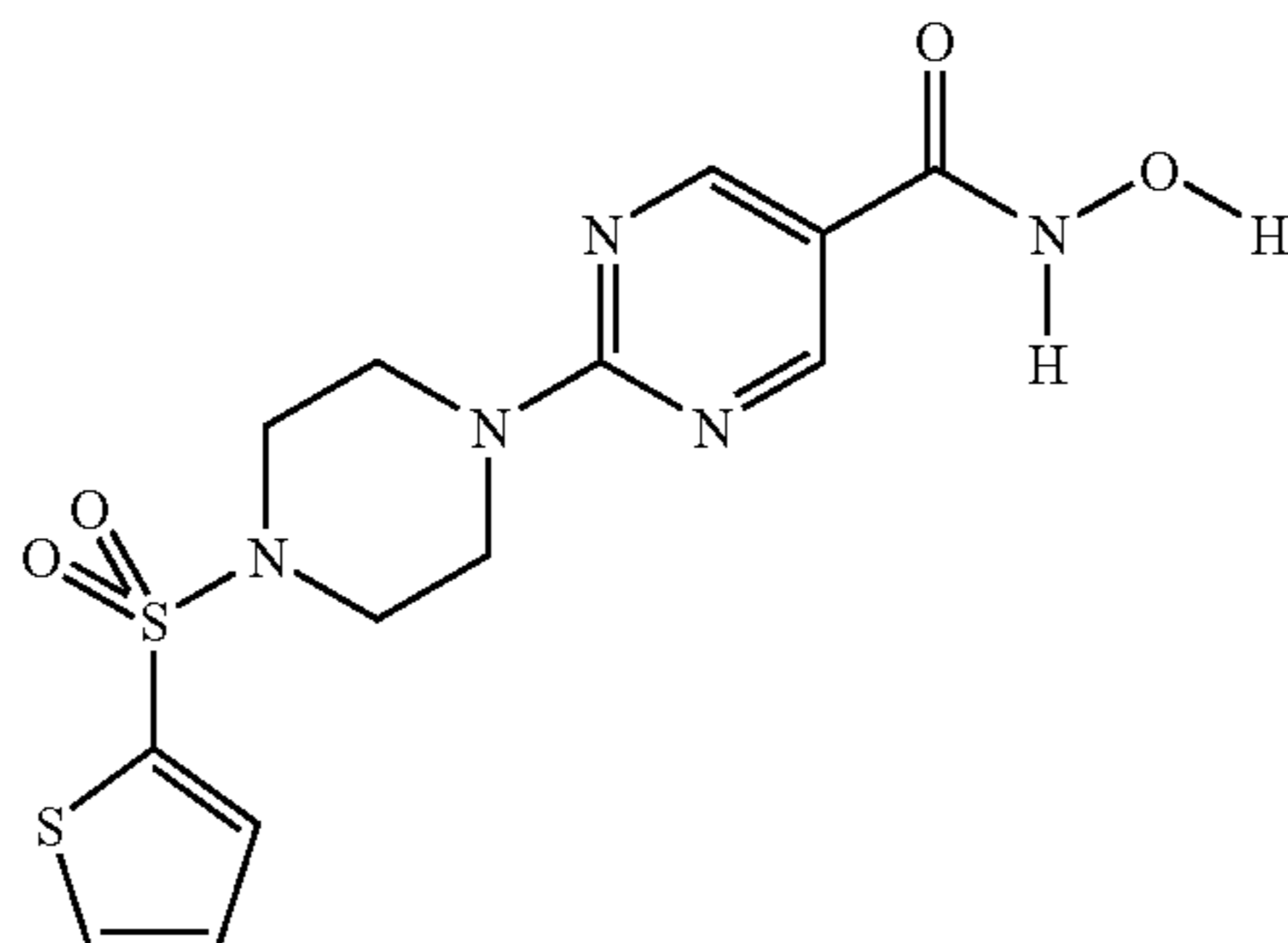
Co. No. 90; Ex. [B15]
