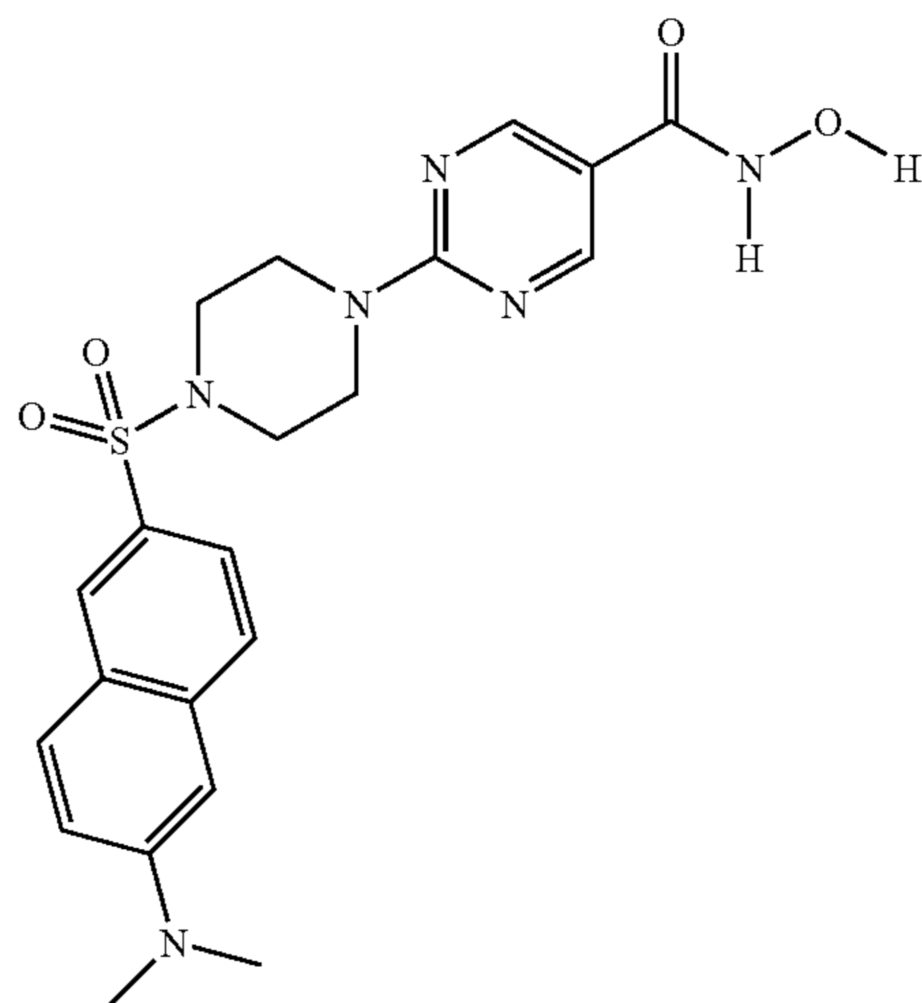
Co. No. 181; Ex. [B32]
