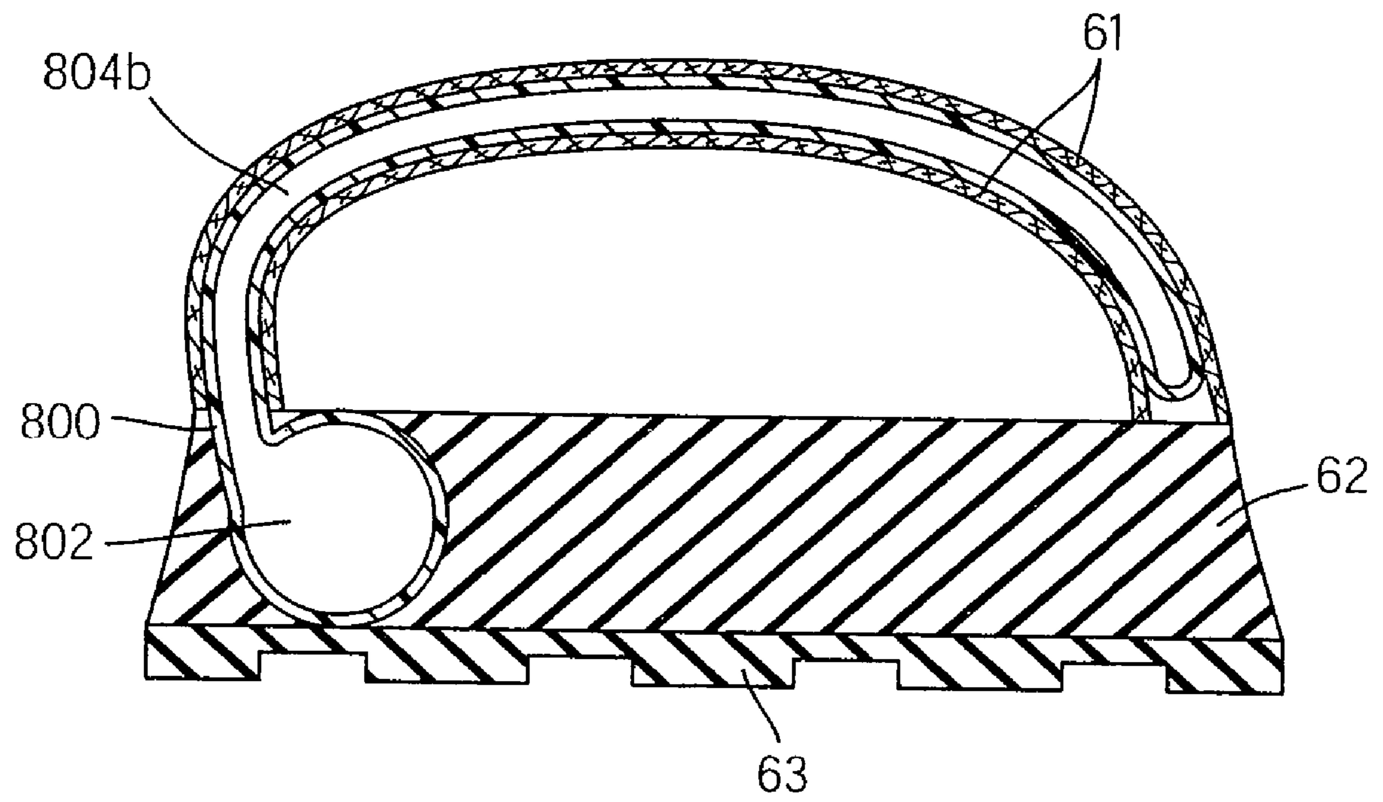
FIG. 24
