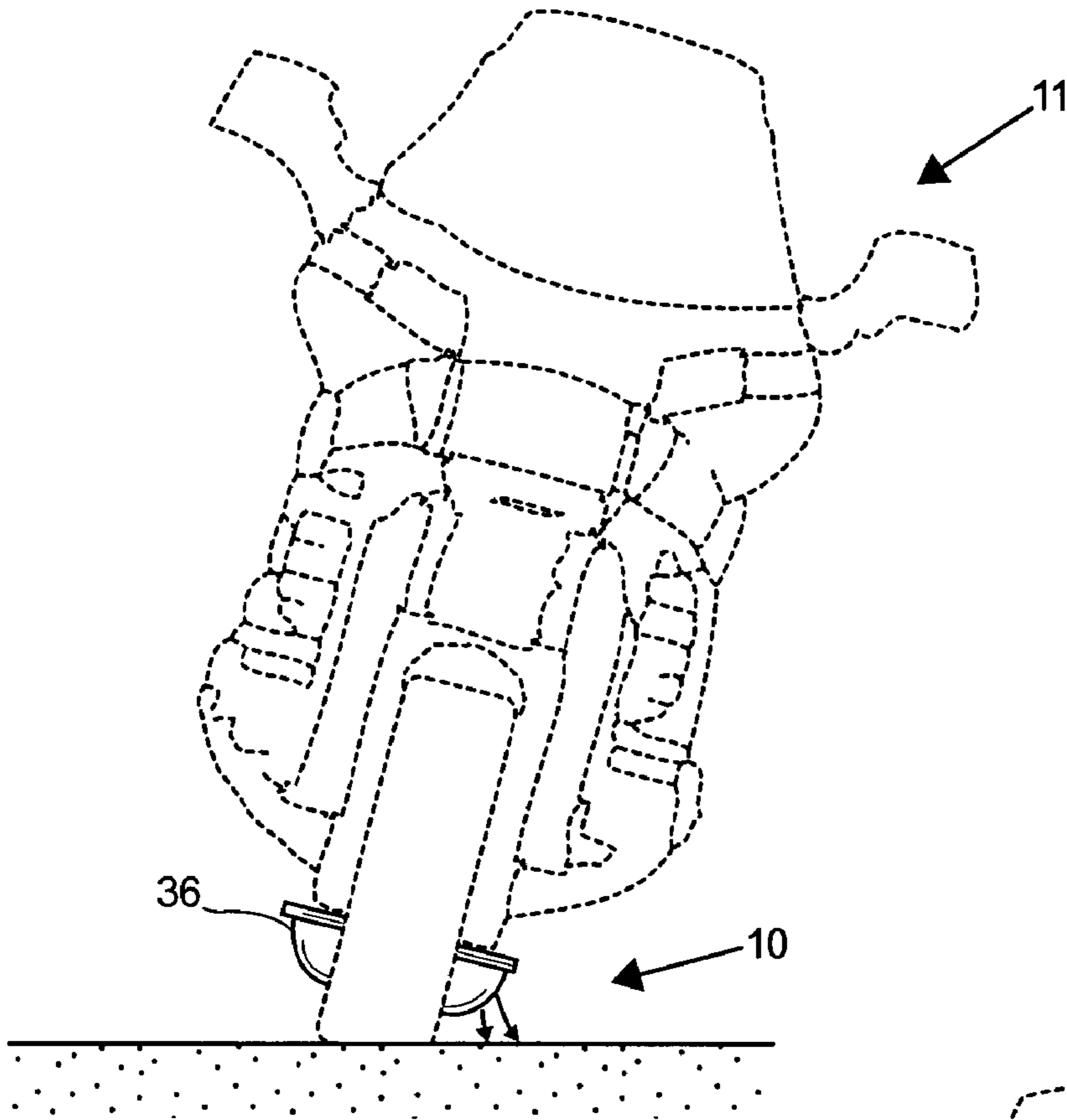
FIG. 6A
