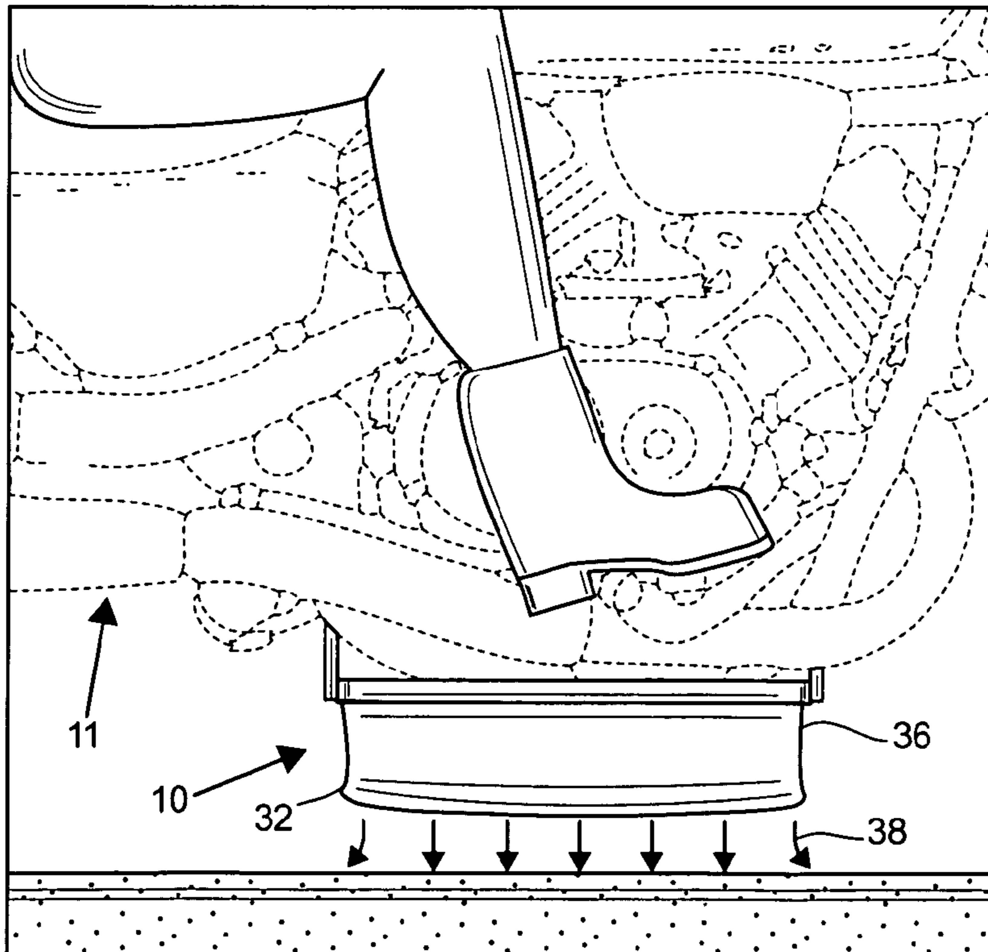
FIG. 5
