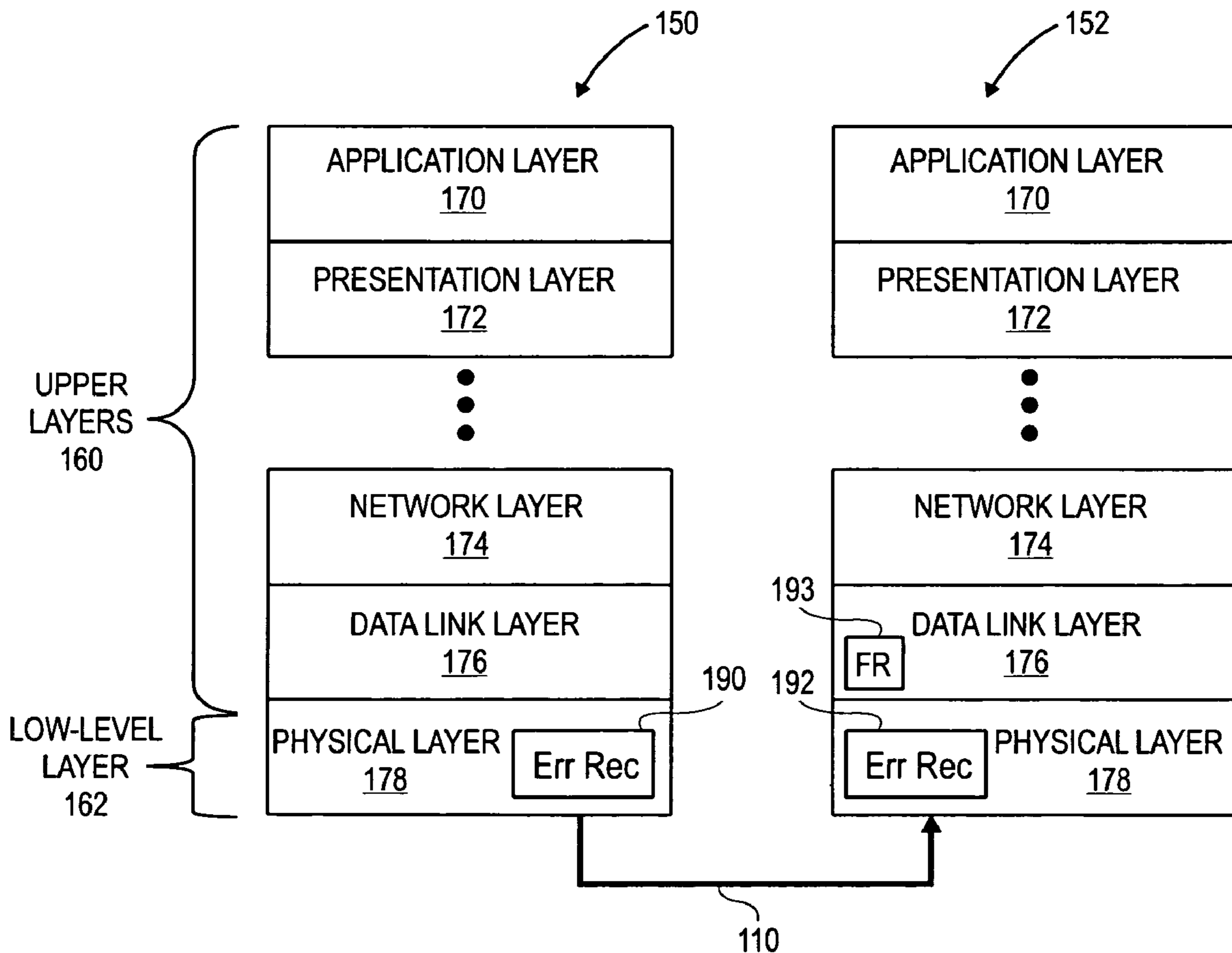
FIG. 1B
