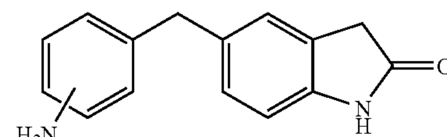
IVa &amp; IVb
