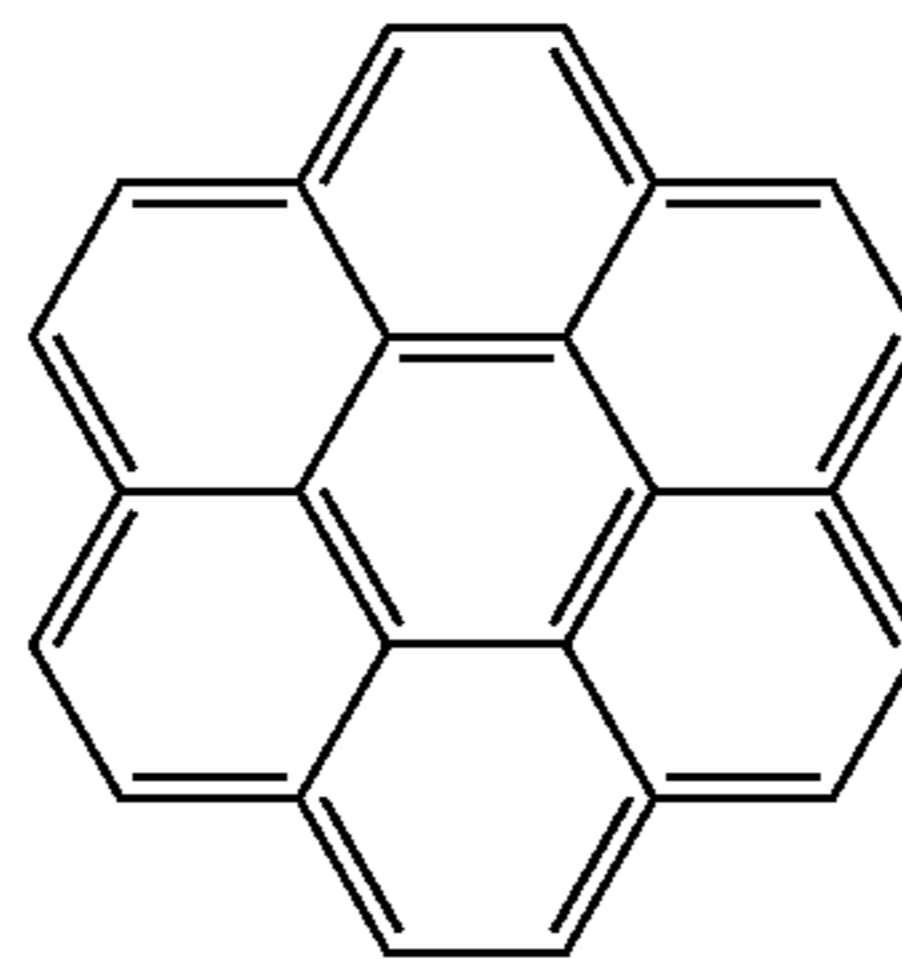
Coronene
