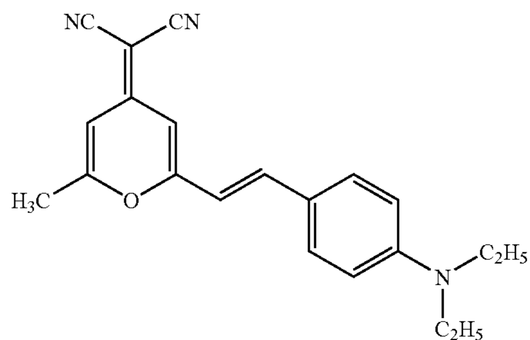
DCM-1
