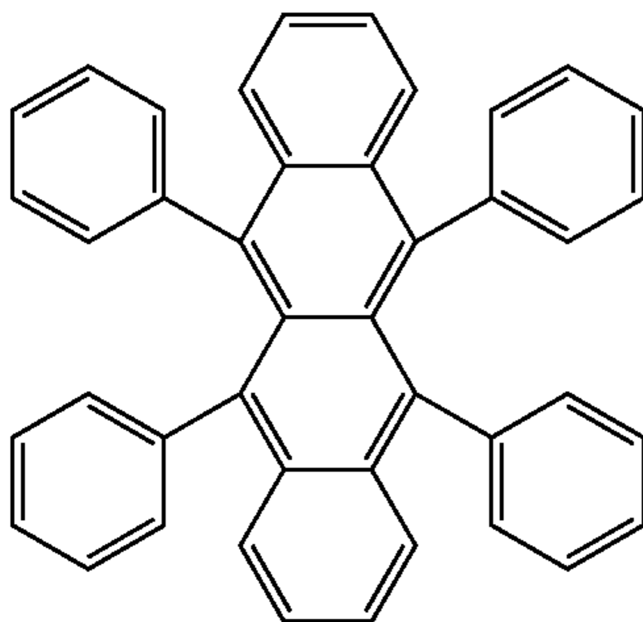
Rubrene
