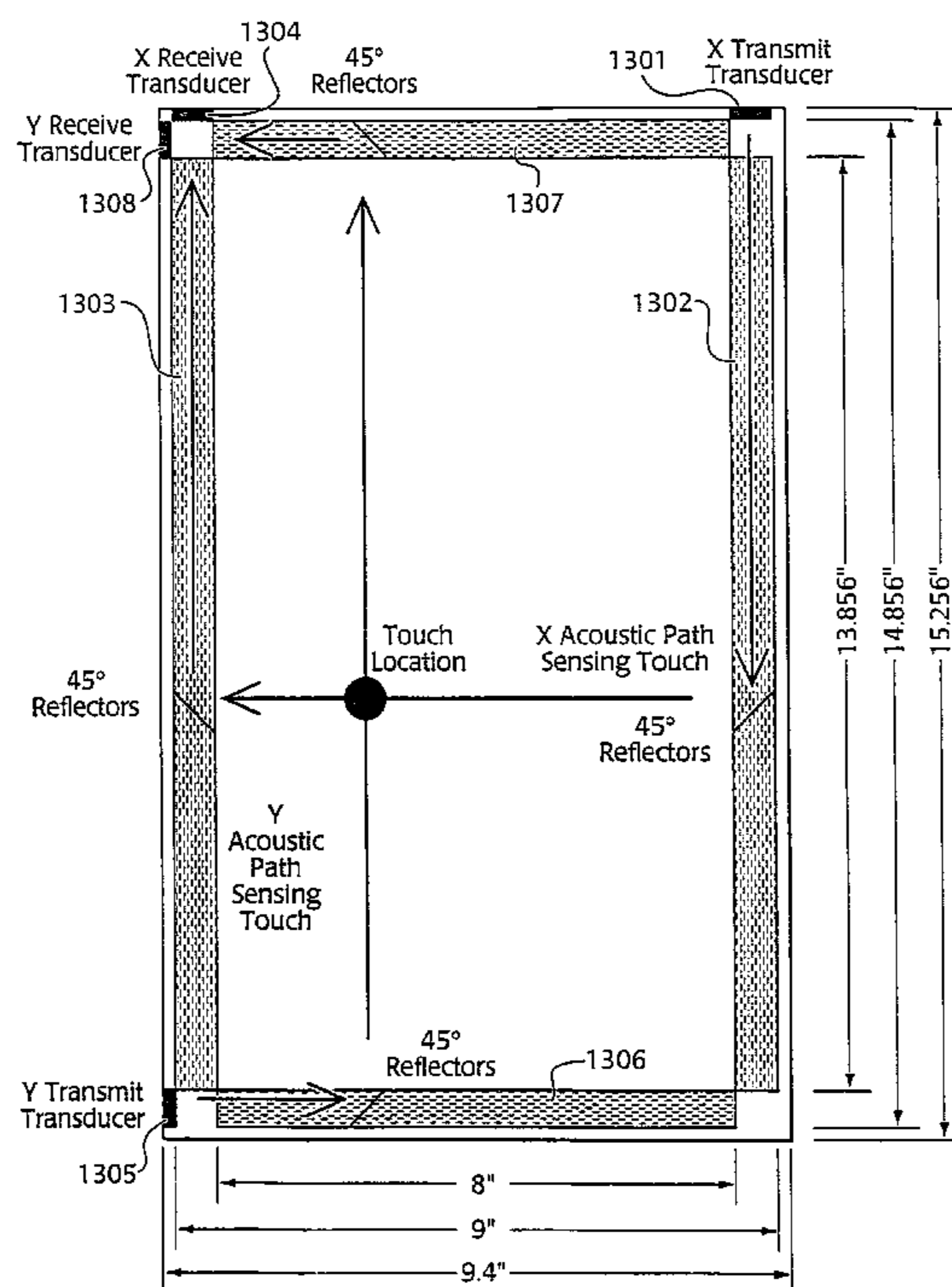
X, Y, 30° Sensor: (a) X & Y Subsystems
