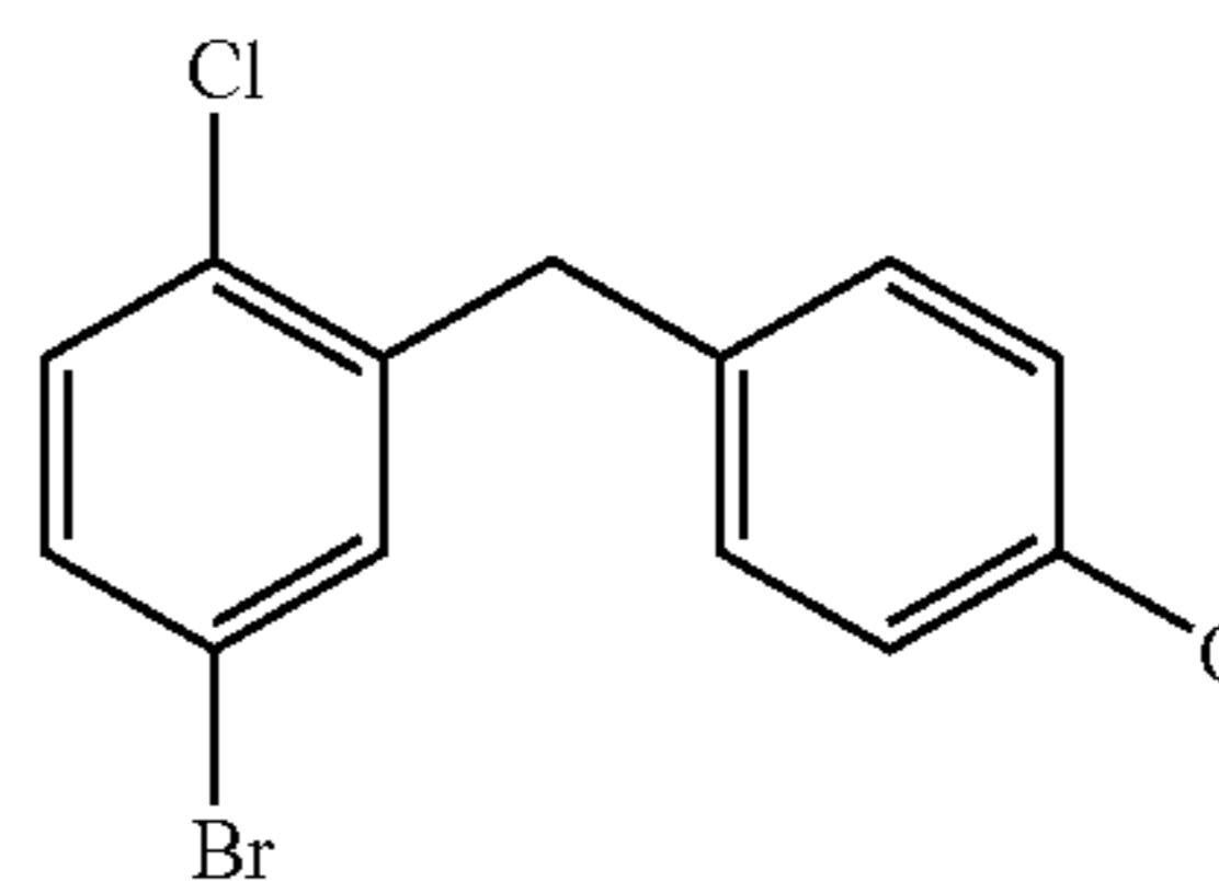
4-Bromo-1-chloro-2-(4-methoxy-benzyl)-benzene
