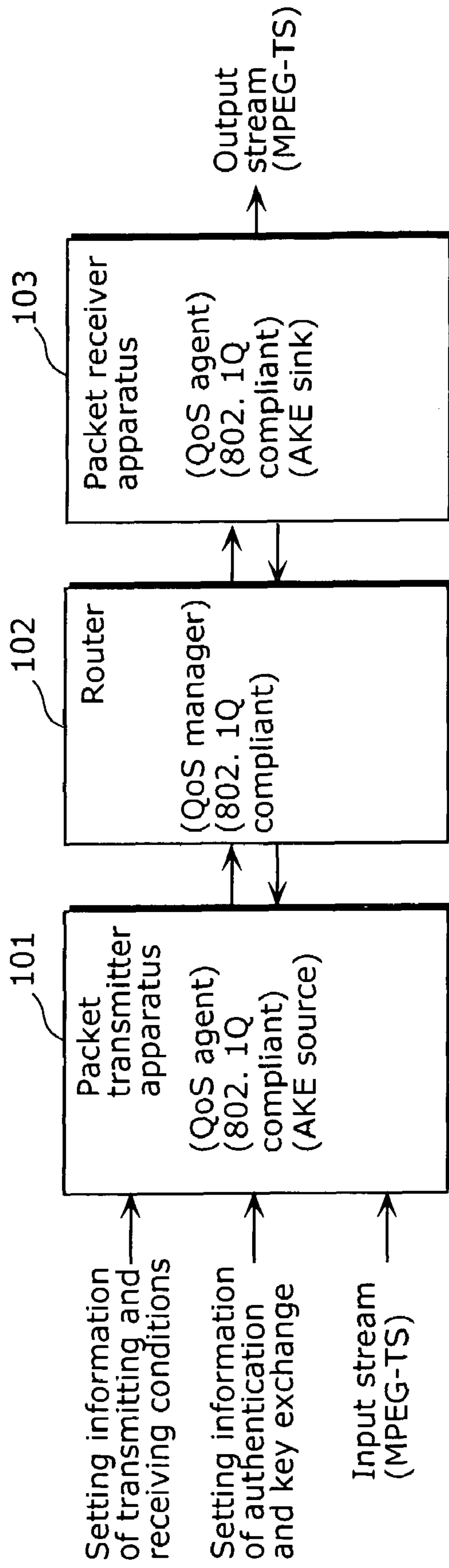
FIG. 5
