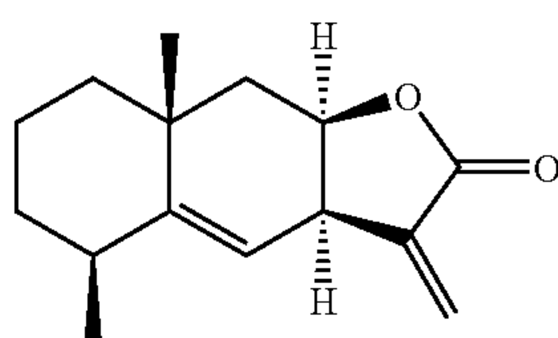
Alantolactone
