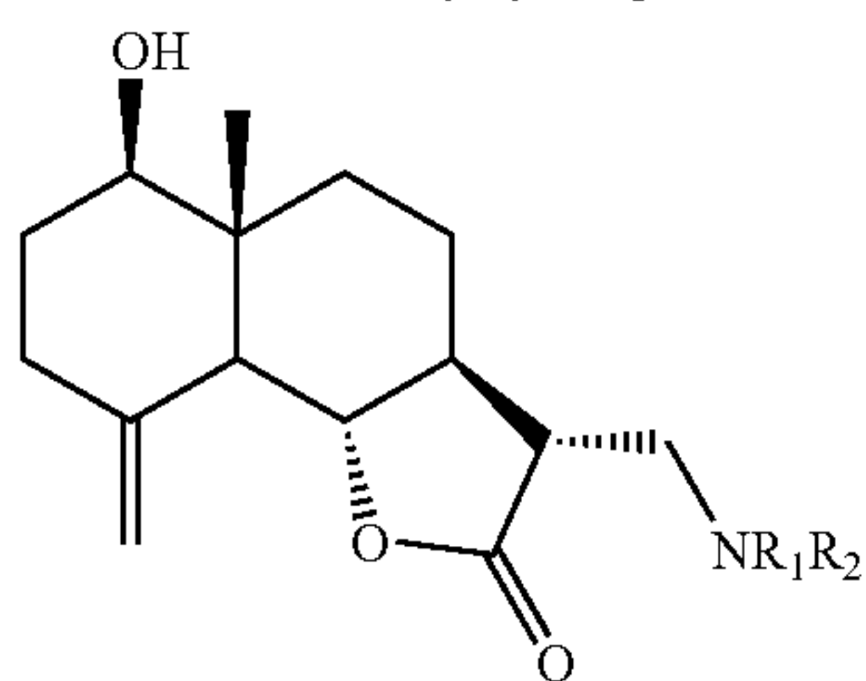
(+) -Aminoreynosins
