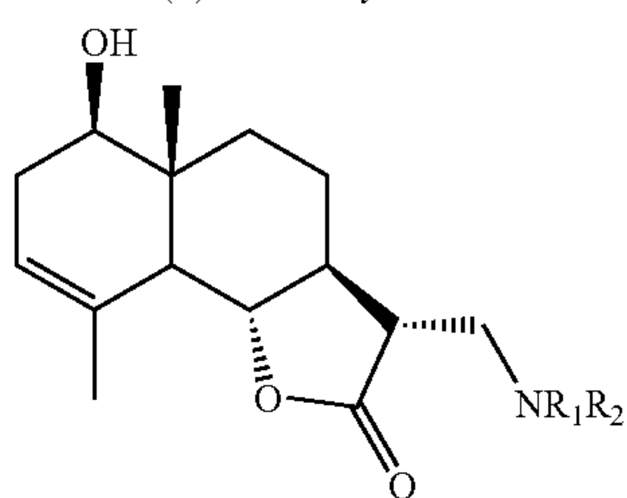
Aminosantamarins
