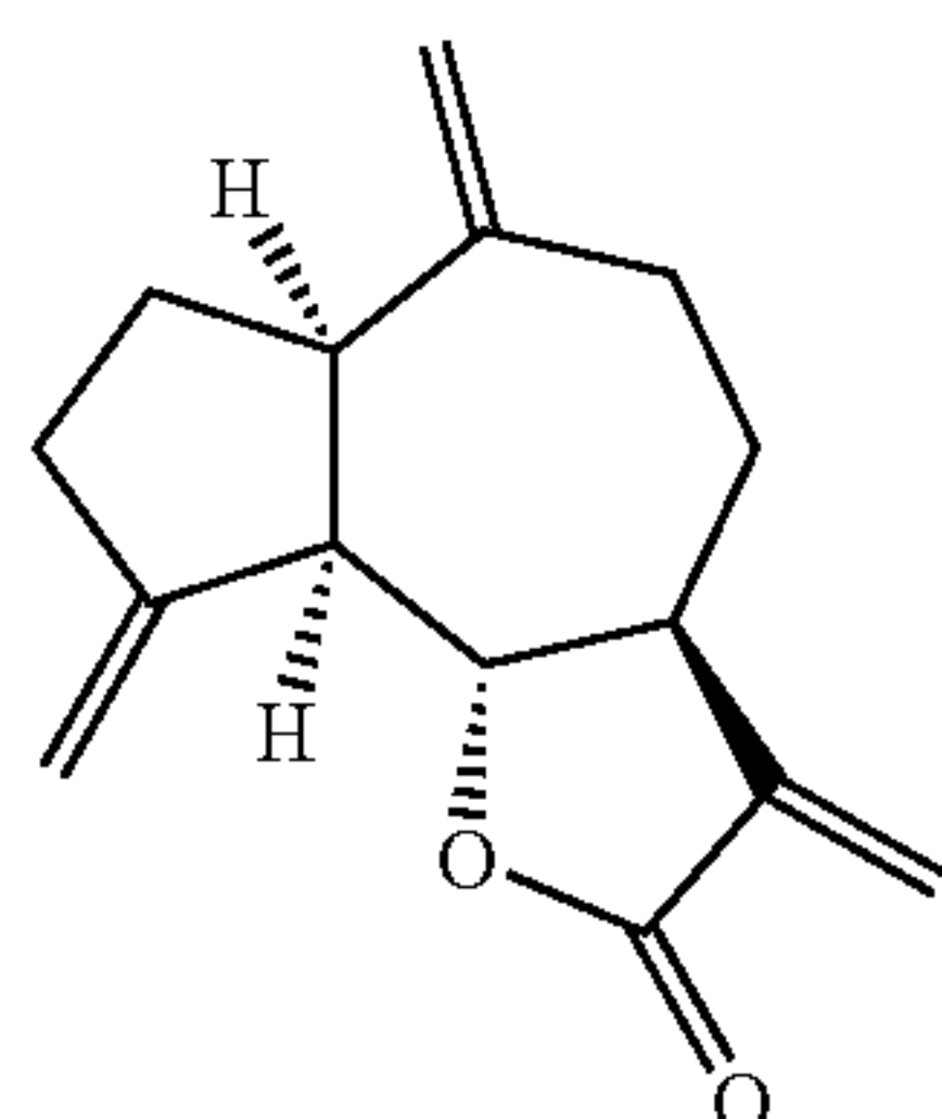
Dehydrocostuslactone
