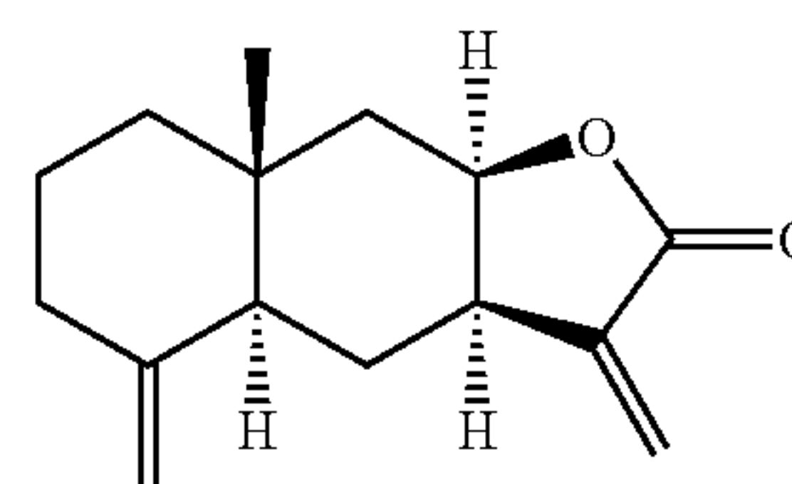
Isoalantolactone
