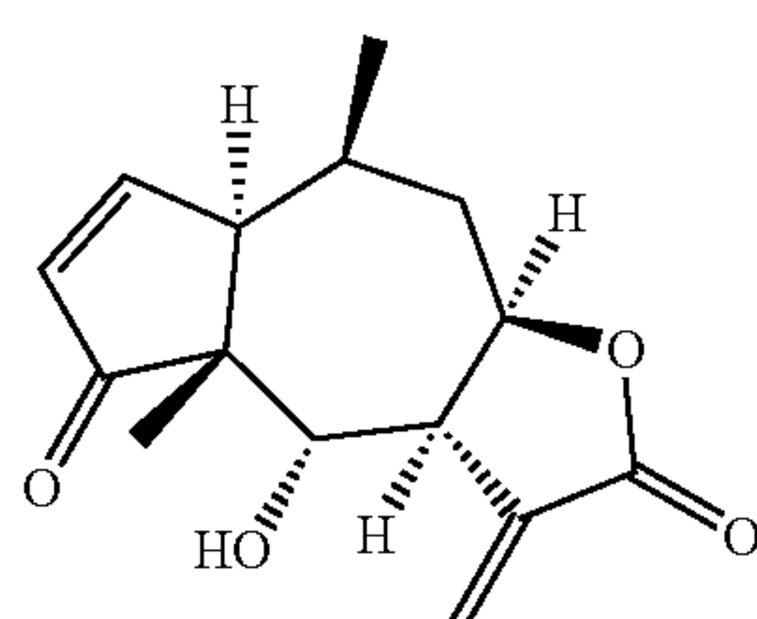
Helenalin
